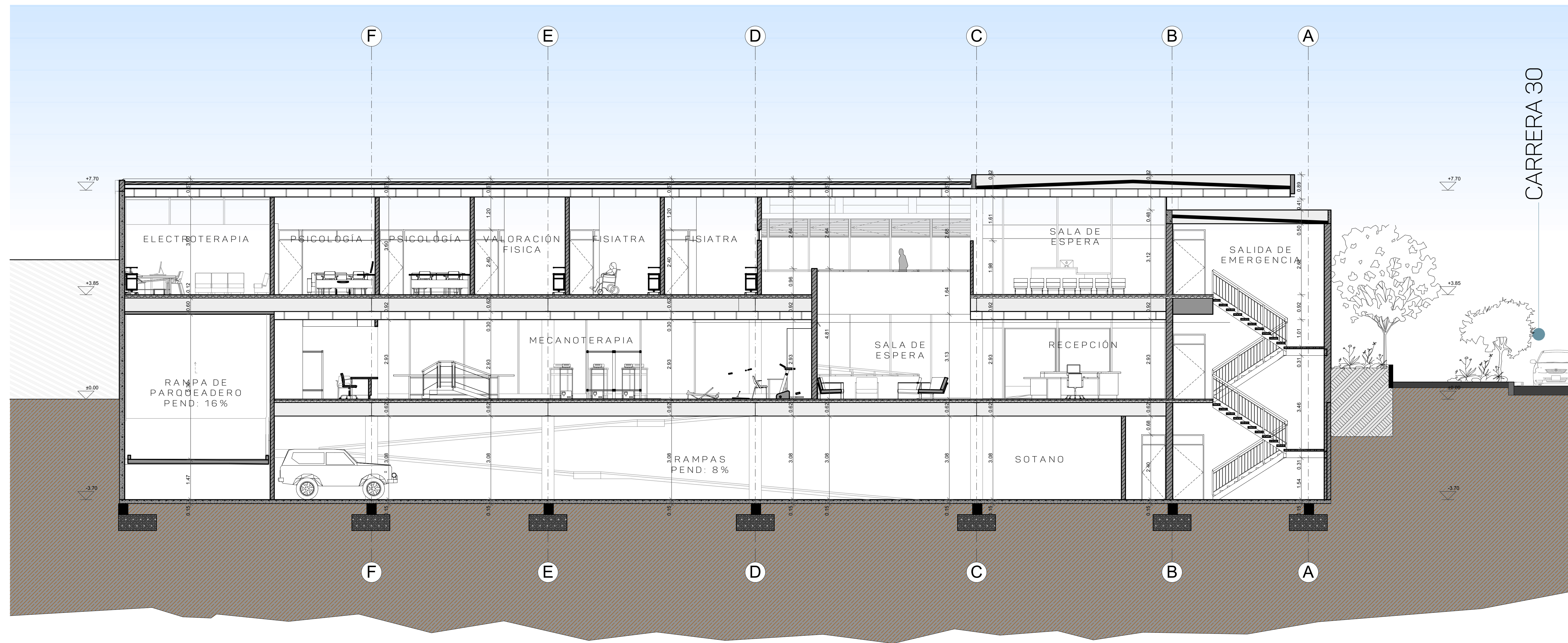
CORTE A-A
