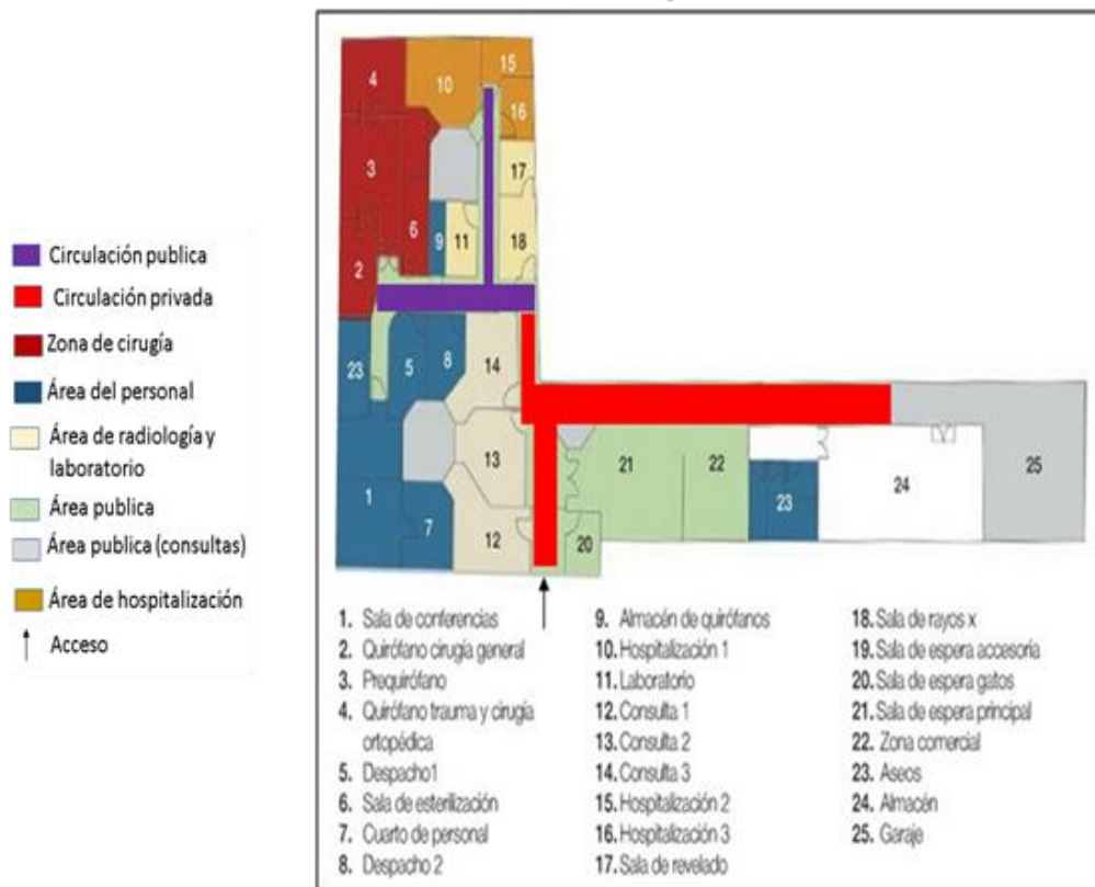
Figura 6. Plano de circulación y zonificación del Centro Veterinario Fauna - Imagen Editada (creación propia)
