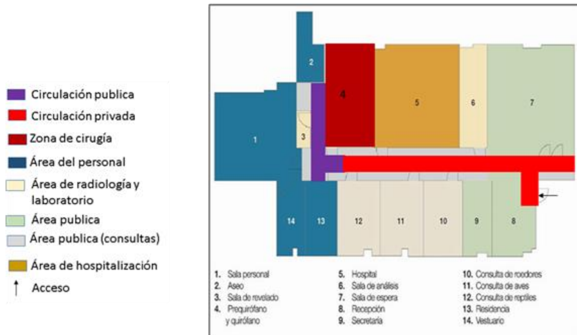
Figura 12. Plano de circulación y zonificación de la Clínica veterinaria exóticas - Imagen Editada (creación propia)
