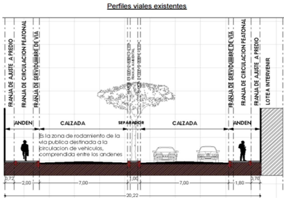
Perfil vial existente AV. LA ROSITA Esc 1:100
