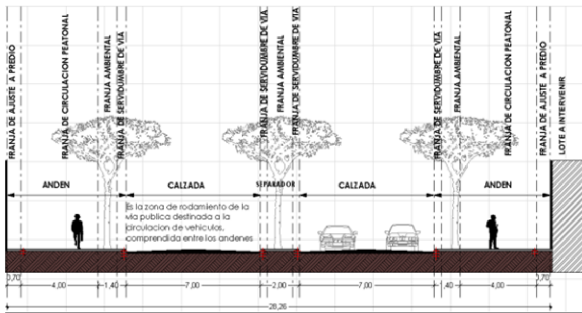
Propuesta de perfil vial AV. LA ROSITA
