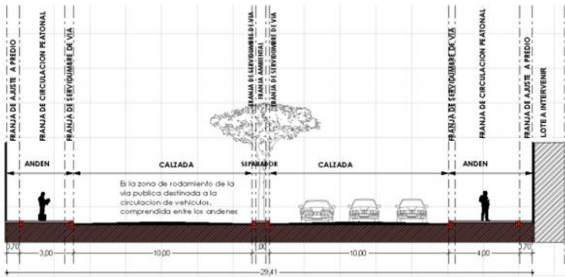
Perfil vial existente CR. 27
