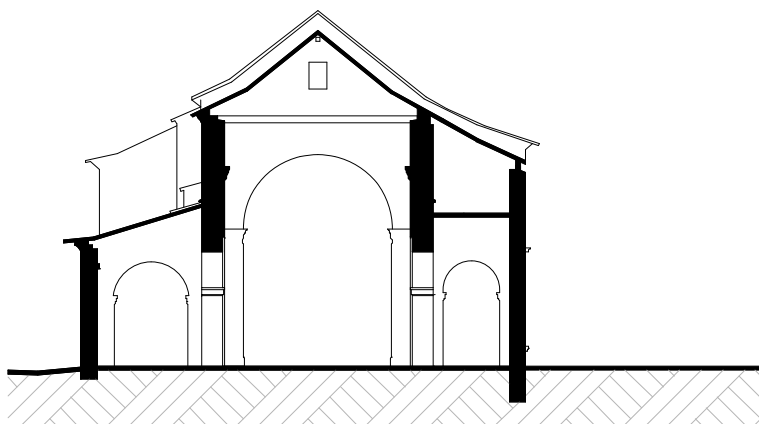
Figura 32. Corte transversal por el templo.
