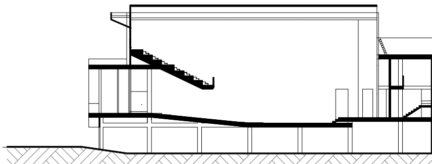
Figura 147. Corte longitudinal por el templo Adventista Redención, Bucaramanga.
