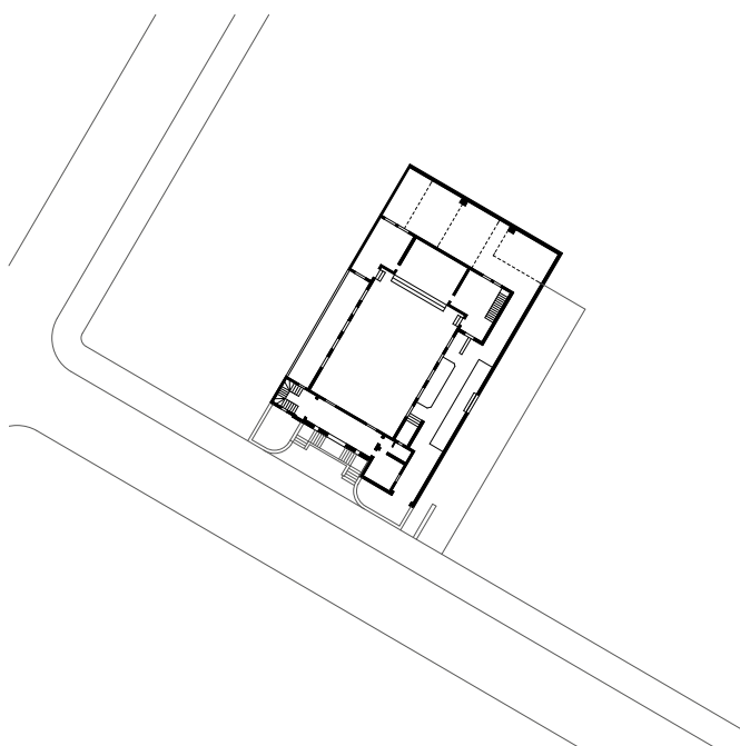
Figura 66. Planta arquitectónica de la primera iglesia presbiteriana. Fuente: Dibujo de Oscar Millán García.
