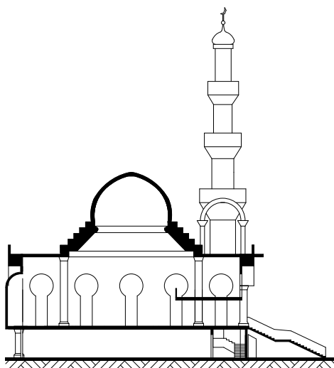
Figura 111. Fachada principal de la mezquita de Maicao y corte transversal en la mezquita de Maicao.
