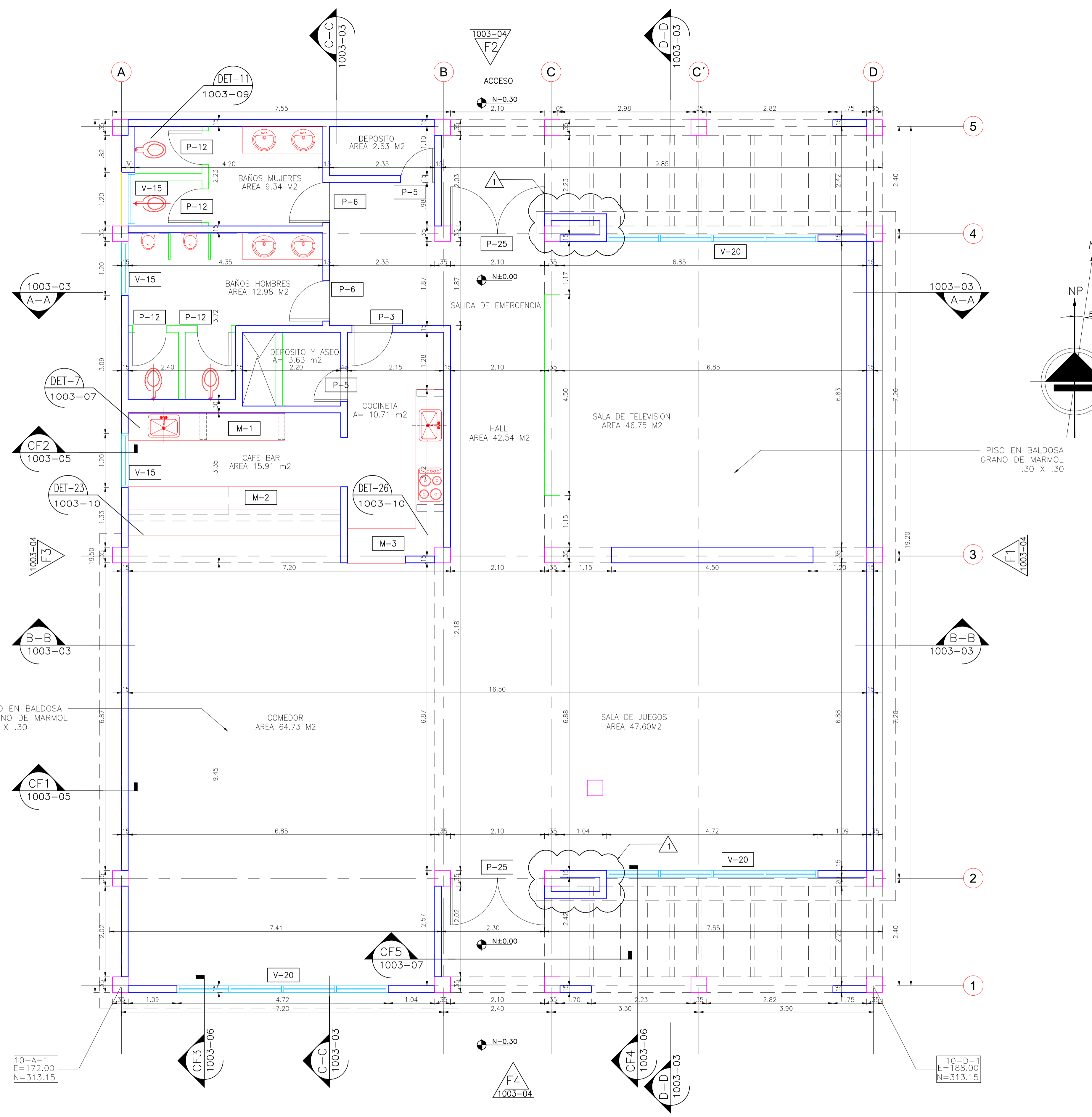
1 PLANTA ARQUITECTONICA ESCALA 1:50
