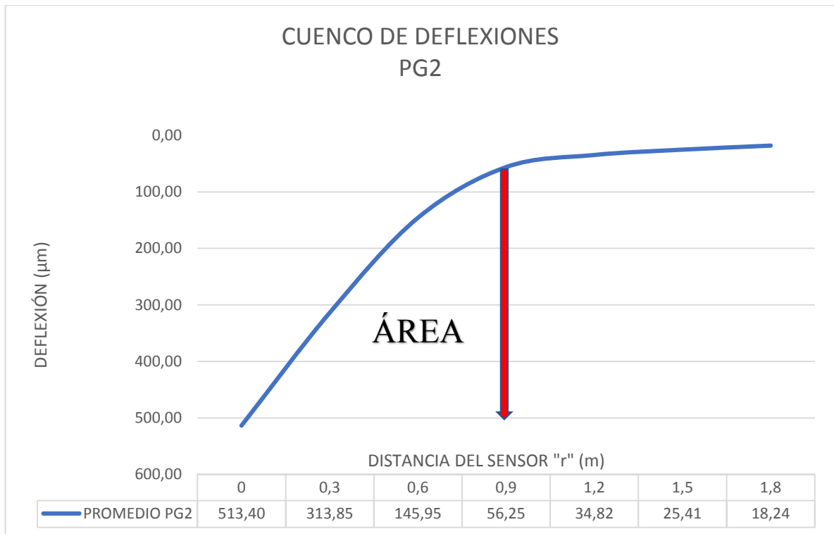
Imagen 1. Cuenco de deflexiones y ubicación del parámetro AREA PG2
