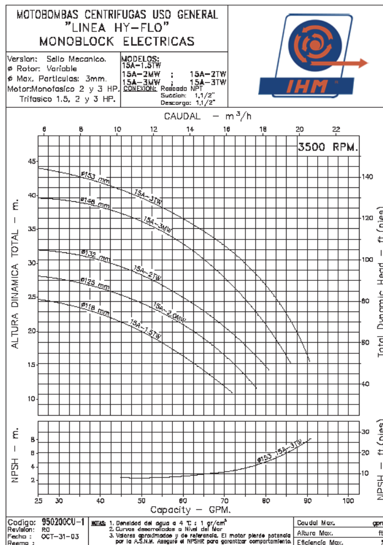
Figura 1 Curva característica de la bomba tipo caracol referencia: 63986000a2 de 1.5 hp
