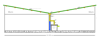
VISTA LATERAL ALTERNATIVA 2
