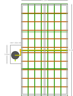
ESTRUCTRA BÁSICA DE LA CUBIERTA VIVIENDA 1 LIMAHOYA
