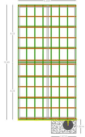
ESTRUCTRA BÁSICA DE LA CUBIERTA VIVIENDA 1 LIMATESA
