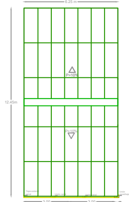
VISTA EN PLANTA DE LA CUBIERTA VIVIENDA 1 LIMATESA
