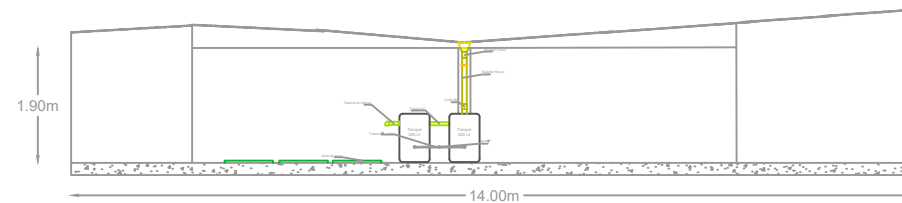
VISTA FACHADA PRINCIPAL VIVIENDA 2
