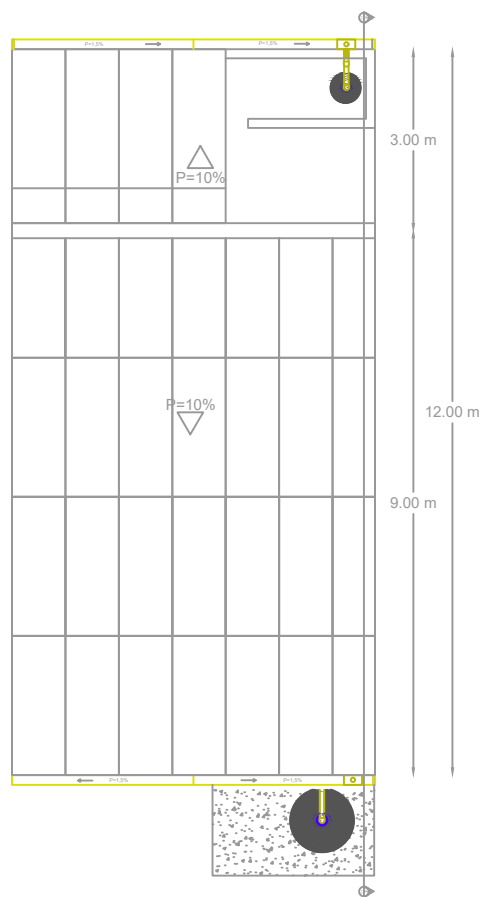
VISTA EN PLANTA DE LA CUBIERTA VIVIENDA 3
