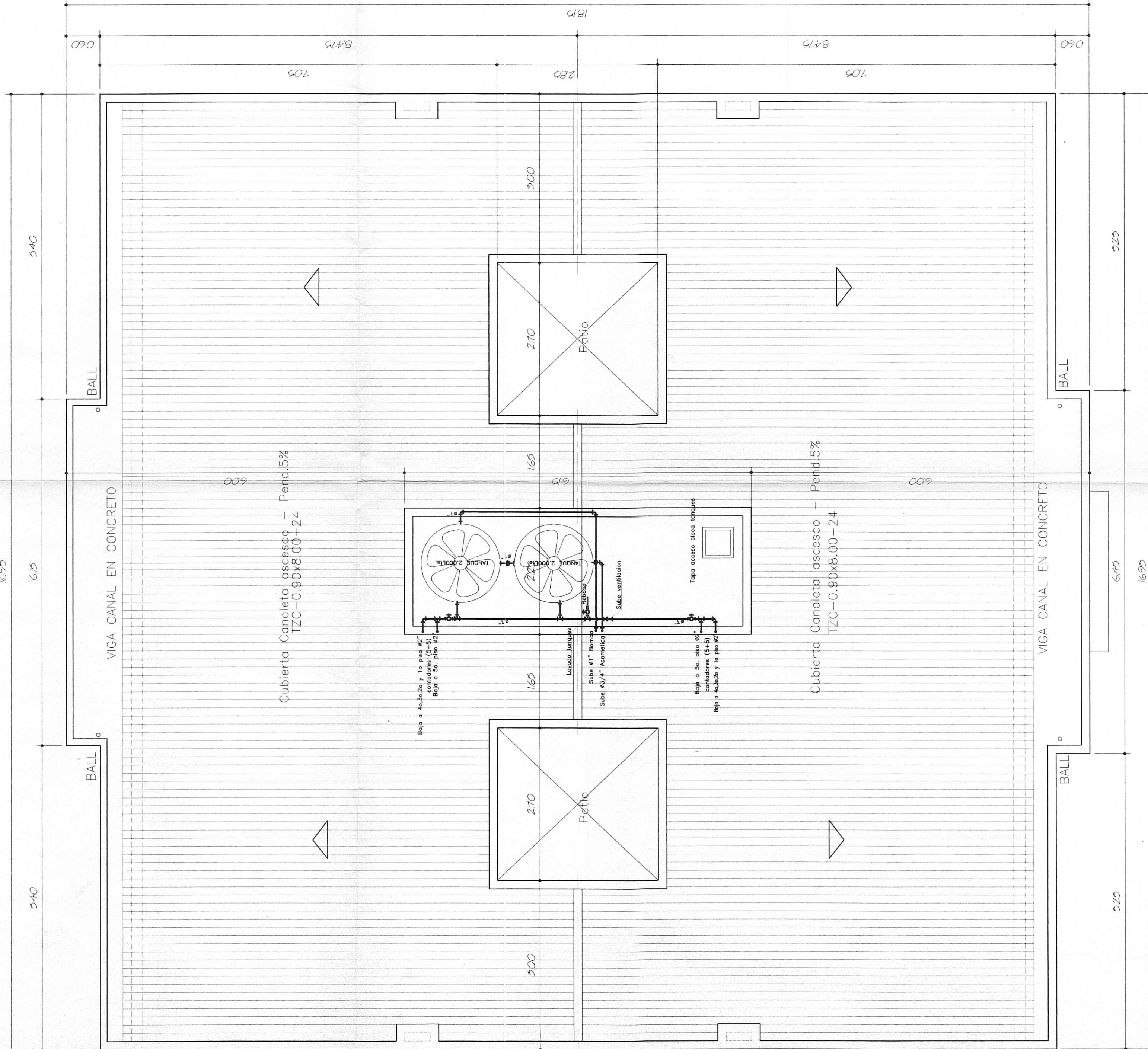
PLANTA CUBIERTA Esc. 1:50
