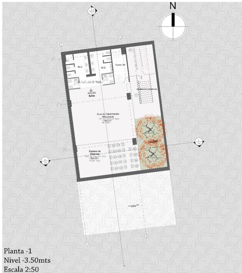
Fig.46. Planta -1 Producción Propia. 2018
