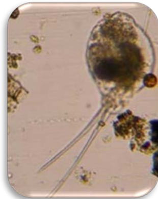
Monommatasp.
