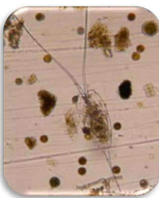
Filiniasp.
