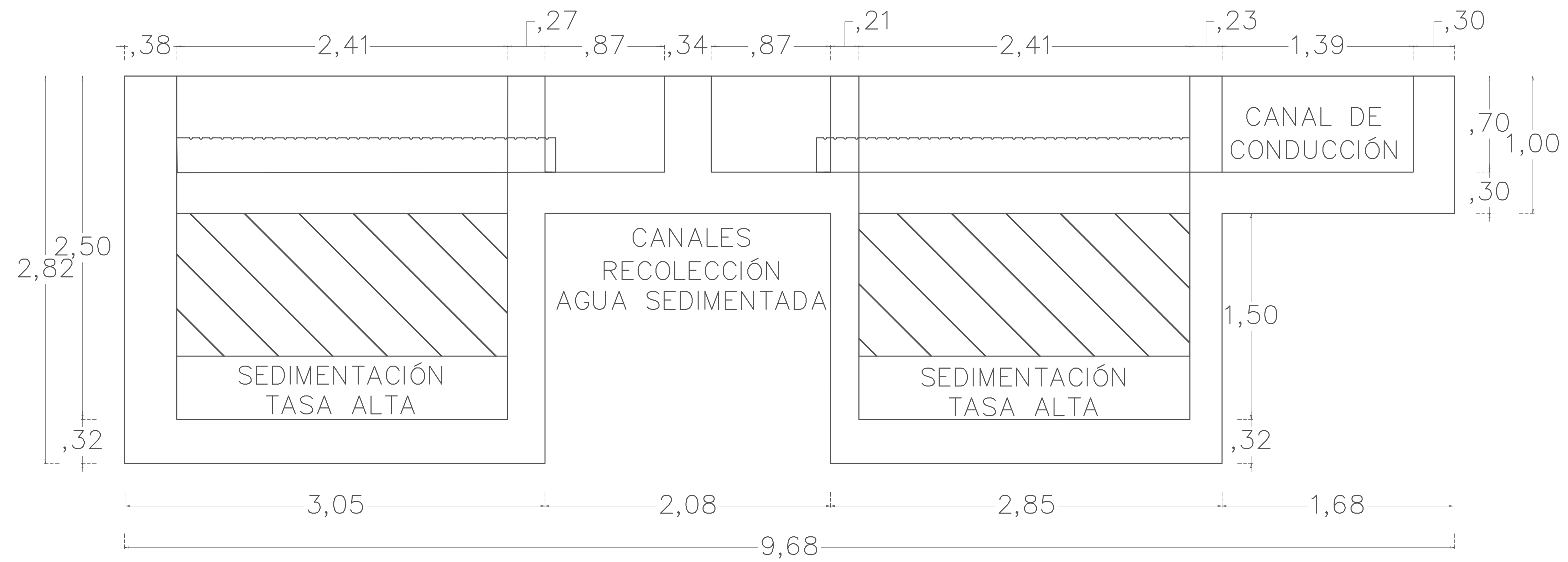
PERFIL TRANSVERSAL SEDIMENTACIÓN CORTE B-B
