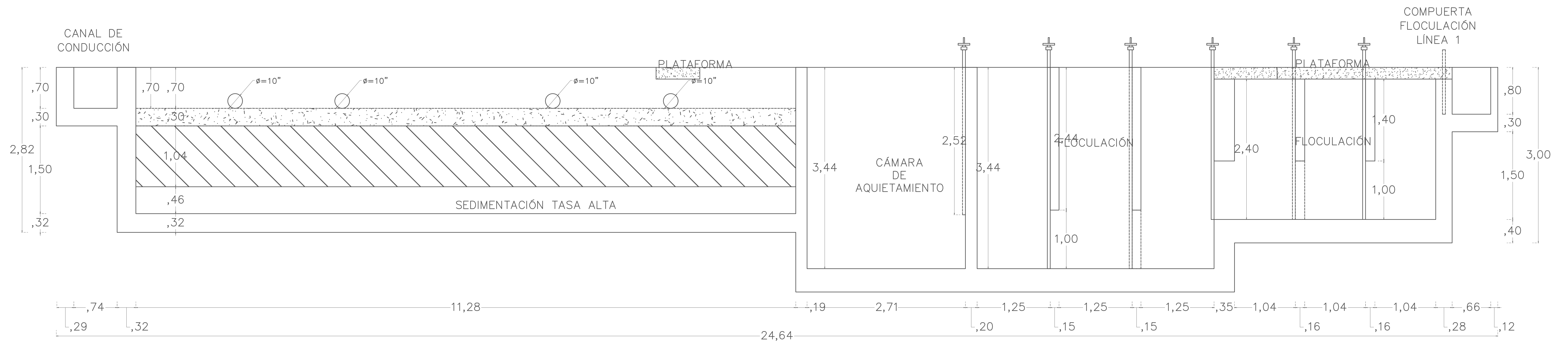
PERFIL LONGITUDINAL FLOCULACION Y SEDIMENTACIÓN CORTE A-A
