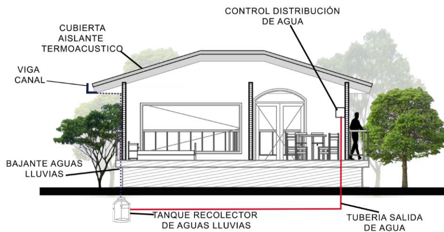
IMAGEN 14 Corte módulo Ecolodge
