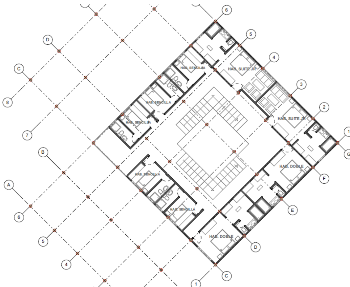
PLANO 8 Habitaciones volúmen administrativo
