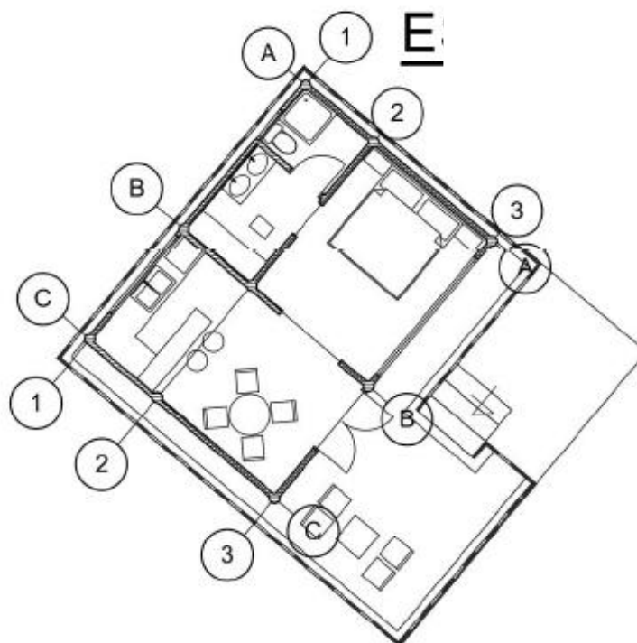
PLANO 22 Planta estructural Modulo glamping Palafito
