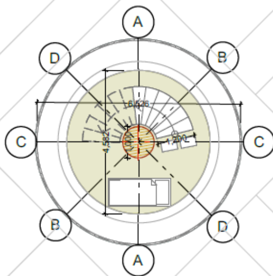
PLANO 7 Módulo glamping Palafito
