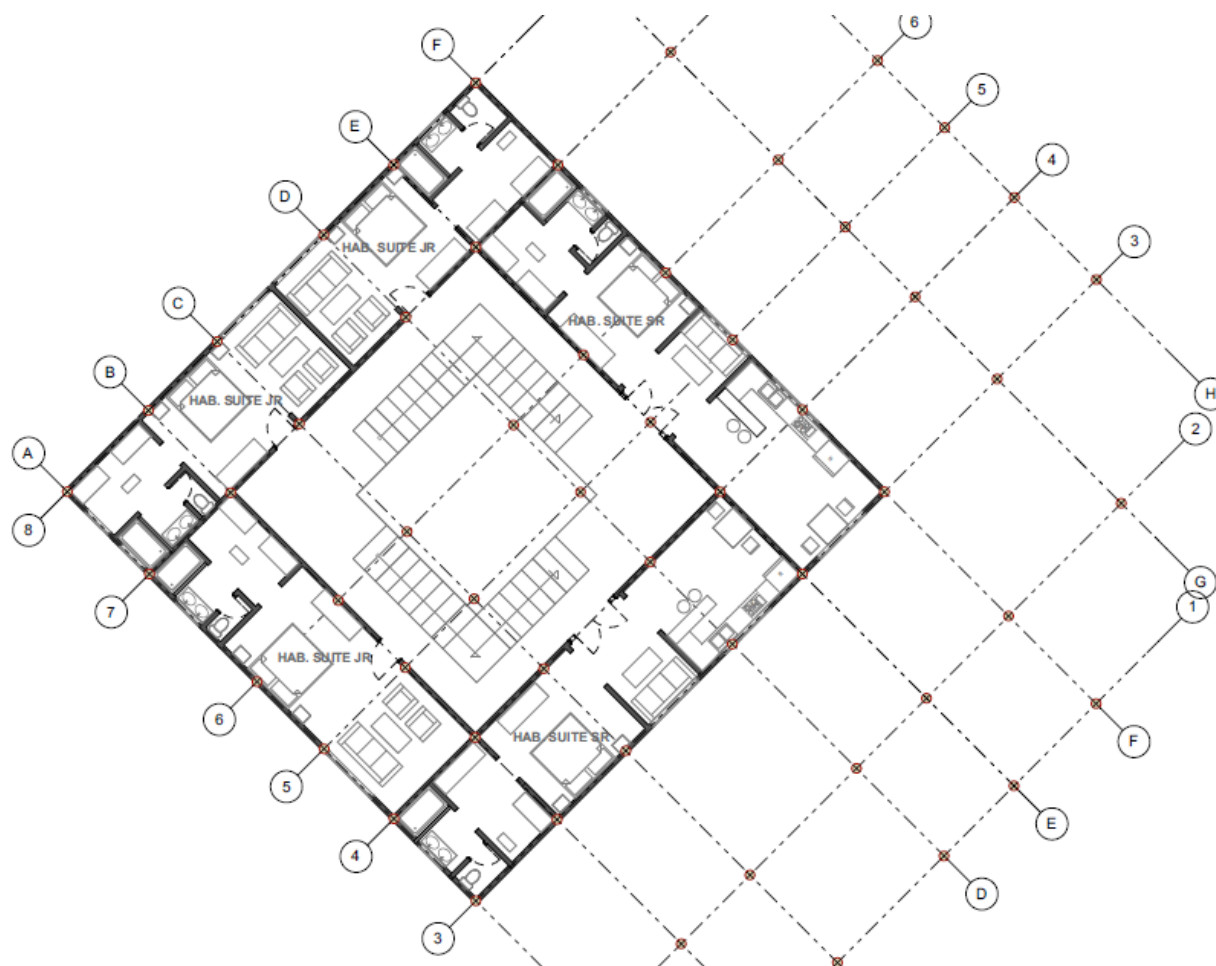
PLANO 9 Habitaciones volumen spa
