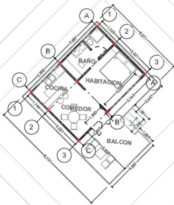
PLANO 6 Módulo glamping Ecolodge
