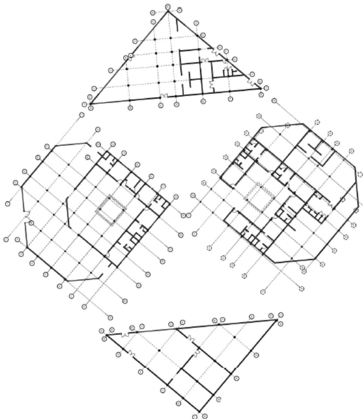
PLANO 20 Planta estructural Hotel Museo
