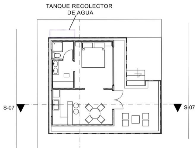
IMAGEN 13 Planta módulo Ecolodge
