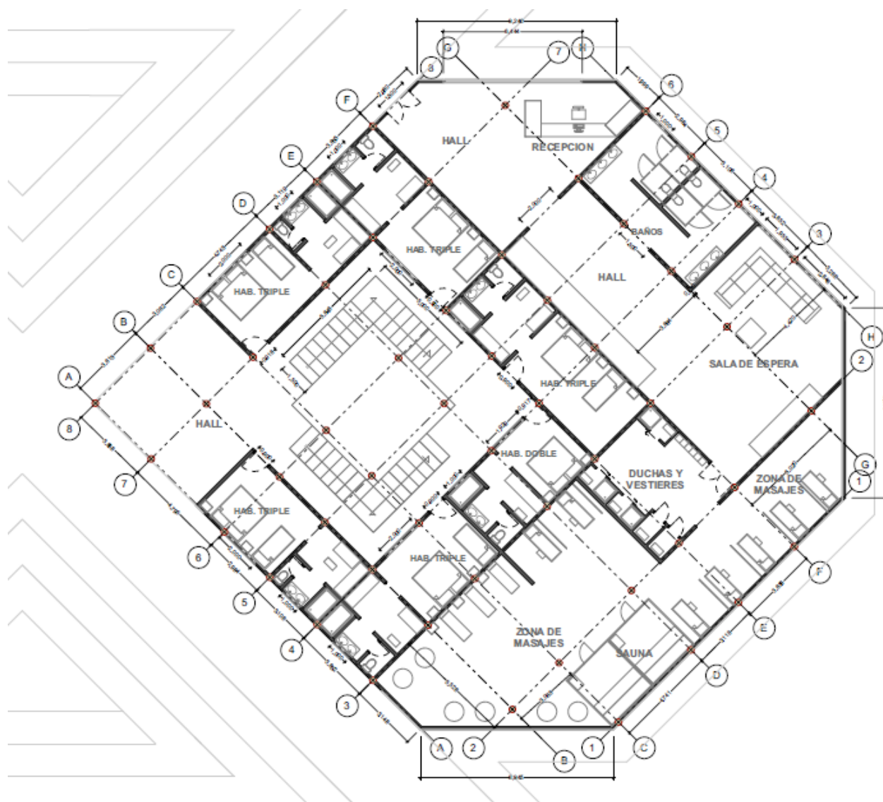
PLANO 5 Zona habitaciones y spa
