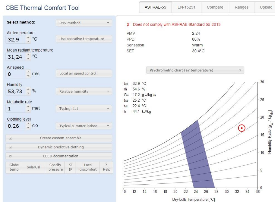
Ilustración 31 Tabulación de datos para hallar el pmv y ppd, (T3-apto301). Elaboración a partir de la herramienta - CBE Thermal Comfort Tool
