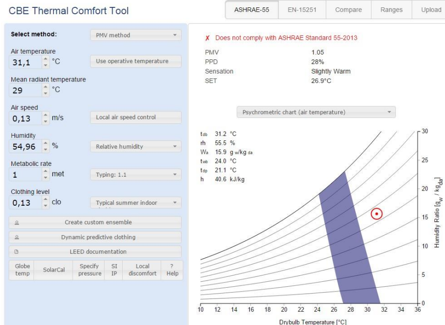
Ilustración 29 Tabulación de datos para hallar el pmv y ppd, (T14-apto404). Elaboración a partir de la herramienta - CBE Thermal Comfort Tool
