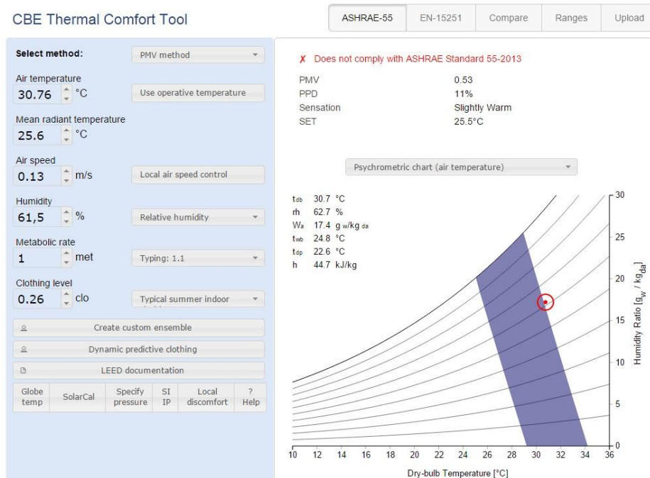
Ilustración 42 Tabulación de datos para hallar el pmv y ppd, (T7-apto203). Elaboración a partir de la herramienta - CBE Thermal Comfort Tool
