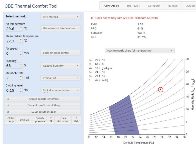
Ilustración 59 Tabulación de datos para hallar el pmv y ppd, (T1-apto206). Elaboración a partir de la herramienta - CBE Thermal Comfort Tool
