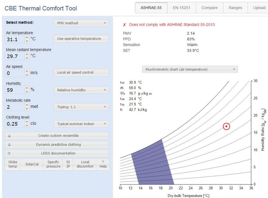
Ilustración 39 Tabulación de datos para hallar el pmv y ppd, (T6-apto406). Elaboración a partir de la herramienta - CBE Thermal Comfort Tool
