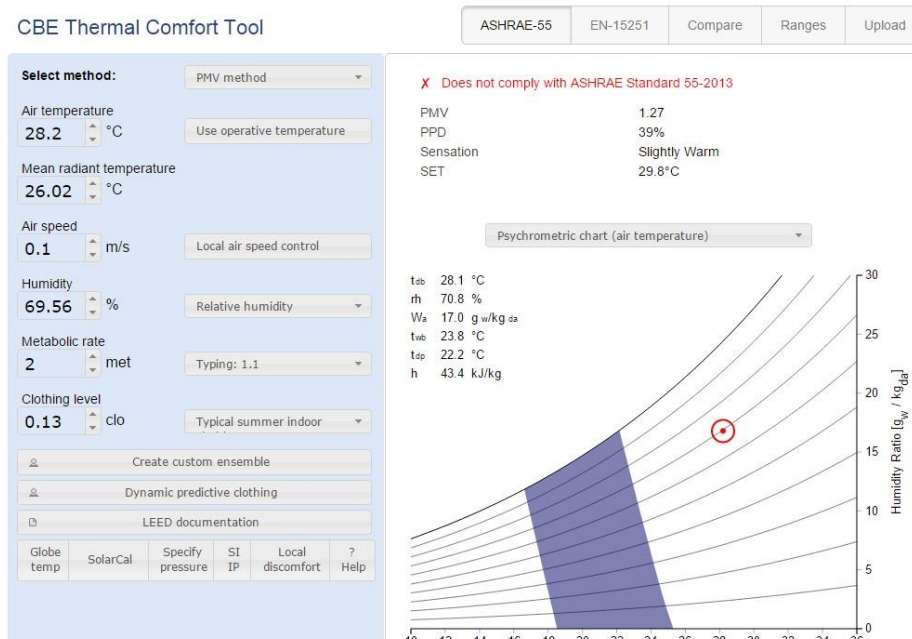
Ilustración 48 Tabulación de datos para hallar el pmv y ppd, (T7-apto403). Elaboración a partir de la herramienta - CBE Thermal Comfort Tool
