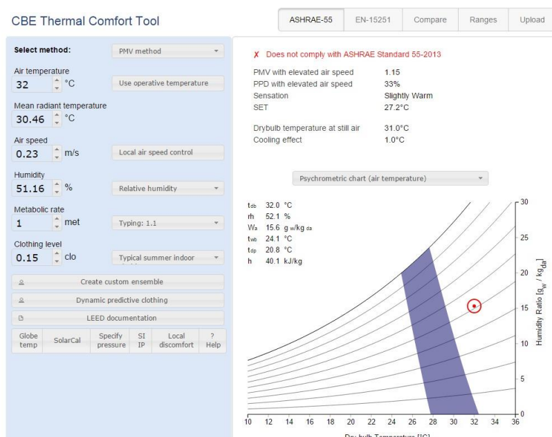
Ilustración 50 Tabulación de datos para hallar el pmv y ppd, (T8-apto202). Elaboración a partir de la herramienta - CBE Thermal Comfort Tool
