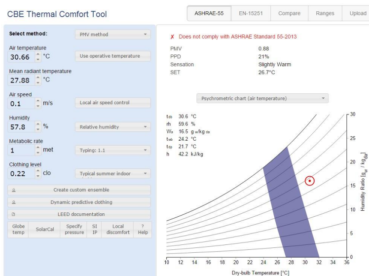
Ilustración 44 Tabulación de datos para hallar el pmv y ppd, (T7-apto302). Elaboración a partir de la herramienta - CBE Thermal Comfort Tool
