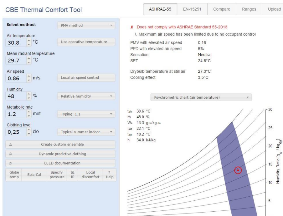
Ilustración 58 Tabulación de datos para hallar el pmv y ppd, (T1-apto205). Elaboración a partir de la herramienta - CBE Thermal Comfort Tool
