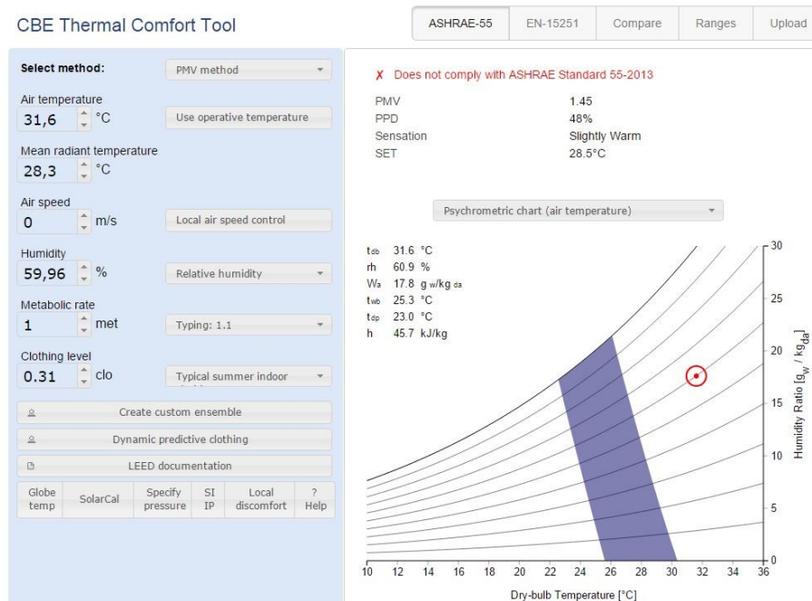
Ilustración 35 Tabulación de datos para hallar el pmv y ppd, (T6-apto206). Elaboración a partir de la herramienta - CBE Thermal Comfort Tool
