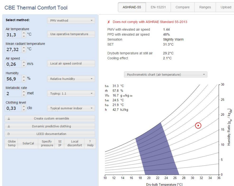
Ilustración 34 Tabulación de datos para hallar el pmv y ppd, (T6-apto204). Elaboración a partir de la herramienta - CBE Thermal Comfort Tool
