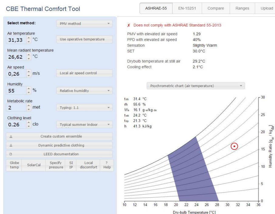
Ilustración 36 Tabulación de datos para hallar el pmv y ppd, (T6-apto304). Elaboración a partir de la herramienta - CBE Thermal Comfort Tool
