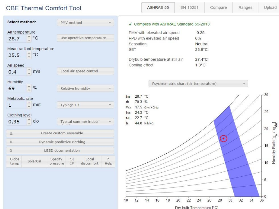
Ilustración 57 Tabulación de datos para hallar el pmv y ppd, (T1-apto204). Elaboración a partir de la herramienta - CBE Thermal Comfort Tool
