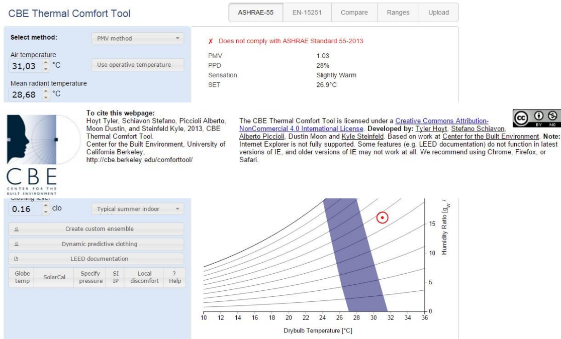
Ilustración 25 Ilustración 18 Tabulación de datos para hallar el pmv y ppd, (T14-apto206). Elaboración a partir de la herramienta - CBE Thermal Comfort Tool
