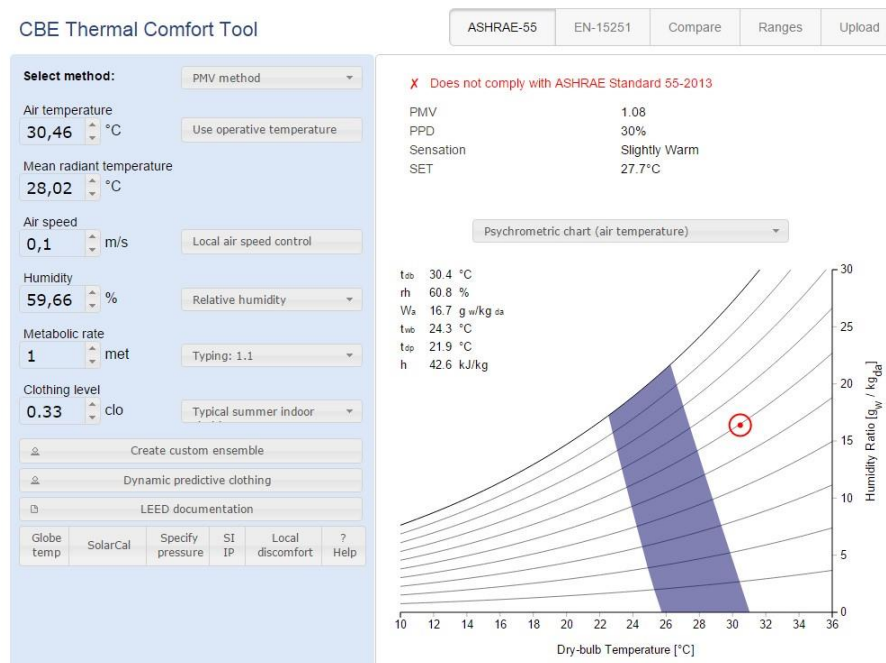
Ilustración 24 Tabulación de datos para hallar el pmv y ppd, [T14-apto205]. Elaboración a partir de la herramienta - CBE Thermal Comfort Tool
