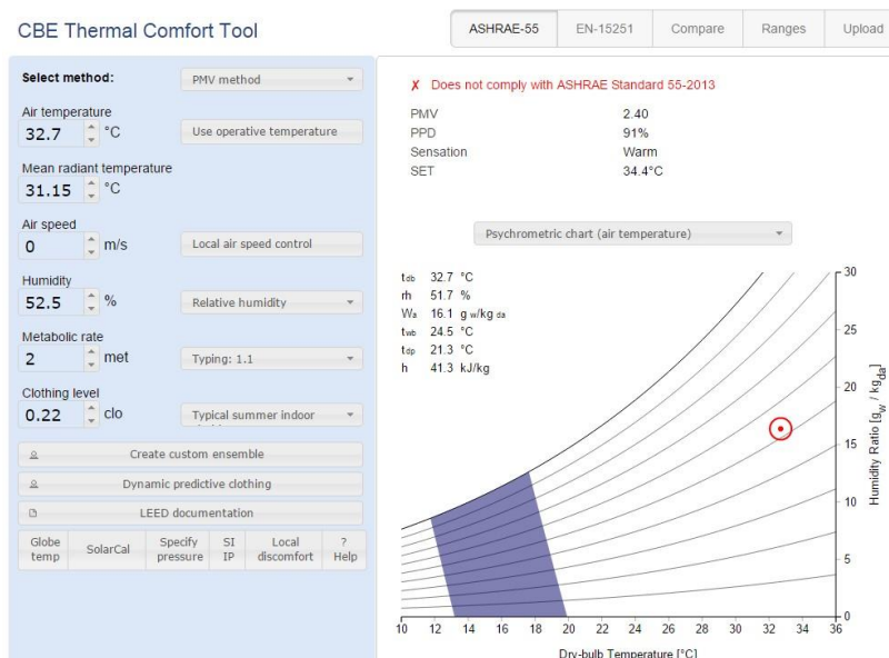
Ilustración 54 Tabulación de datos para hallar el pmv y ppd, (T8-apto305). Elaboración a partir de la herramienta - CBE Thermal Comfort Tool
