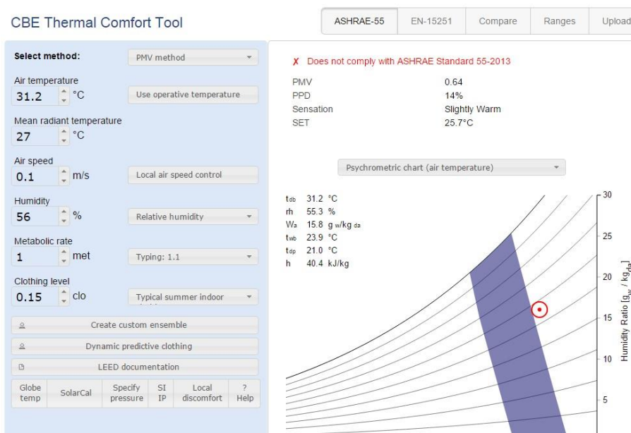
Ilustración 38 Tabulación de datos para hallar el pmv y ppd, (T6-apto404). Elaboración a partir de la herramienta - CBE Thermal Comfort Tool
