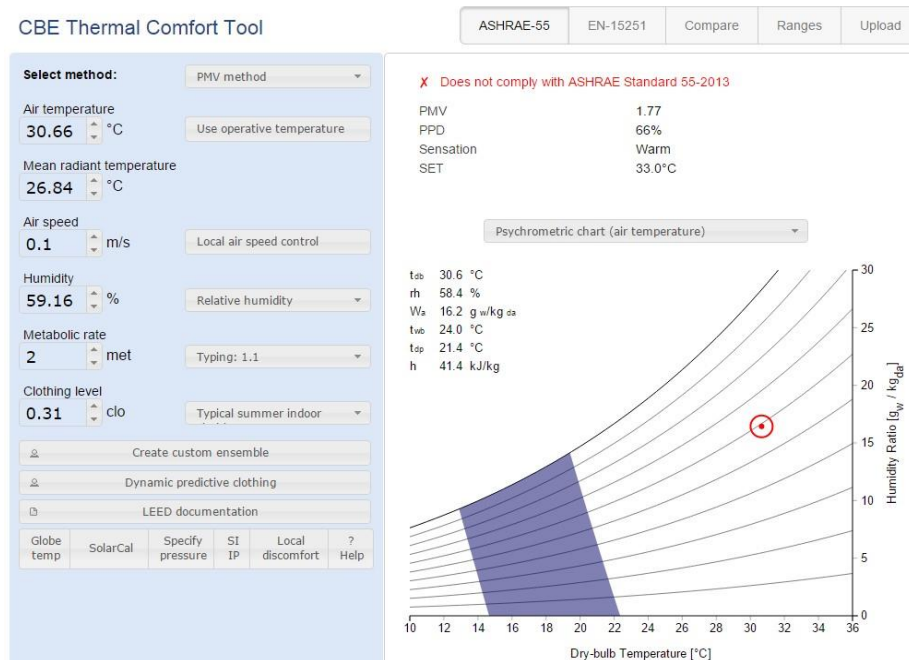
Ilustración 45 Tabulación de datos para hallar el pmv y ppd, (T7-apto303). Elaboración a partir de la herramienta - CBE Thermal Comfort Tool
