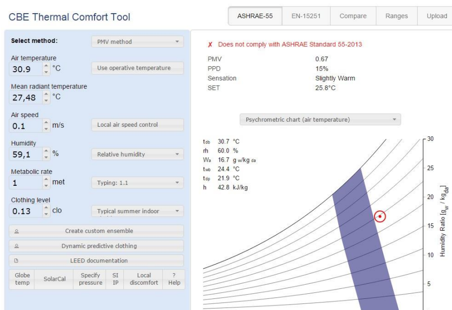
Ilustración 40 Tabulación de datos para hallar el pmv y ppd, (T7-apto201). Elaboración a partir de la herramienta - CBE Thermal Comfort Tool
