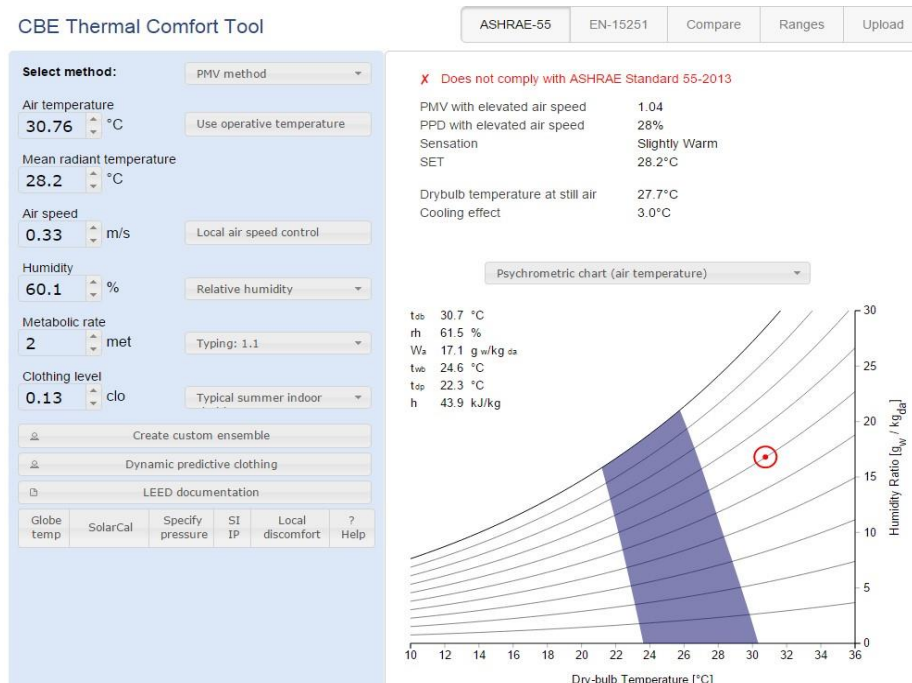
Ilustración 47 Tabulación de datos para hallar el pmv y ppd, (T7-apto402). Elaboración a partir de la herramienta - CBE Thermal Comfort Tool
