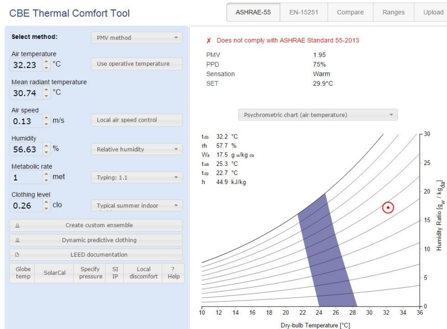
Ilustración 51 Tabulación de datos para hallar el pmv y ppd, (T8-apto204). Elaboración a partir de la herramienta - CBE Thermal Comfort Tool
