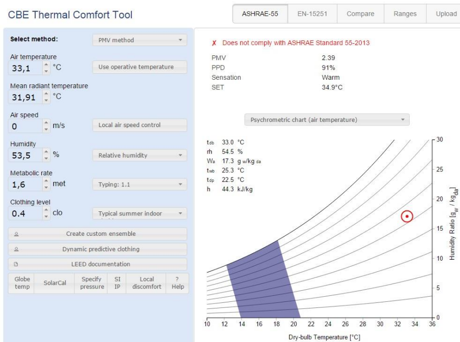
Ilustración 32 Tabulación de datos para hallar el pmv y ppd, (T3-apto401). Elaboración a partir de la herramienta - CBE Thermal Comfort Tool
