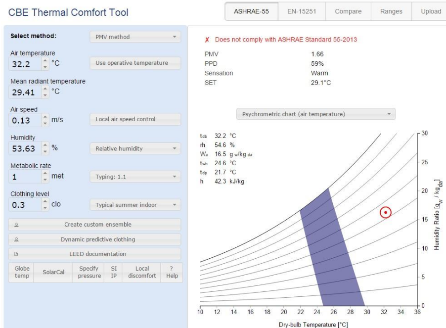
Ilustración 49 Tabulación de datos para hallar el pmv y ppd, (T8-apto201). Elaboración a partir de la herramienta - CBE Thermal Comfort Tool
