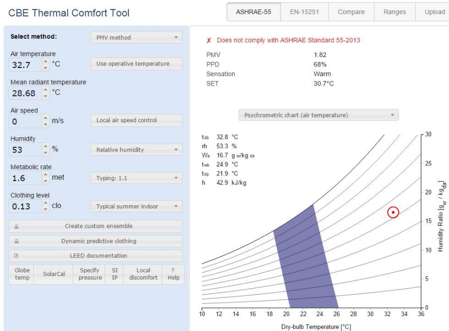
Ilustración 53 Tabulación de datos para hallar el pmv y ppd, (T8-apto301). Elaboración a partir de la herramienta - CBE Thermal Comfort Tool
