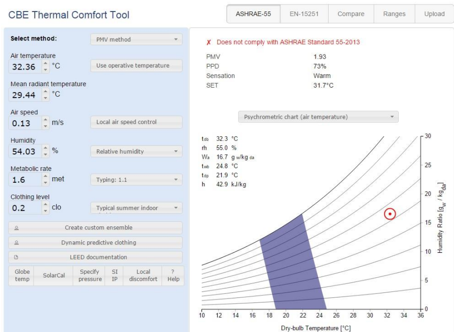
Ilustración 55 Tabulación de datos para hallar el pmv y ppd, (T8-apto306). Elaboración a partir de la herramienta - CBE Thermal Comfort Tool
