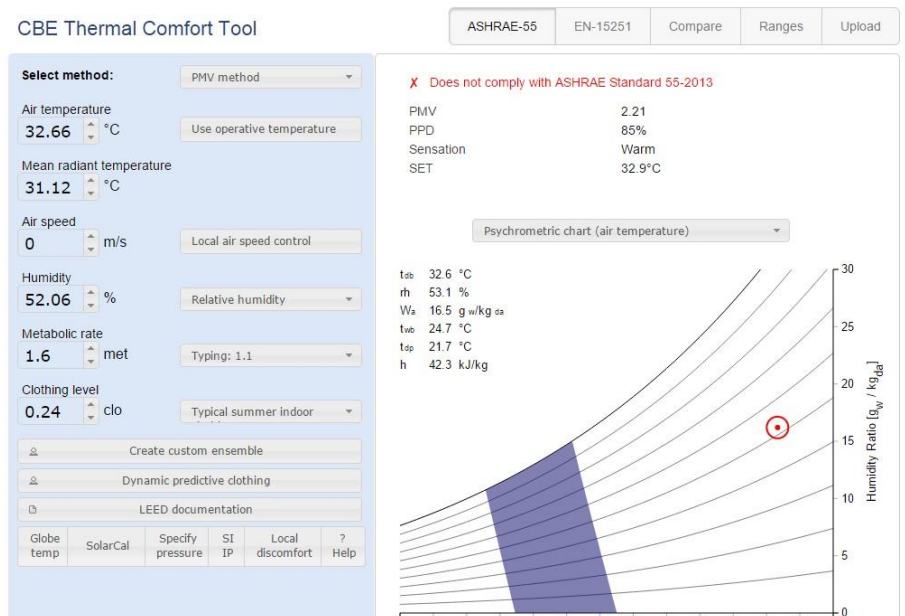
Ilustración 56 Tabulación de datos para hallar el pmv y ppd, (T8-apto401). Elaboración a partir de la herramienta - CBE Thermal Comfort Tool
