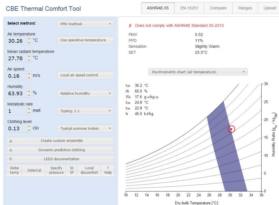
Ilustración 43 Tabulación de datos para hallar el pmv y ppd, (T7-apto301). Elaboración a partir de la herramienta - CBE Thermal Comfort Tool
