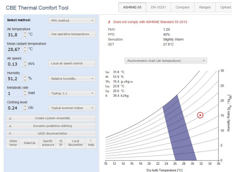
Ilustración 30 Tabulación de datos para hallar el pmv y ppd, (T3-apto203). Elaboración a partir de la herramienta - CBE Thermal Comfort Tool
