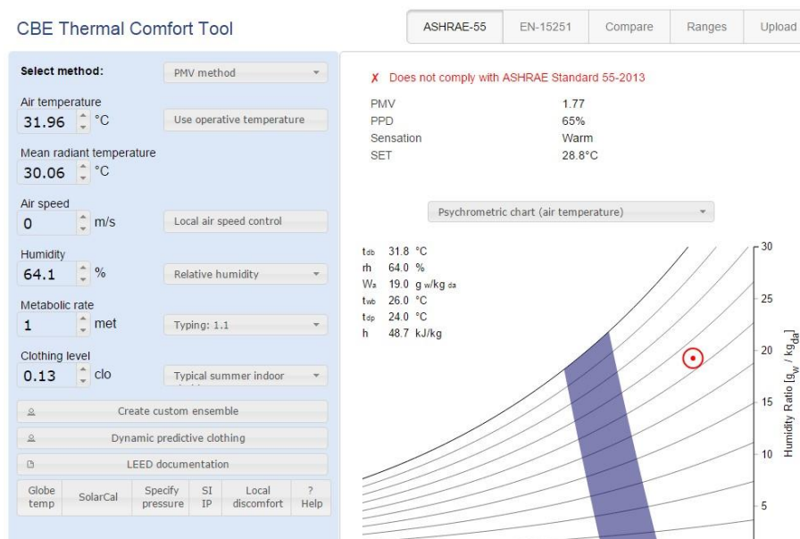
Ilustración 52 Tabulación de datos para hallar el pmv y ppd, (T8-apto206). Elaboración a partir de la herramienta - CBE Thermal Comfort Tool
