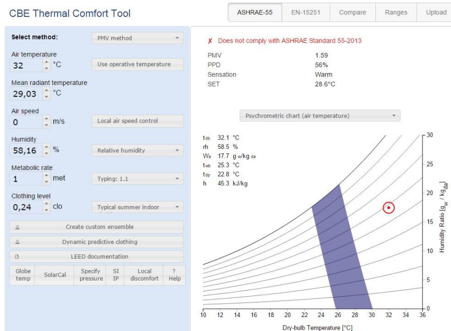
Ilustración 33 Tabulación de datos para hallar el pmv y ppd, (T3-apto402). Elaboración a partir de la herramienta - CBE Thermal Comfort Tool
