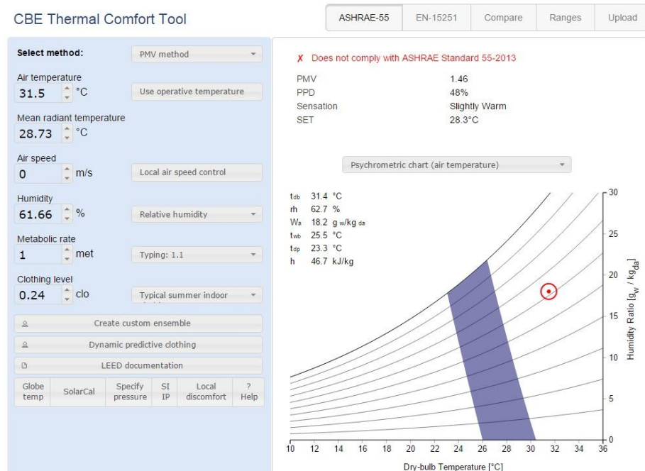
Ilustración 46 Tabulación de datos para hallar el pmv y ppd, (T7-apto401). Elaboración a partir de la herramienta - CBE Thermal Comfort Tool
