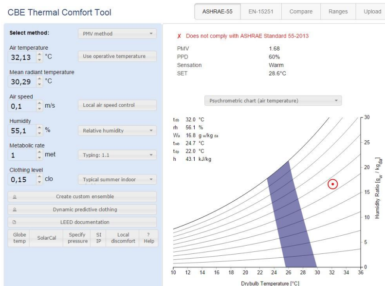
Ilustración 27 Tabulación de datos para hallar el pmv y ppd, (T14-apto305). Elaboración a partir de la herramienta - CBE Thermal Comfort Tool
