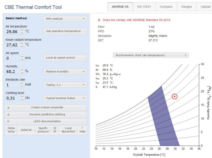
Ilustración 28 Tabulación de datos para hallar el pmv y ppd, (T14-apto306). Elaboración a partir de la herramienta - CBE Thermal Comfort Tool
