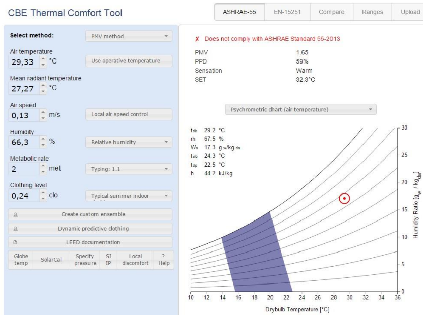
Ilustración 26 Ilustración 18 Tabulación de datos para hallar el pmv y ppd, (T14-apto304). Elaboración a partir de la herramienta - CBE Thermal Comfort Tool
