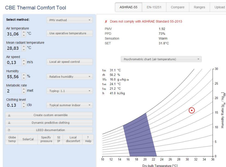
Ilustración 37 Tabulación de datos para hallar el pmv y ppd, (T6-apto305). Elaboración a partir de la herramienta - CBE Thermal Comfort Tool
