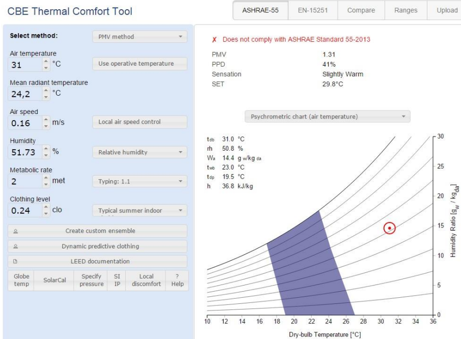
Ilustración 41 Tabulación de datos para hallar el pmv y ppd, (T7-apto202). Elaboración a partir de la herramienta - CBE Thermal Comfort Tool
