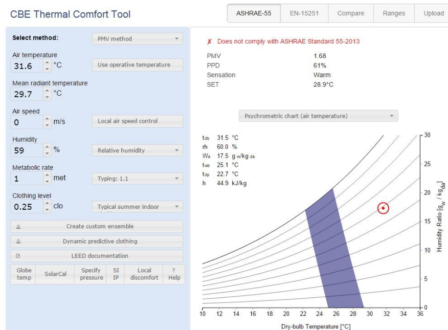
Ilustración 60 Tabulación de datos para hallar el pmv y ppd, (T1-apto305). Elaboración a partir de la herramienta - CBE Thermal Comfort Tool
