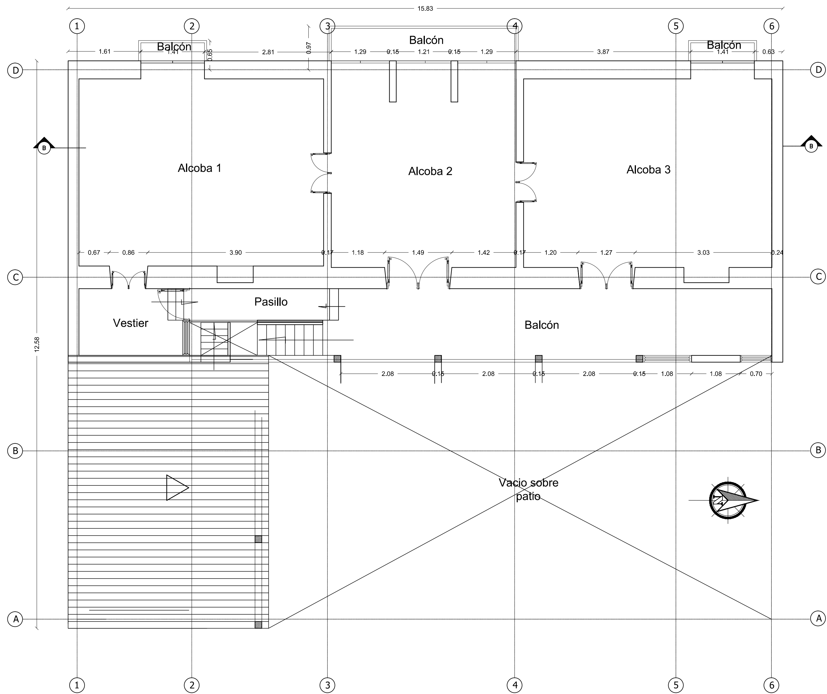
PLANTA SEGUNDO PISO (Existente) Escala _____1:50
