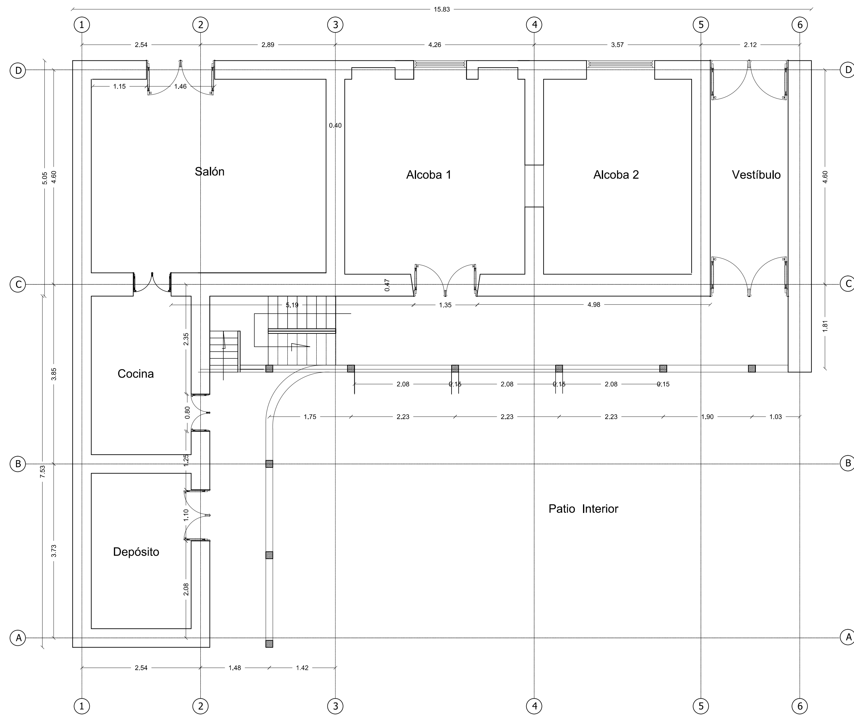
PLANTA PRIMER PISO (Existente) Escala _____1:50
