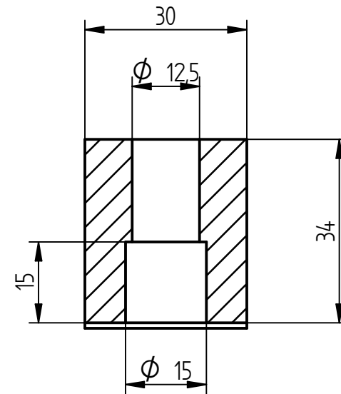
CORTE A-A
