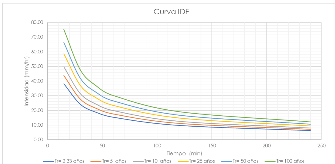
Figura 3-2 Curvas IDF, estación Inst Agr Sta Sofía Fuente: Consorcio Aguas de los Andes, 2018
