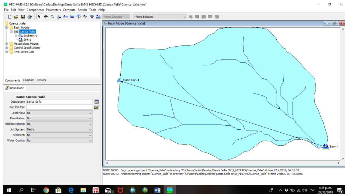
Figura 3-9 Cuenca El Valle, HEC-HMS Fuente. Consorcio Aguas de los Andes, 2018
