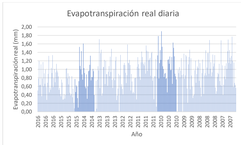
Figura 3-12 Evapotranspiración Real estimada para la cuenca El Valle
