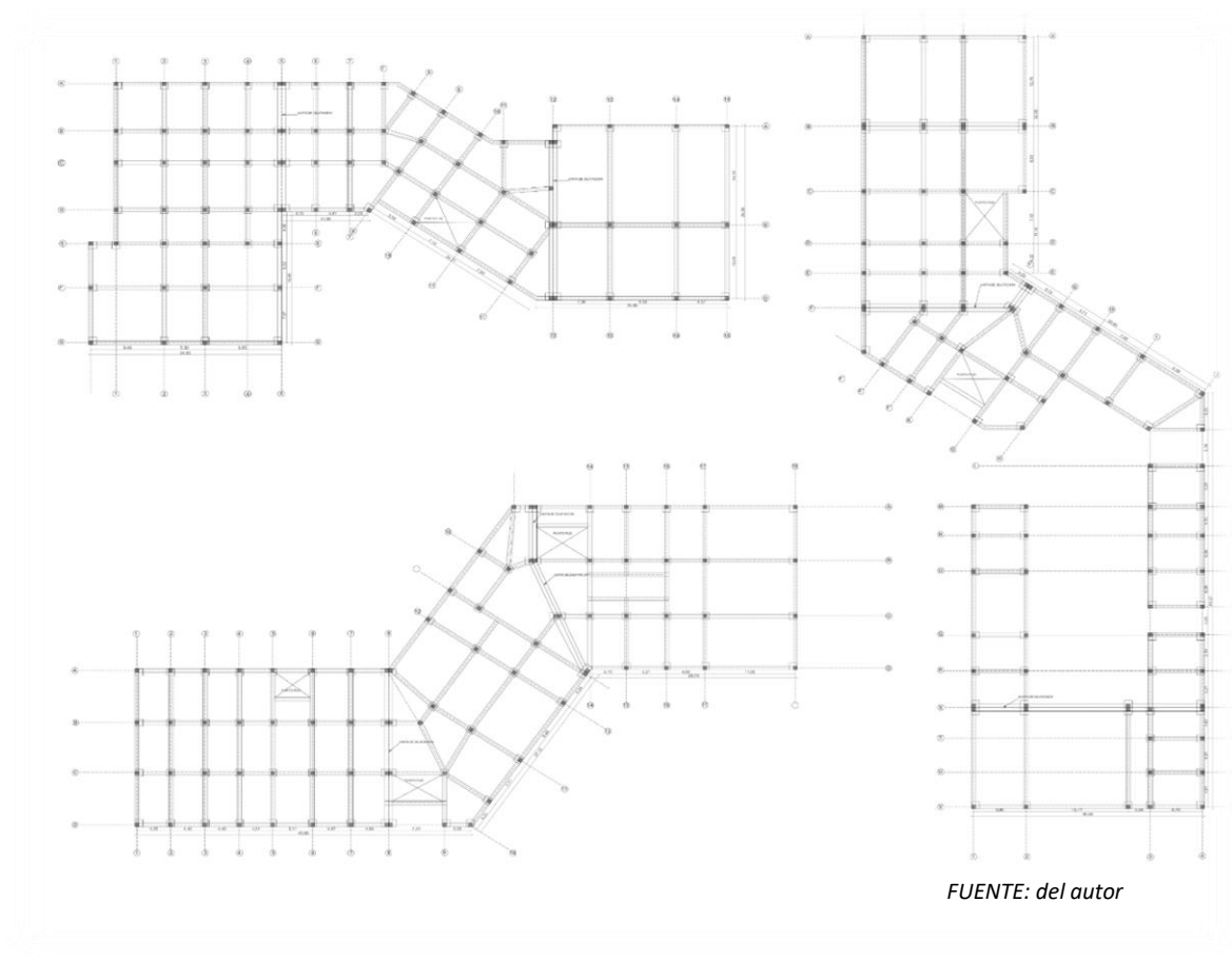
ILUSTRACION 50: Planta estructural
