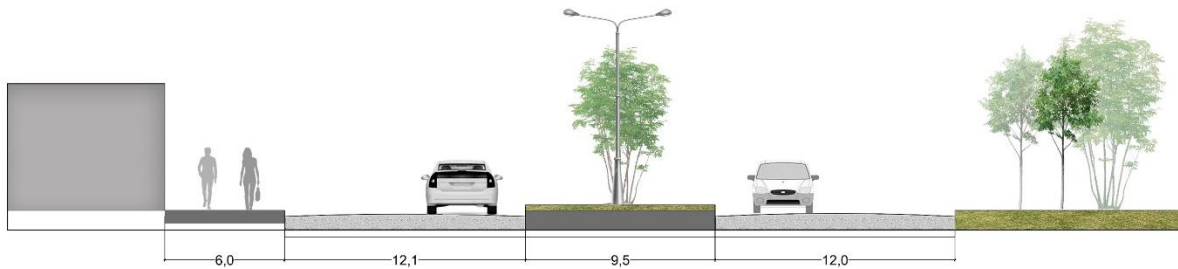
ILUSTRACION 31: Perfil Vial troncal del caribe
