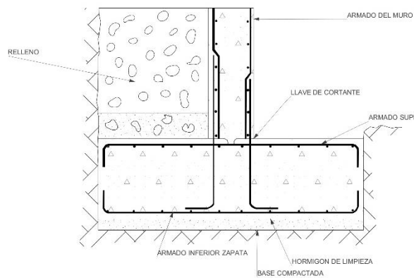
ILUSTRACION 52: detalle de zapata bajo muro
