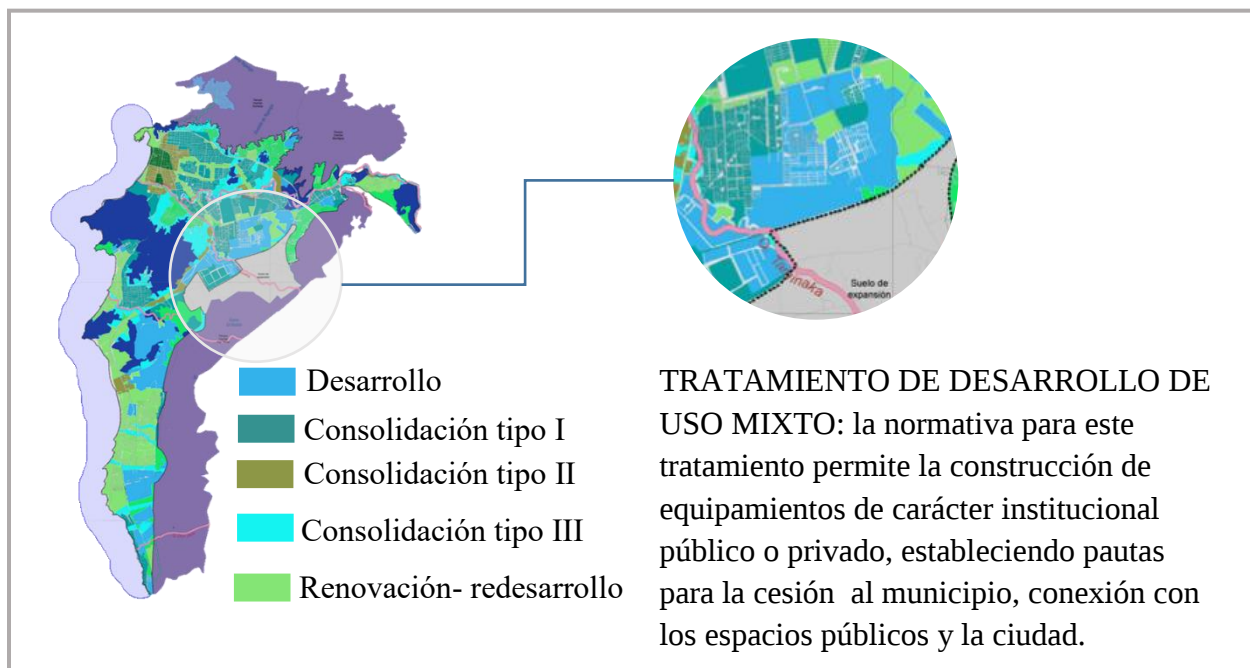
ILUSTRACION 19: Tratamientos del suelo de Santa Marta
