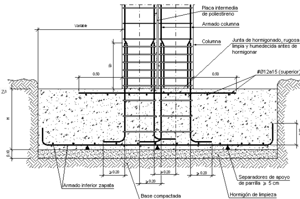
ILUSTRACION 53: detalle de zapata en junta de dilatación
