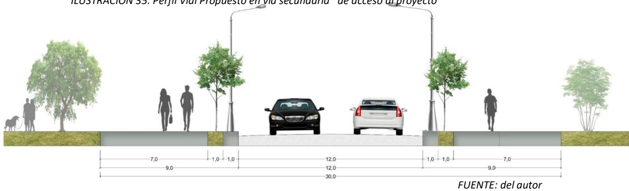
ILUSTRACION 35: Perfil Vial Propuesto en vía secundaria de acceso al proyecto
