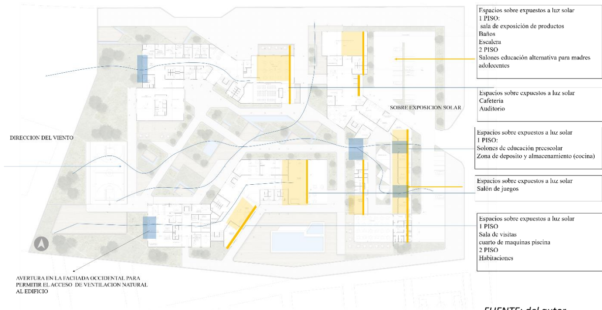
ILUSTRACION 55 : Análisis Bioclimático del proyecto
