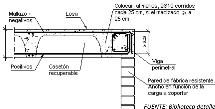
ILUSTRACION 54 detalle de apoyo de placa aligerada sobre muro
