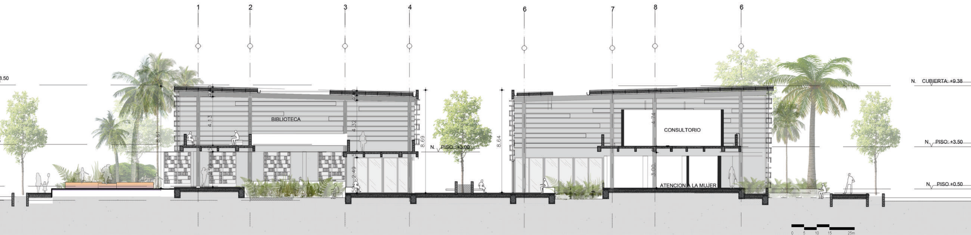
Figura 50. Sección transversal A-A. Garcés. J. (Agosto, 2018)
