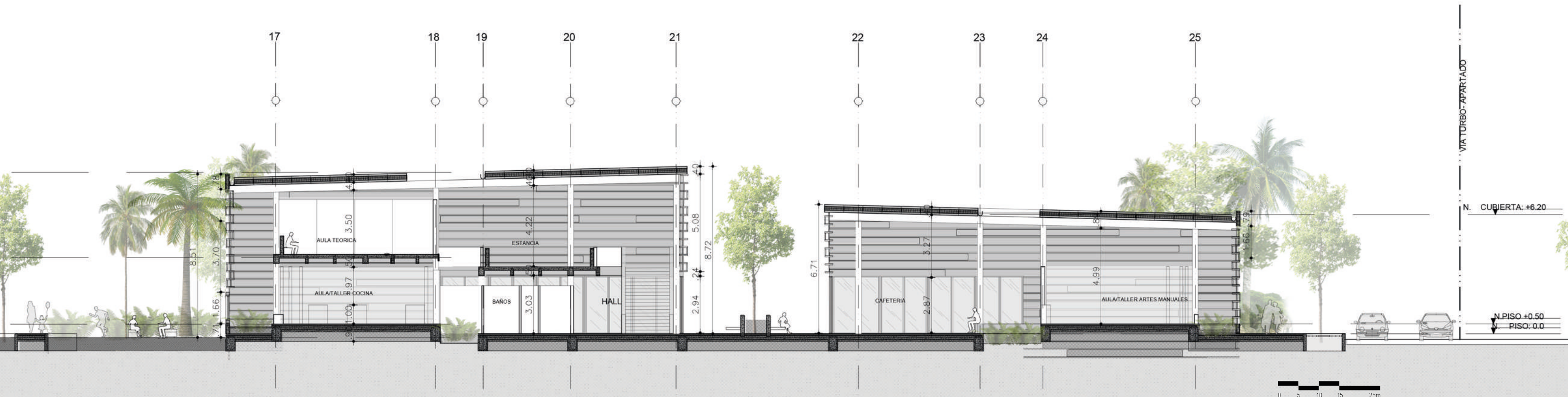
Figura 51. Sección transversal C-C. Garcés. J. (Agosto, 2018)
