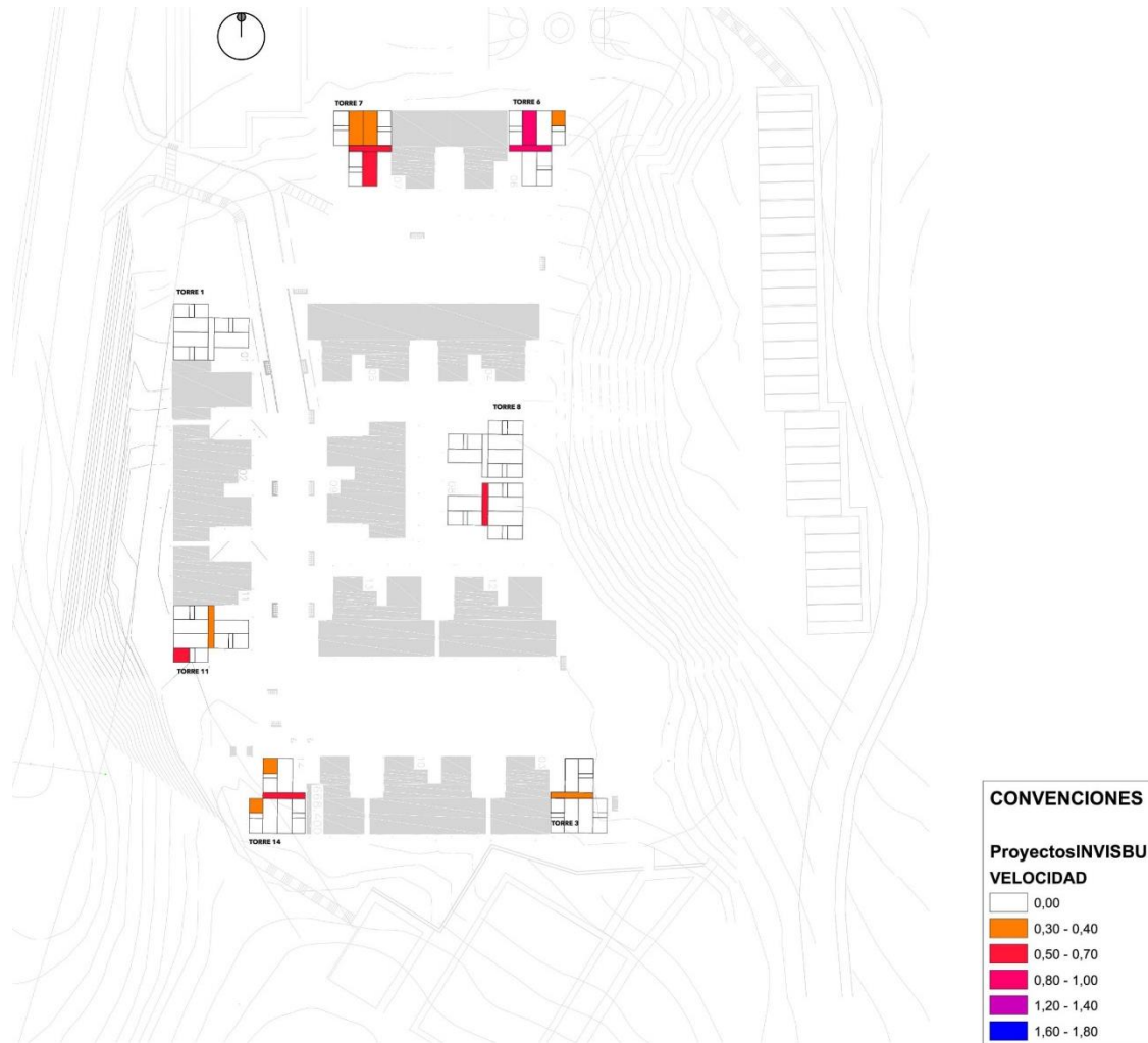
Ilustración 16 Velocidad del viento, basado en tomas de muestras en sitio, tercer piso, 2015. Fuente elaboración propia.
