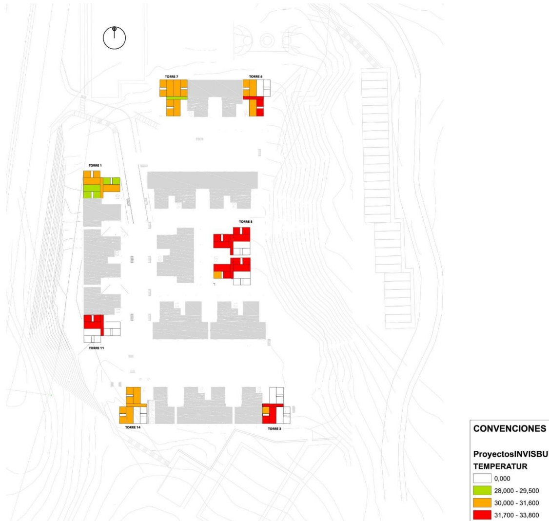
Ilustración 3 Temperatura ambiente, basado en tomas de muestras en sitio, segundo piso, 2015. Fuente elaboración propia.
