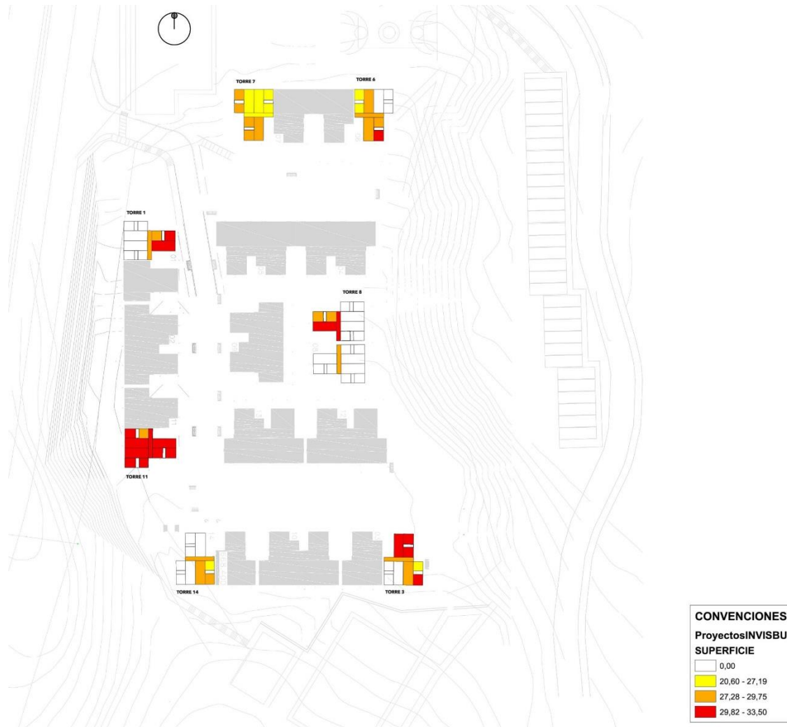
Ilustración 8 Temperatura media radiante, basado en tomas de muestras en sitio, cuarto piso, 2015. Fuente elaboración propia.
