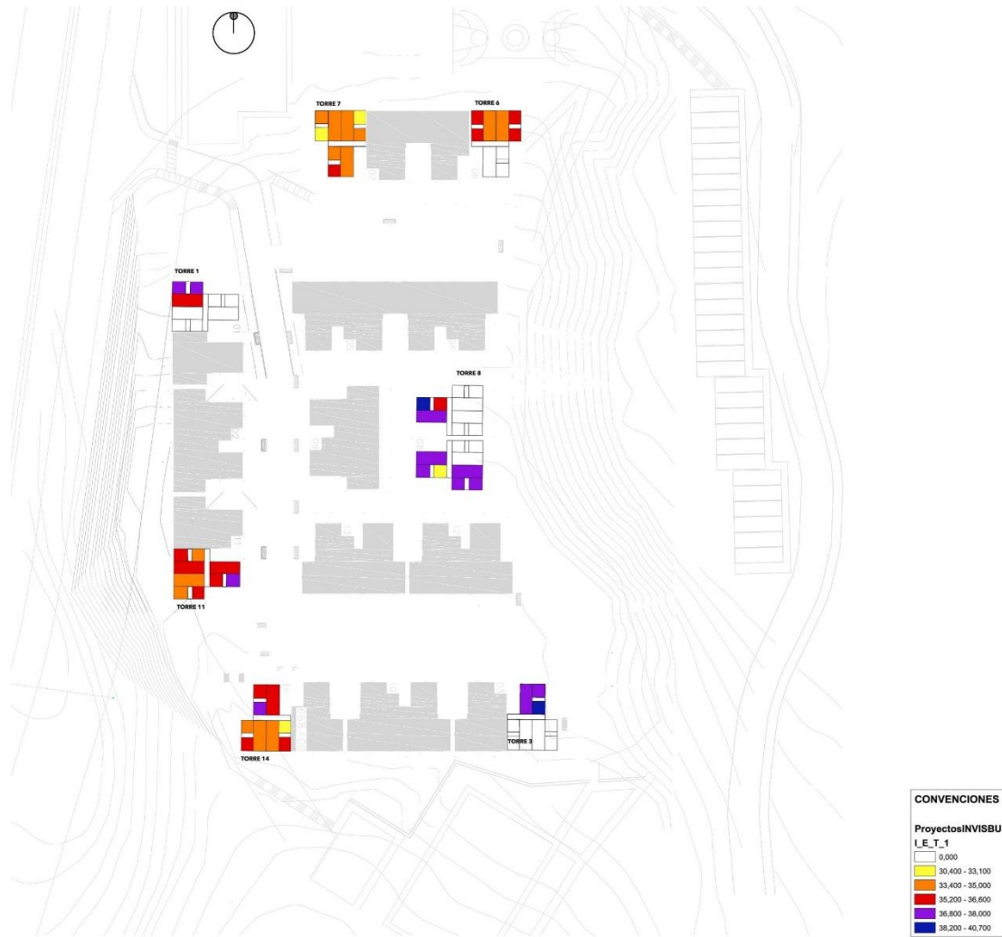
Ilustración 13 Estrés térmico, basado en tomas de muestras en sitio, tercer piso, 2015. Fuente elaboración propia.
