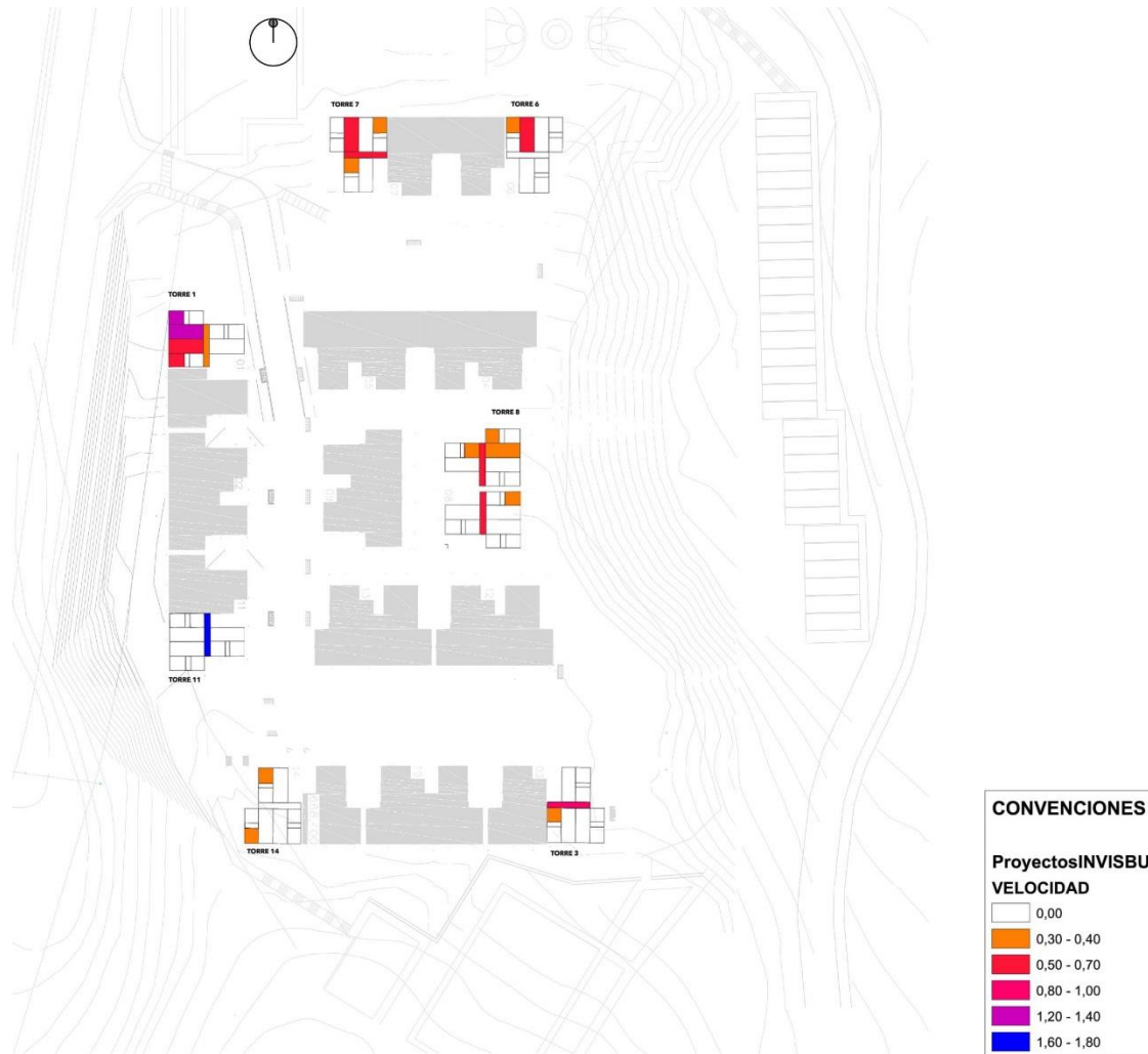
Ilustración 15 Velocidad del viento, basado en tomas de muestras en sitio, segundo piso, 2015. Fuente elaboración propia.
