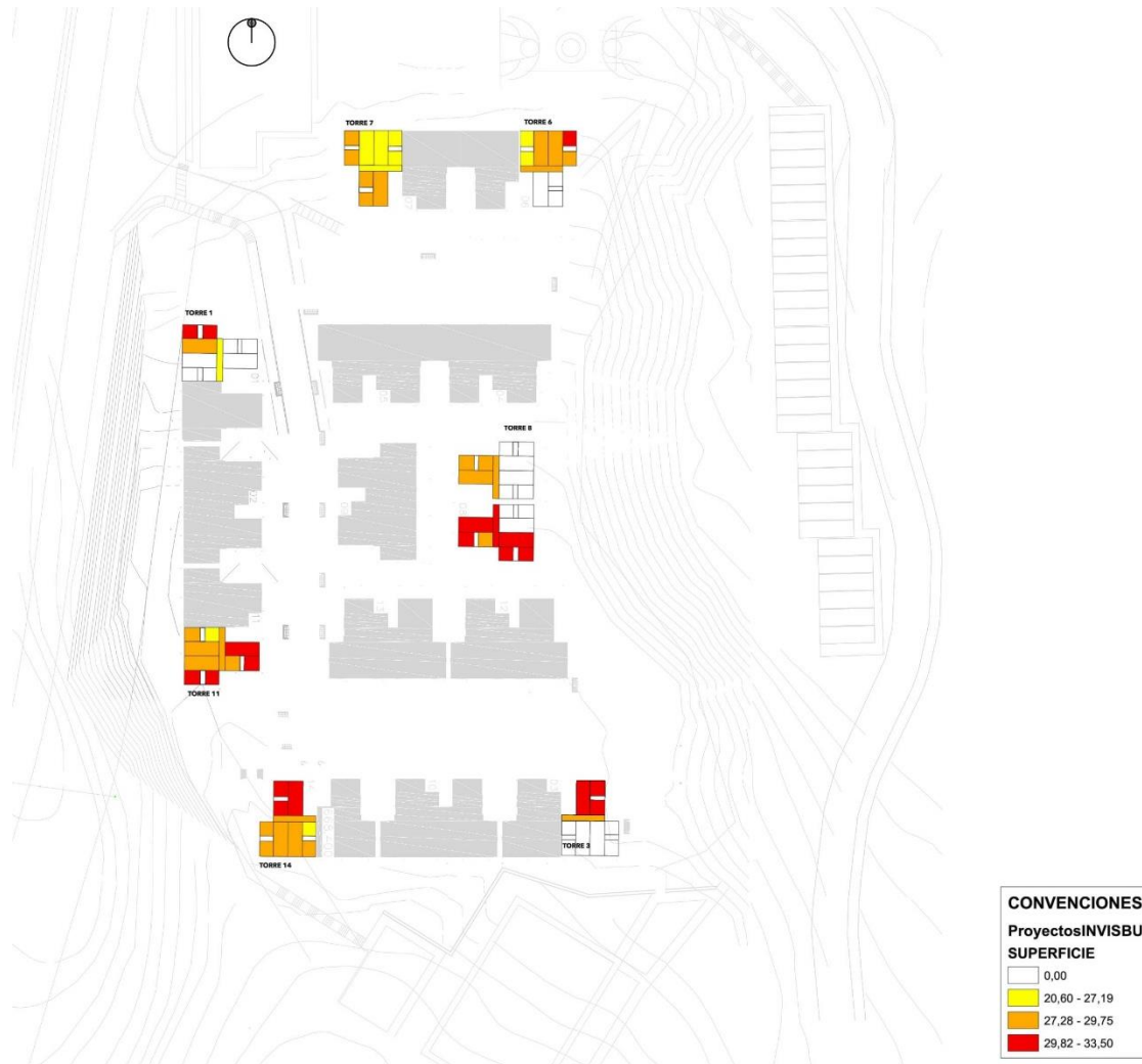
Ilustración 7 Temperatura media radiante, basado en tomas de muestras en sitio, tercer piso, 2015. Fuente elaboración propia.
