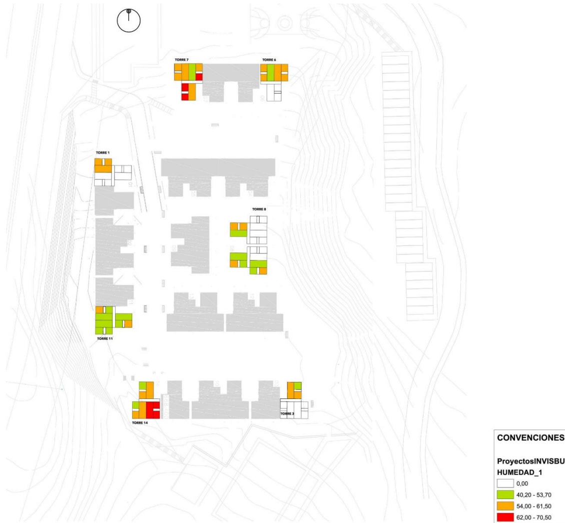
Ilustración 10 Humedad relativa, basado en tomas de muestras en sitio, tercer piso, 2015. Fuente elaboración propia.
