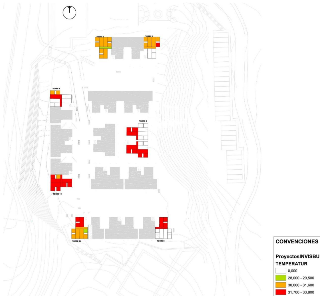
Ilustración 4 Temperatura ambiente, basado en tomas de muestras en sitio, tercer piso, 2015. Fuente elaboración propia.
