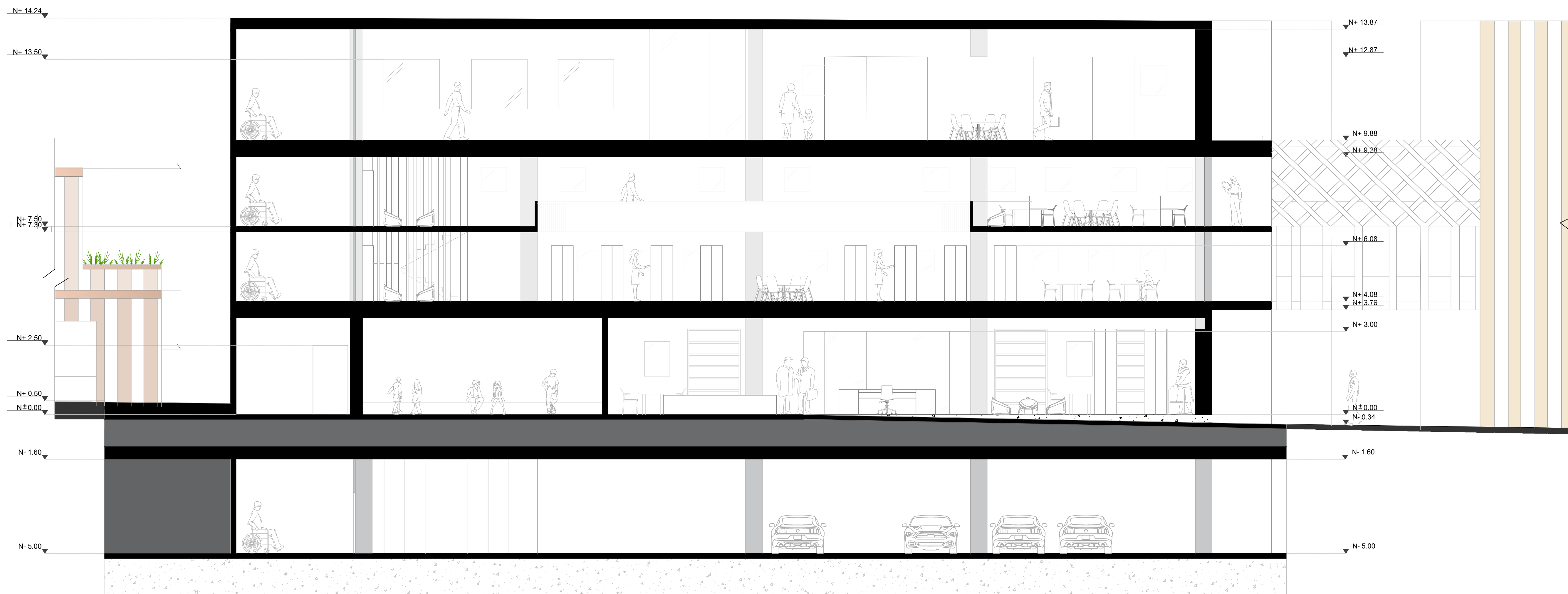
A21 CORTE LONGITUDINAL BB ESC 1:80
