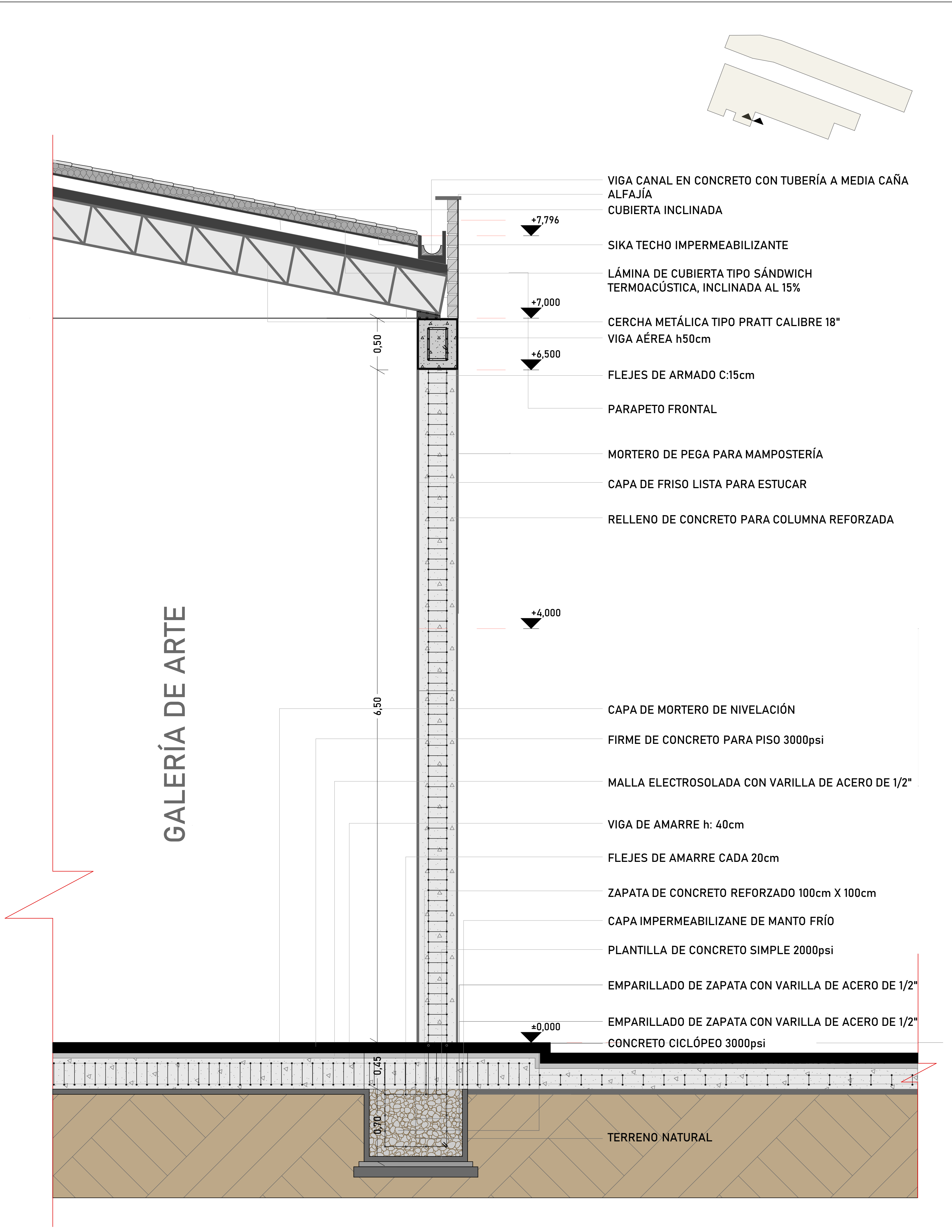
CORTE POR FACHADA #2 ESC_1:20
