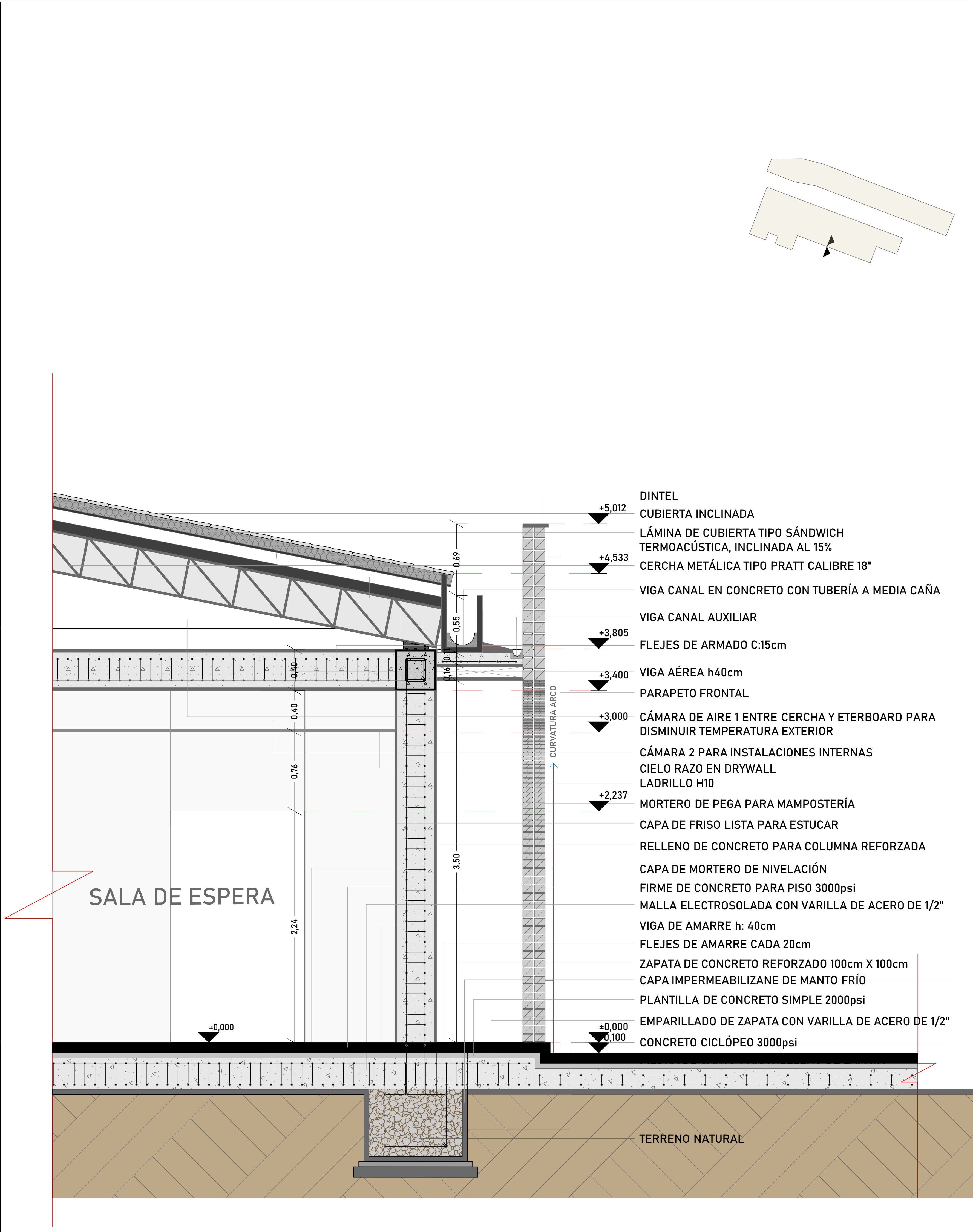
CORTE POR FACHADA #1 ESC_1:20
