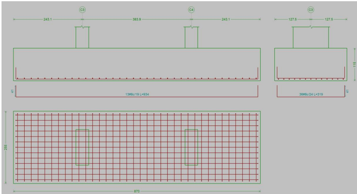
Ilustración 6. Despiece zapata tipo 6
