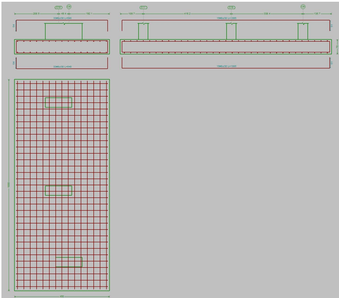
Ilustración 3. Despiece zapata tipo 3
