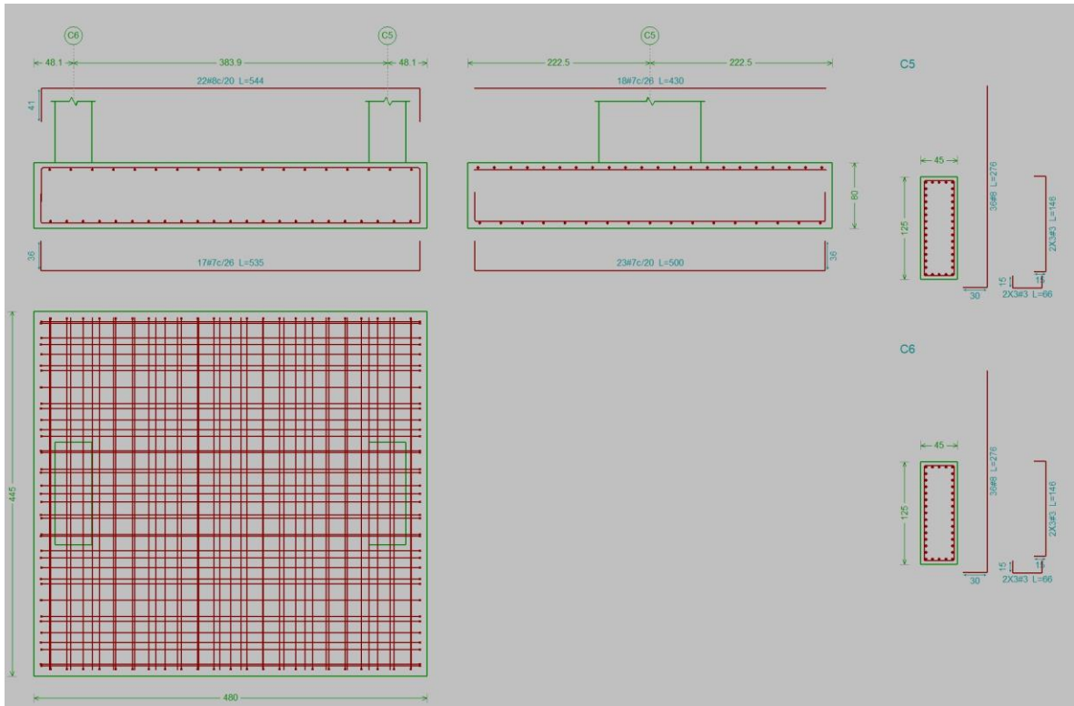
Ilustración 1. Despiece zapata tipo 1
