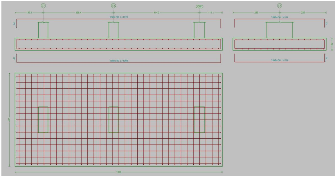
Ilustración 4. Despiece zapata tipo 4
