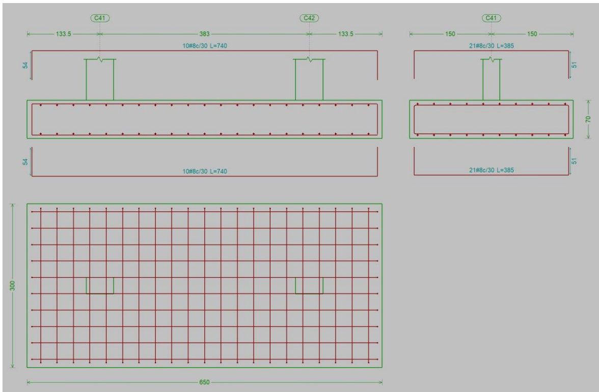
Ilustración 5. Despiece zapata tipo 5
