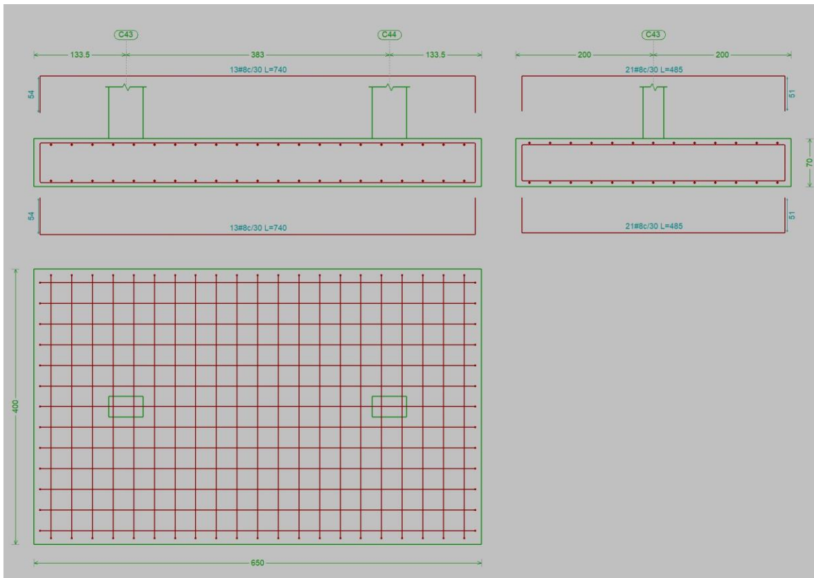
Ilustración 2. Despiece zapata tipo 2
