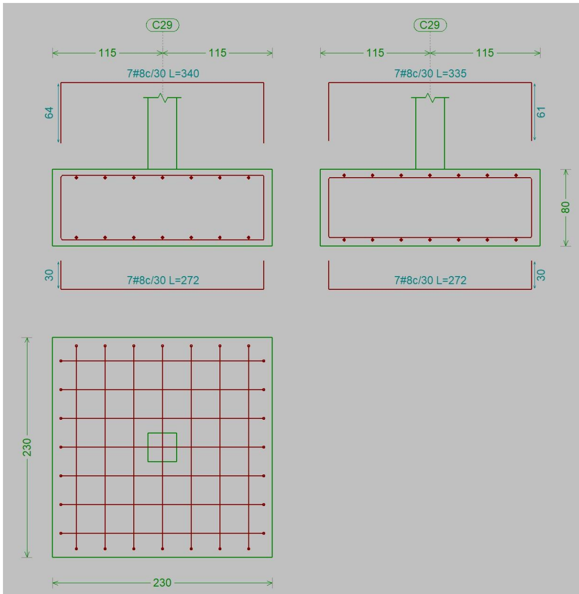
Ilustración 7. Despiece zapata tipo 7
