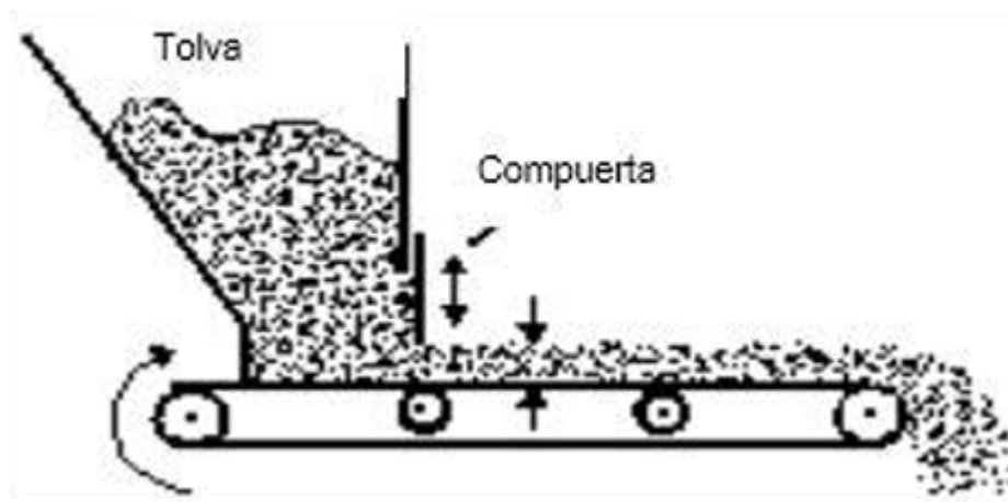
Figura 5. Dosificador de banda rodante
