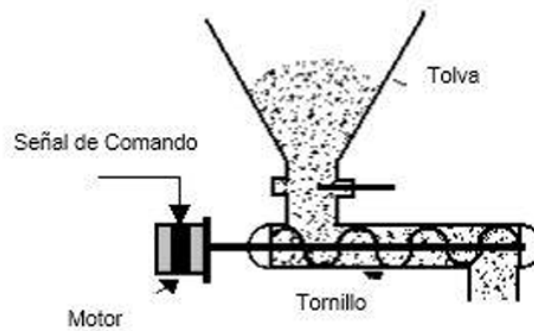
Figura 3. Dosificador de tornillo
