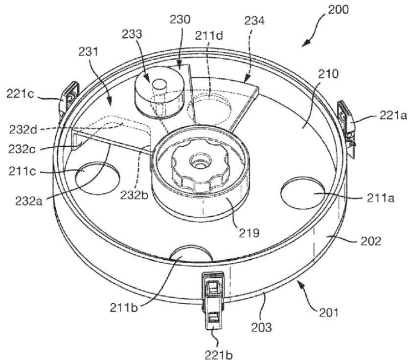
Figura 17. Mecanismo de la patente No° ES2844977
