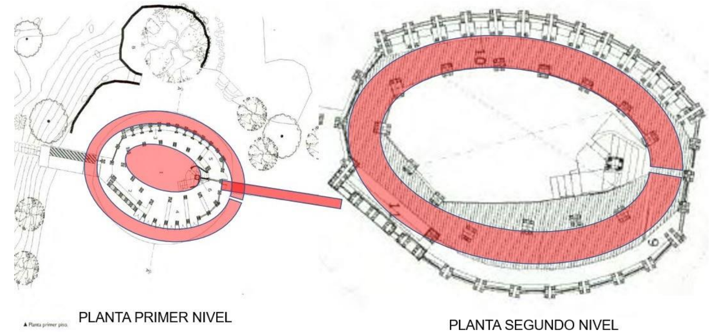
Figura 48 – imagen de planos de biblioteca – casa del pueblo intervenida – sistema de circulación y conexión
