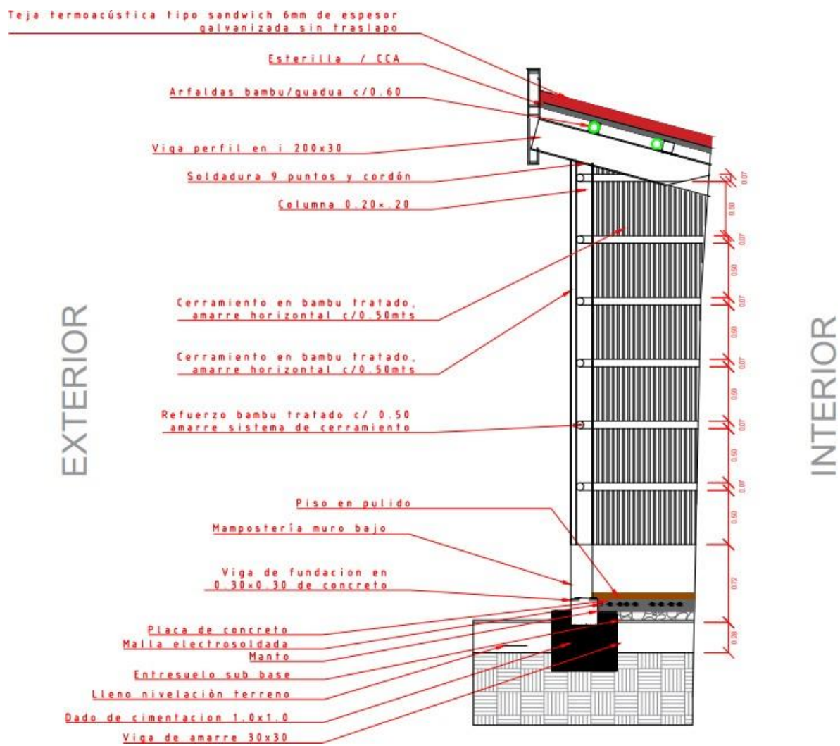
Figura 70 – Imaginario – sección – corte por fachada proyecto( fuente elaboración propia 2021)
