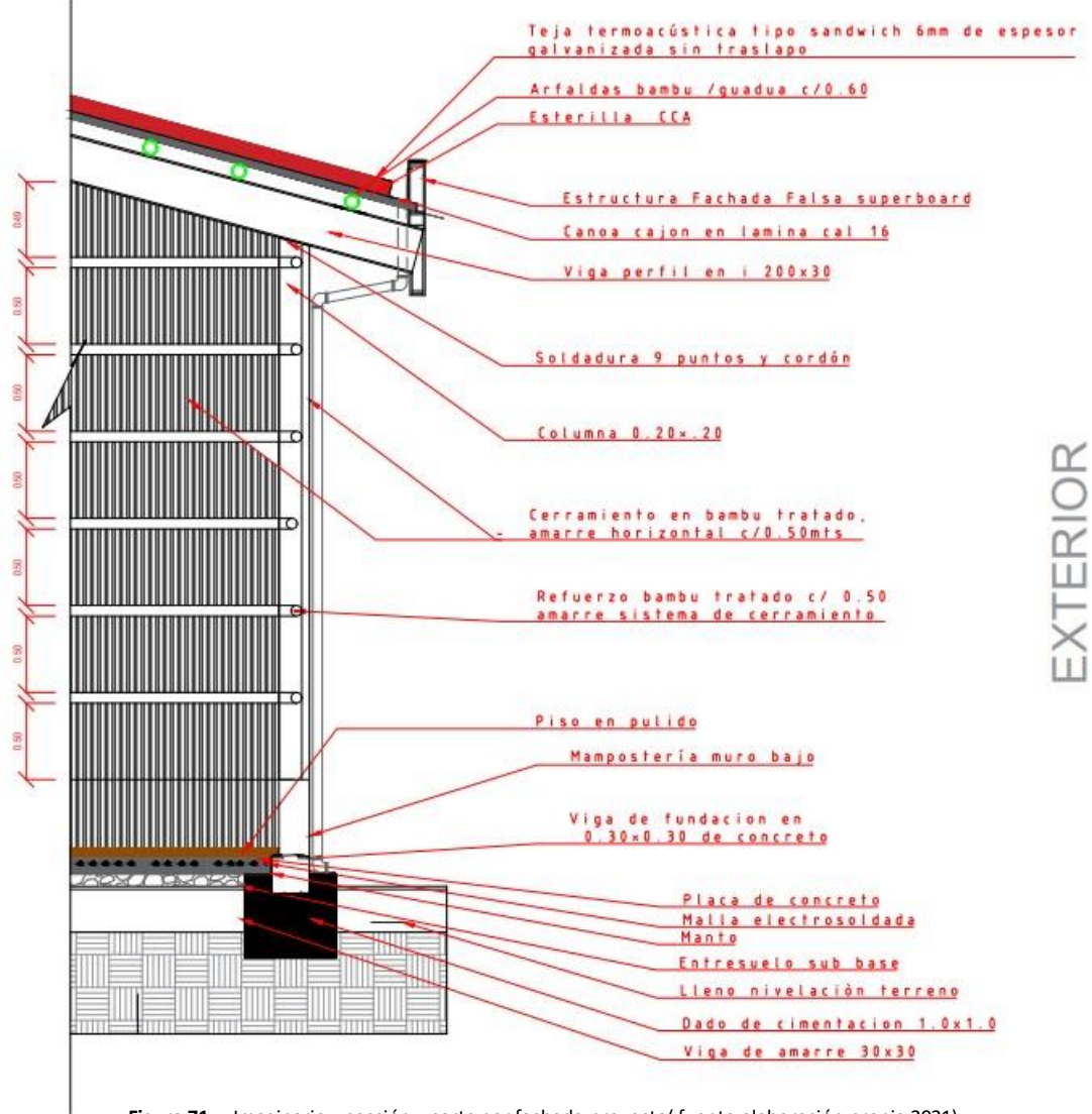
Figura 71 – Imaginario – sección – corte por fachada proyecto( fuente elaboración propia 2021)
