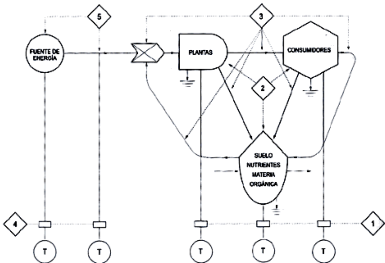
Figura 2, Estratégias de restauración según tipos de tensionantes
