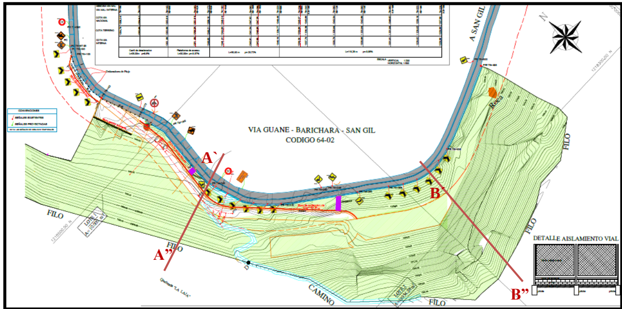
Figura 15. Cortes topográficos
