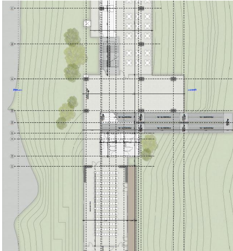
Figura 97. Planta nivel -8.00
