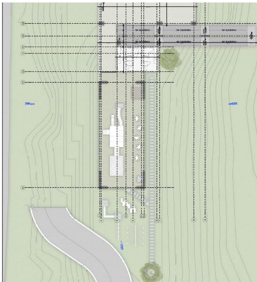
Figura 98. Planta nivel -12.00
