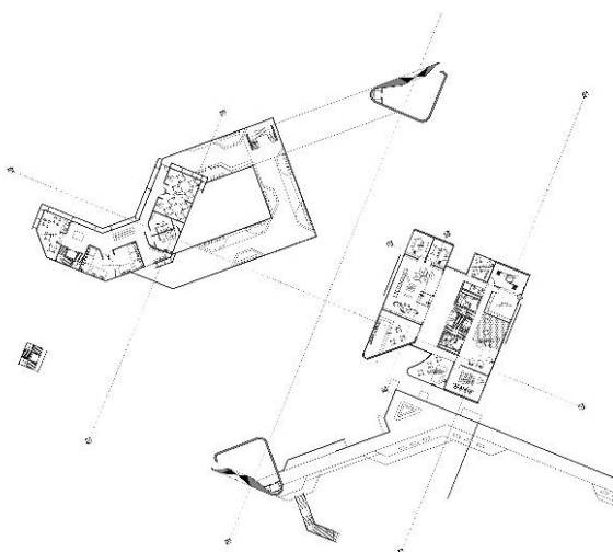
Planimetría 5: Planta segundo piso
