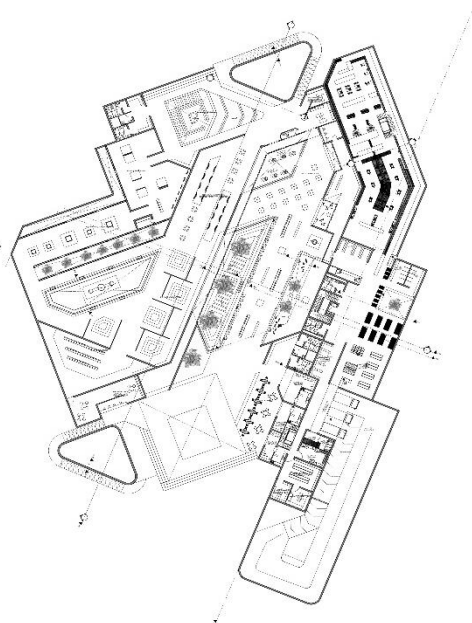
Planimetría 8: Planta subterránea Fuente: Elaboración propia
