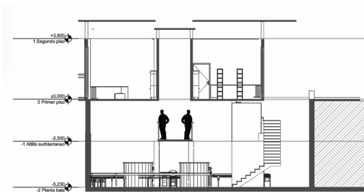
Planimetría 11: Corte A-4 detalle de área de productividad Fuente: elaboración propia
