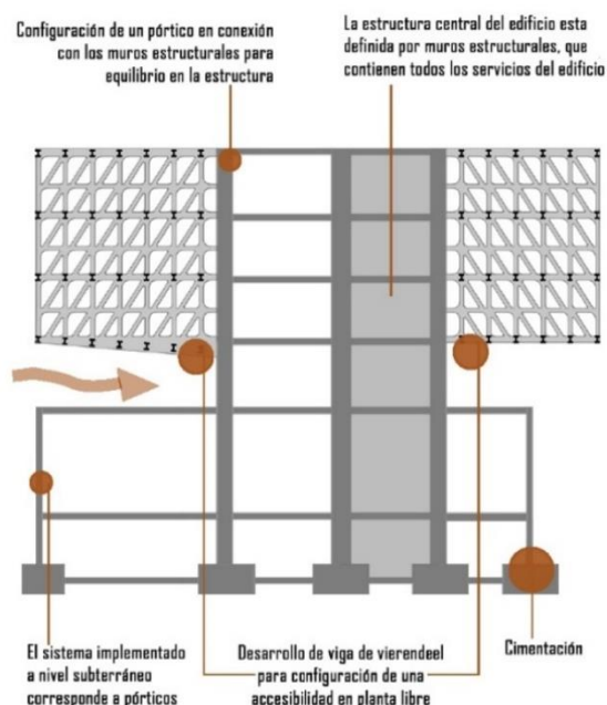
Planimetría 16 :Corte E-1 Fuente: Elaboración propia
