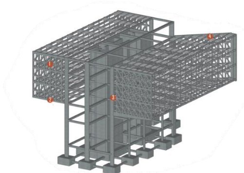
Ilustración 60: Modelo 3D del sistema de vierendeel Fuente: Elaboración propia
