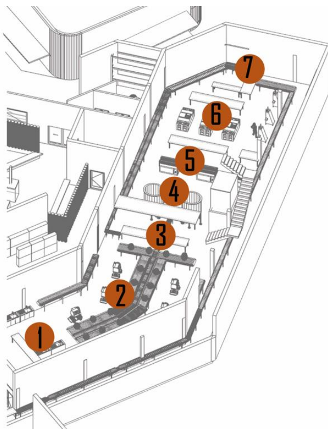
Ilustración 50: Isométrico de la función del área productiva Función: elaboración propia
