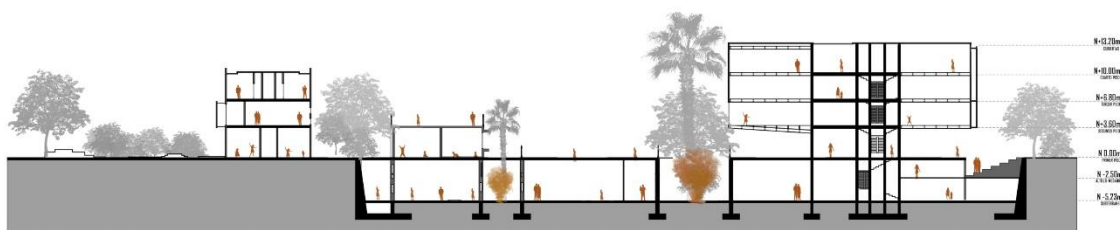
Planimetría 13: Corte A-3 Fuente: Elaboración propia
