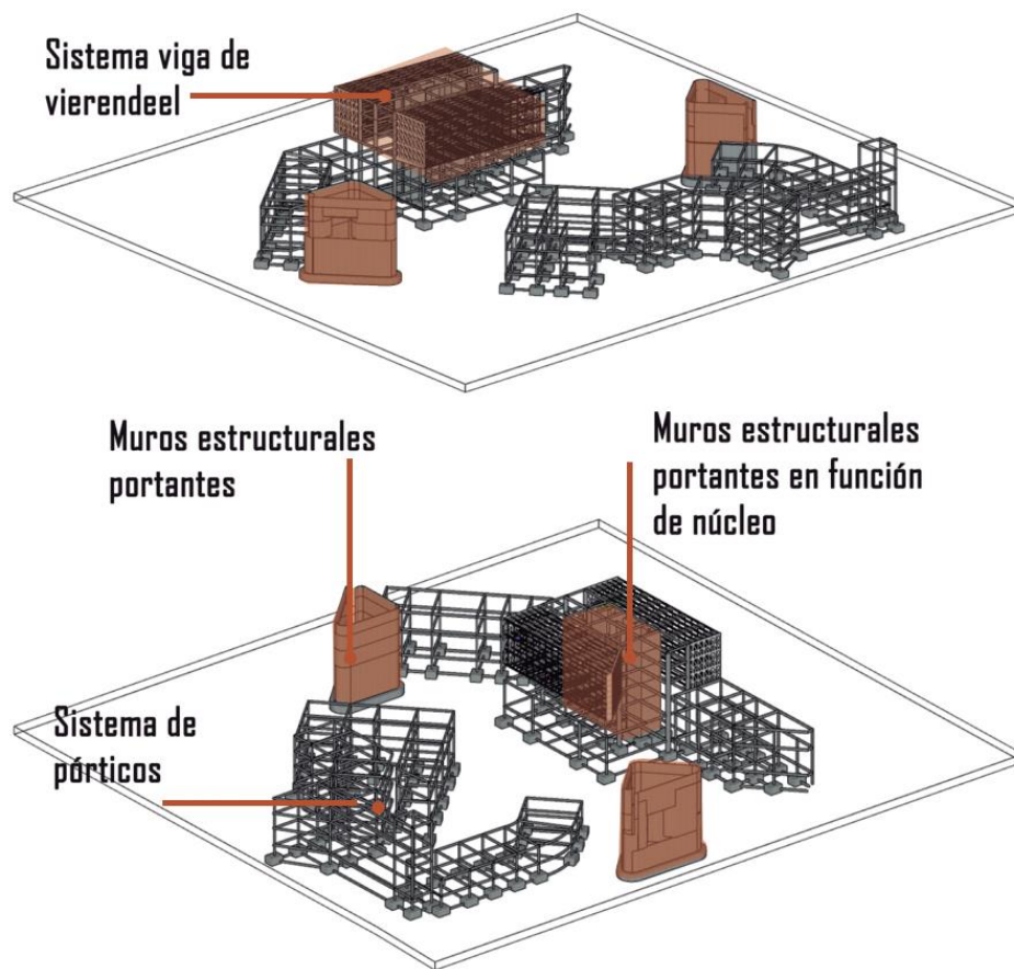
Ilustración 55: Disposición del sistema estructural Fuente; Elaboración propia
