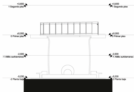
Planimetría 10: Detalle de vacío de agua Fuente: Elaboración propia
