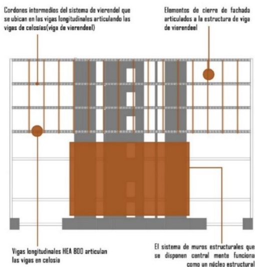
Planimetría 17: Corte E-2 Fuente: Elaboración propia
