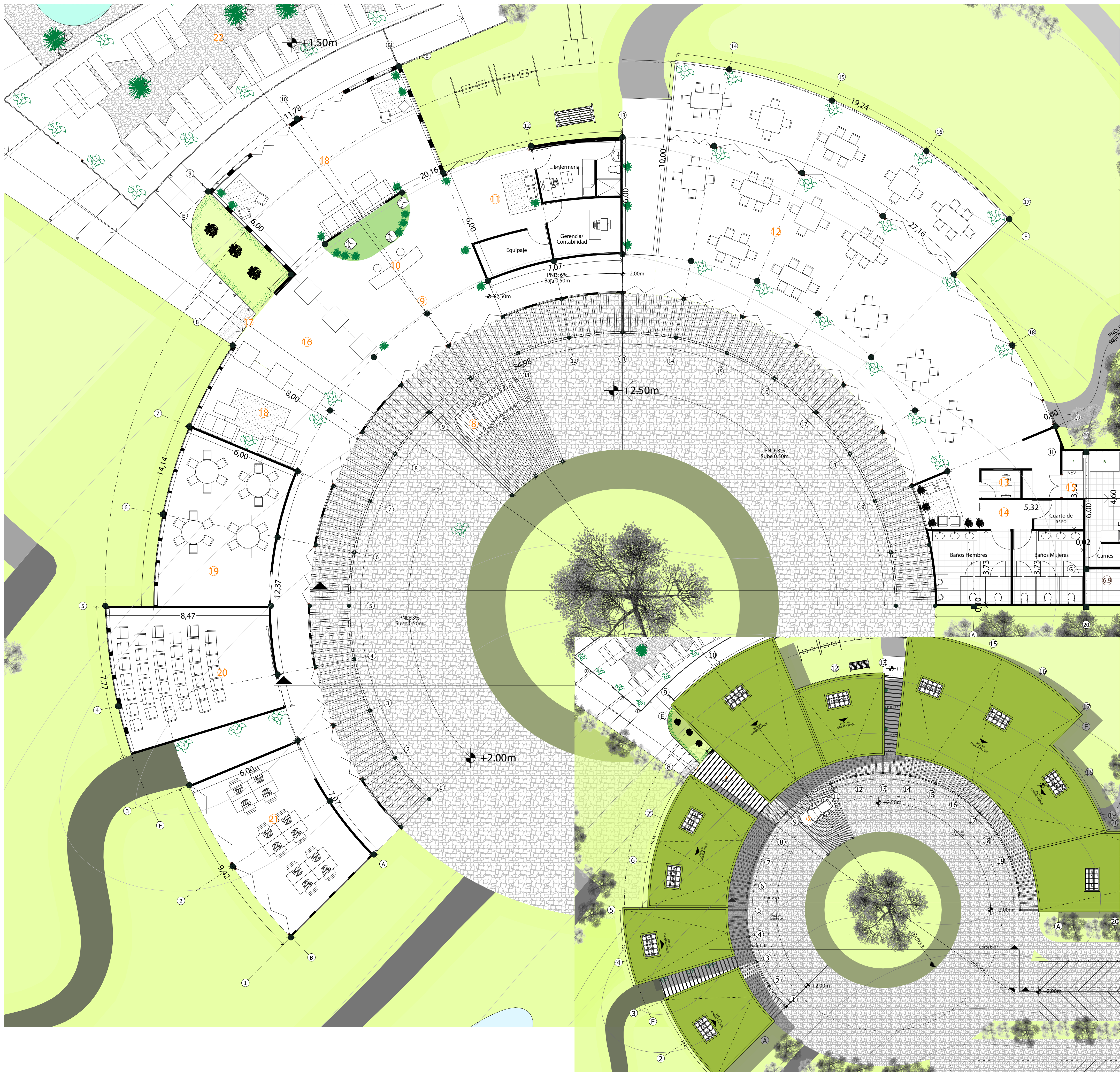
PLANTA ARQUITECTONICA ZONA MODULO PRINCIPAL
