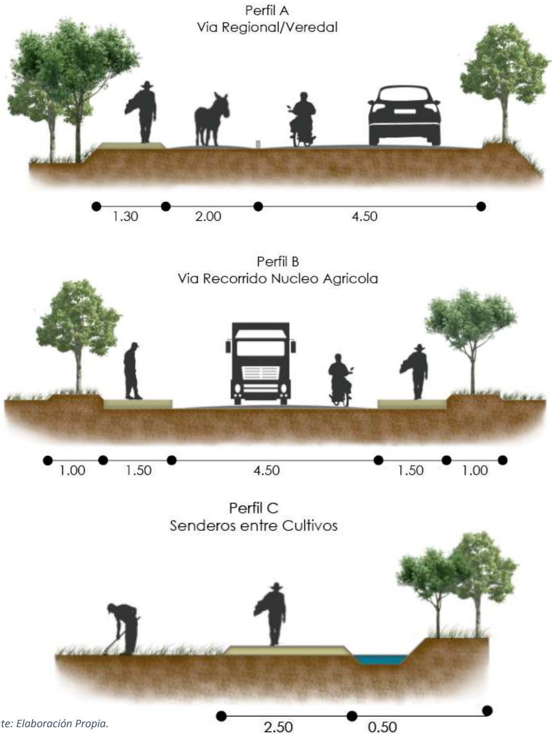
Ilustración 40 Perfiles Viales Propuestos
