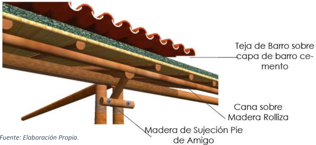
Ilustración 55 Cubierta
