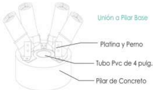
Ilustración 57 Unión a Pilar Base
