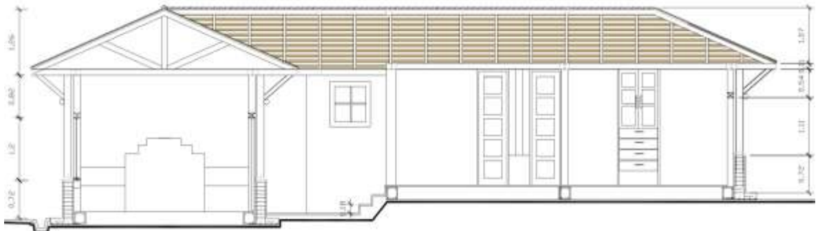
Ilustración 54 Corte Longitudinal Vivienda Digna.
