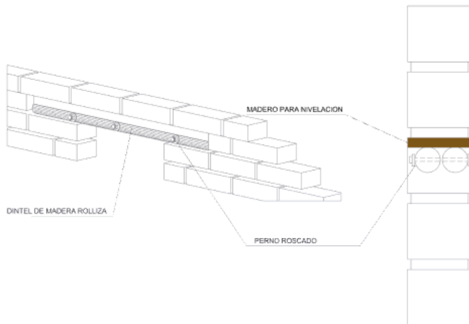
Ilustración 59 Detalle Dintel Típico
