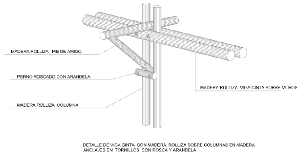
Ilustración 58 Detalle Viga Cinta
