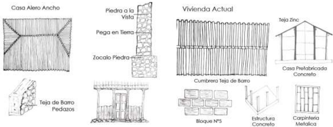
Ilustración 24 Casa Alero Ancho-Vivienda Actual.
