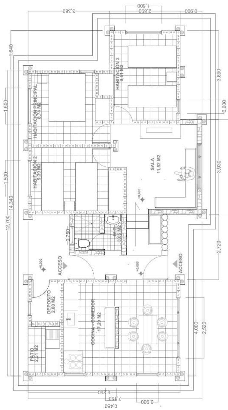
Ilustración 50 Planta Vivienda Digna.
