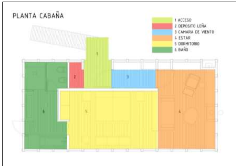
Figura 14. Planta de cabañas del hotel Awasi
