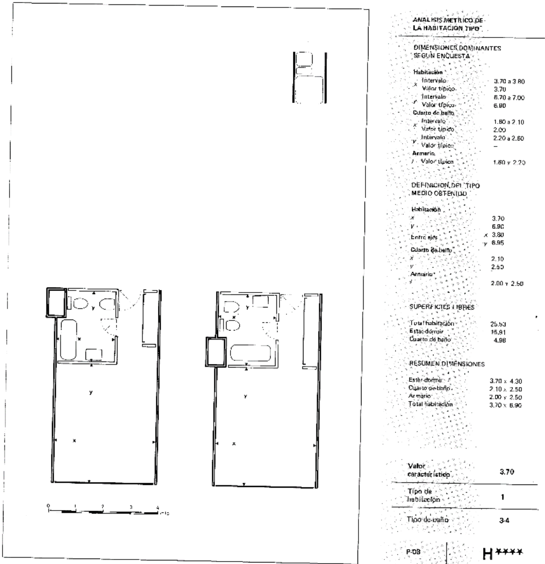
Figura 9. Organización de habitación estandarizada de hotel
