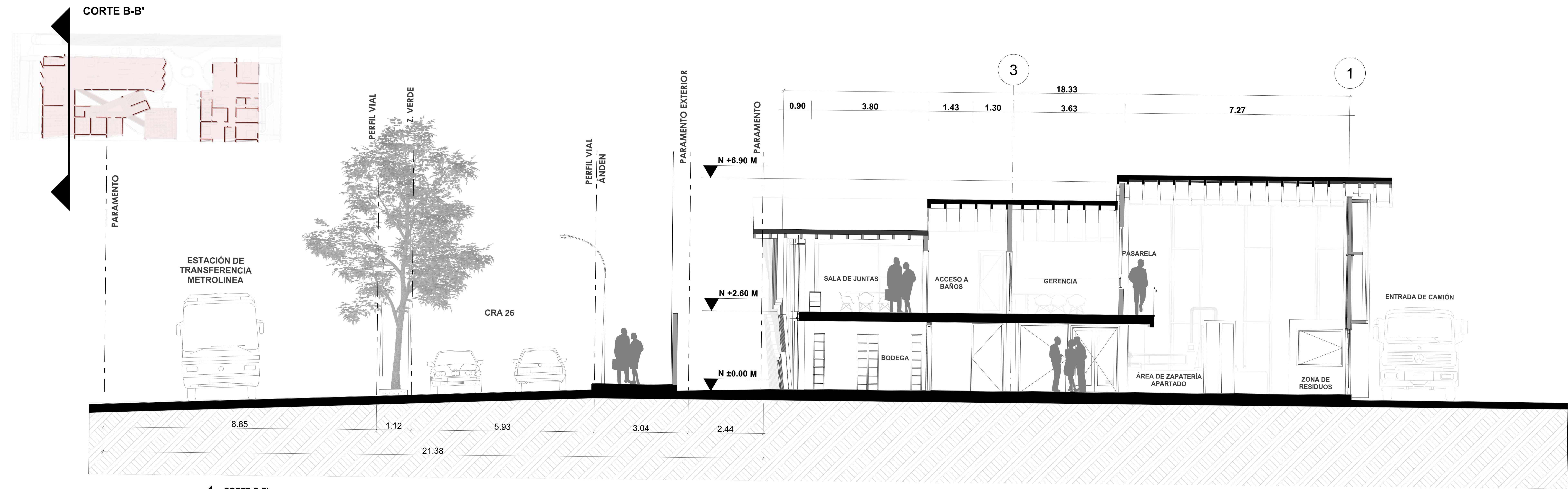
CORTE TRANSVERSAL B-B - ZONA INDUSTRIAL ESC 1:50
