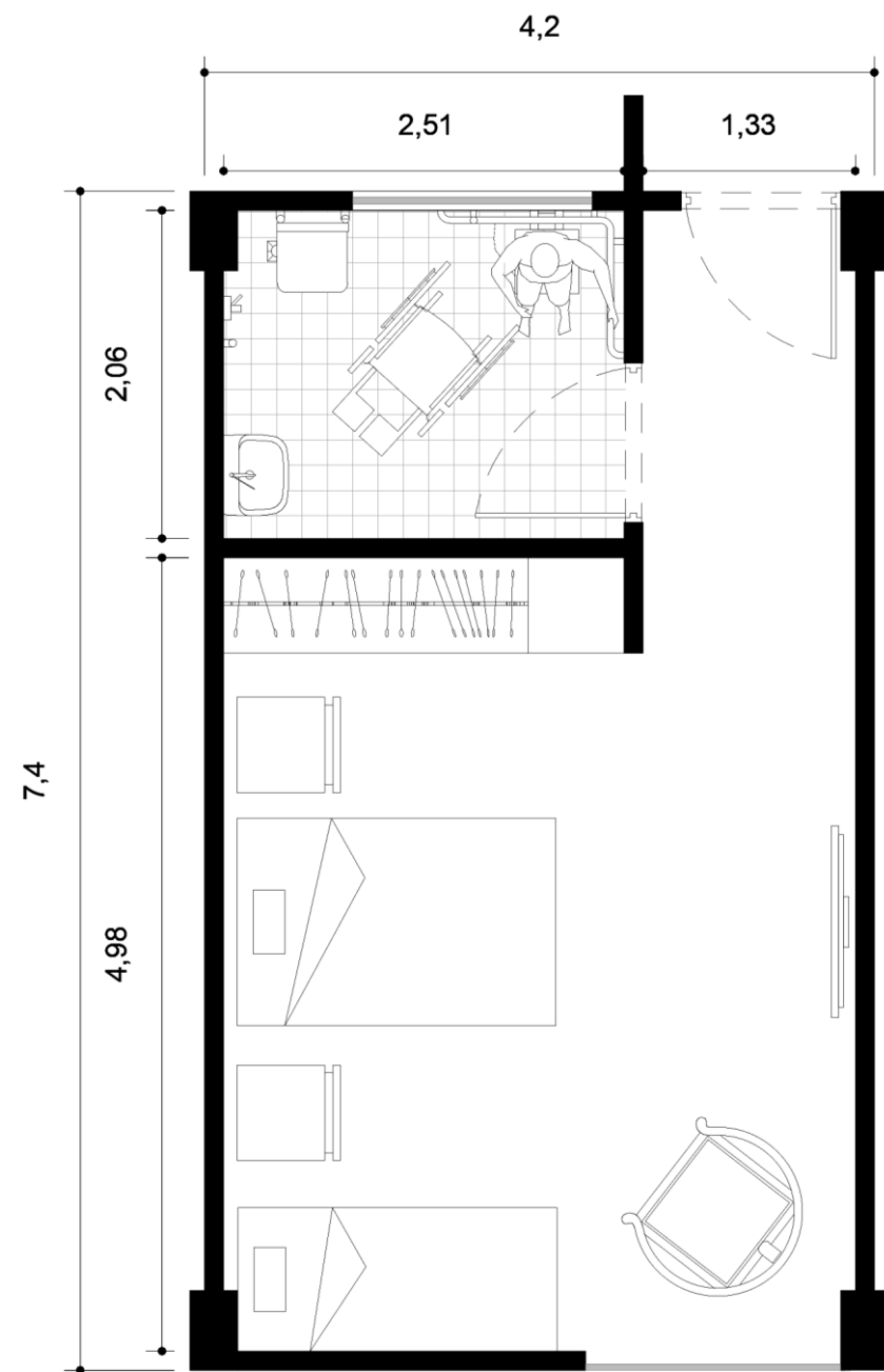
Planta alcoba tipo 1 ESC 1:50
