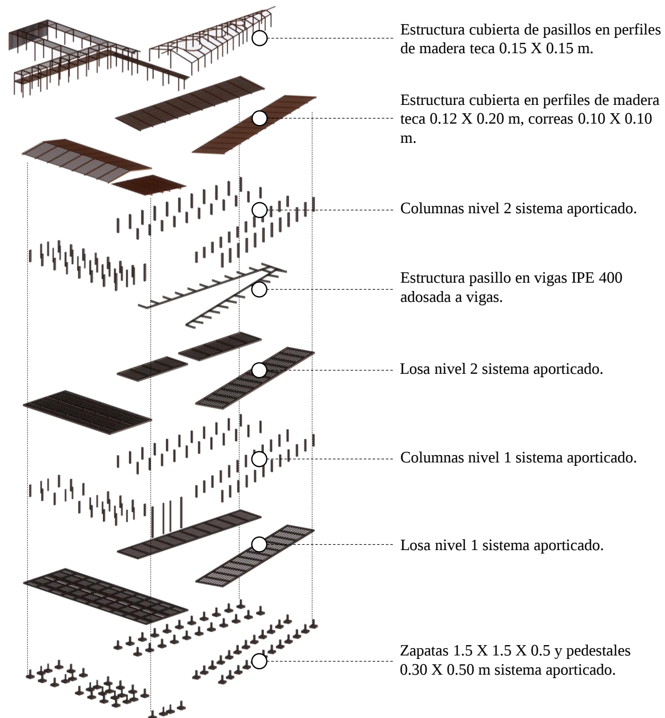
Fig. 53 Isométrico sistema estructural explotado. Juan F. Guerrero. 2022
