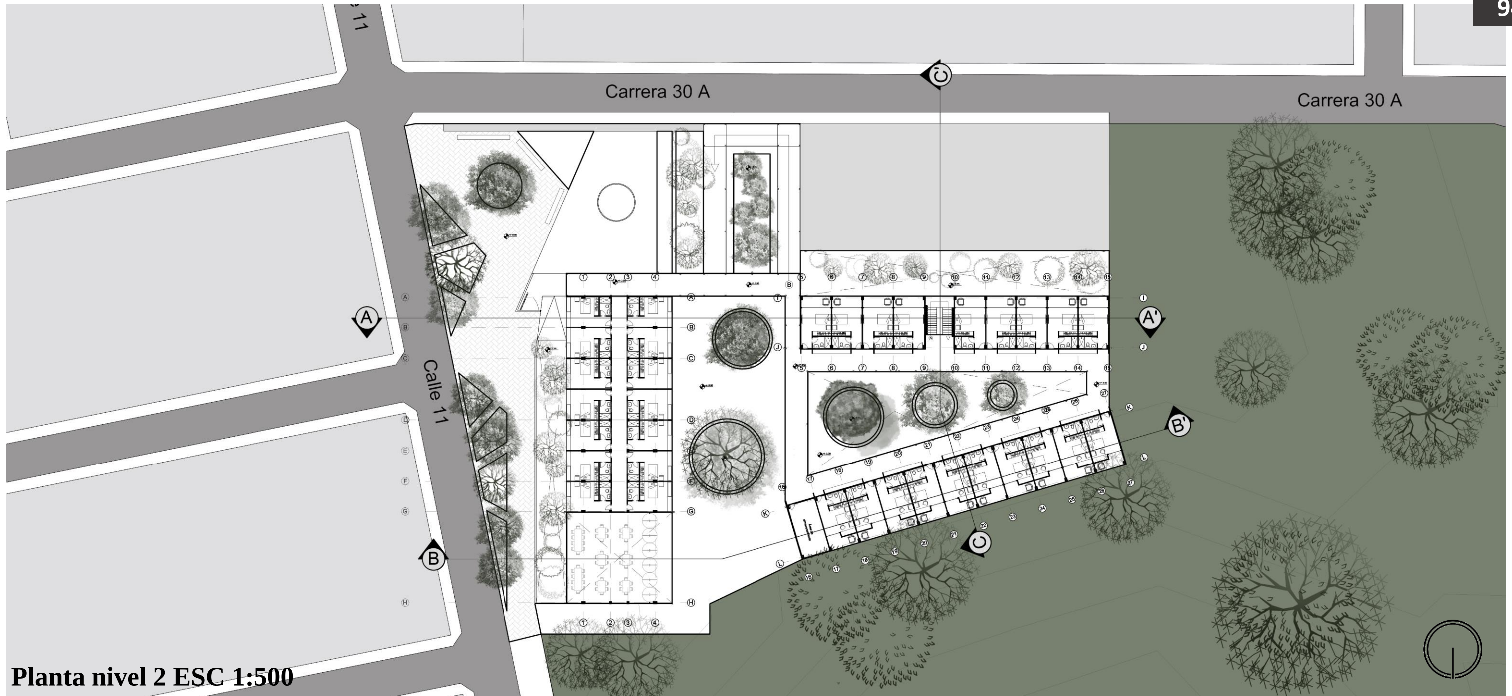
Fig. 64 Planta segundo nivel
