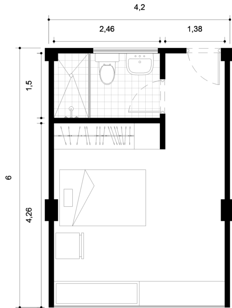
Planta alcoba tipo 1 ESC 1:50
