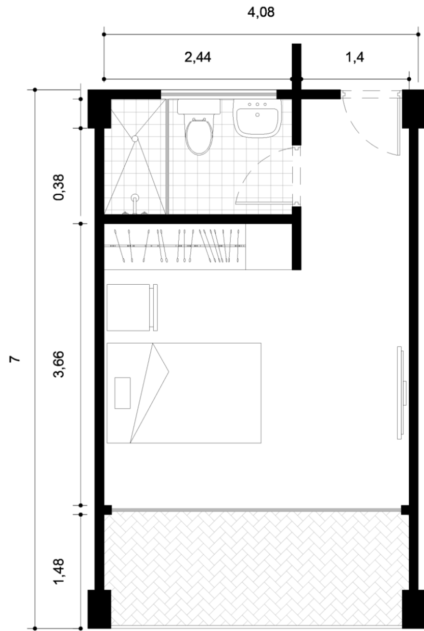
Planta alcoba tipo 1 ESC 1:50
