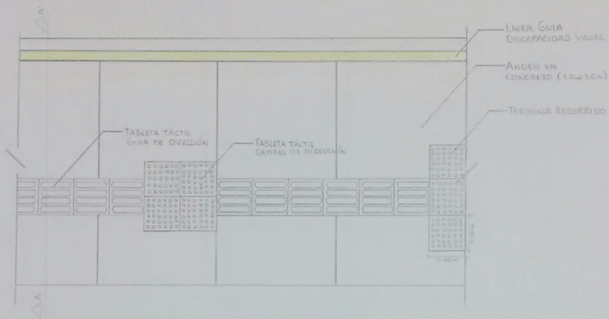
DETALLE ANDEN DISCAPACIDAD ESC. 1:20
