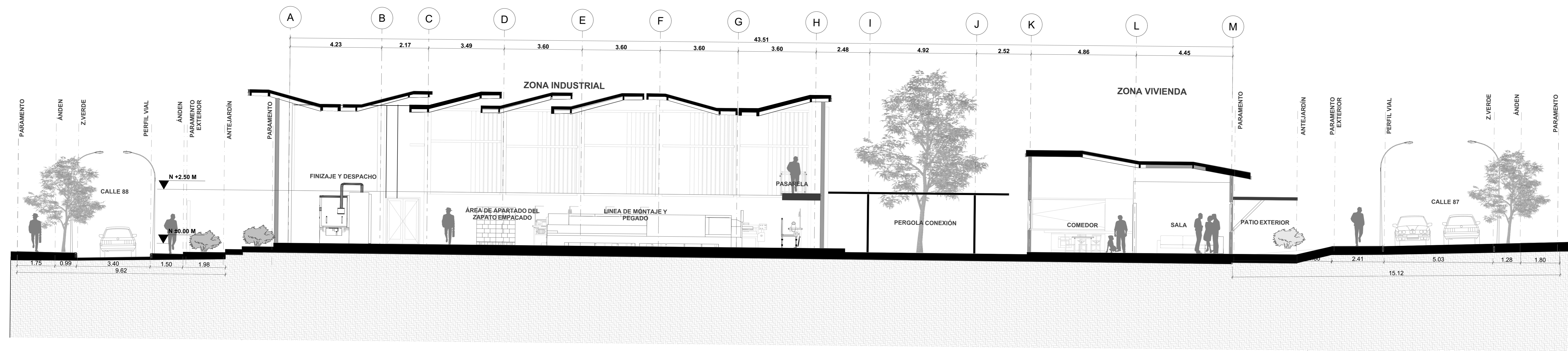
CORTE LONGITUDINAL A-A - CASA HUELLA ESC 1:75
