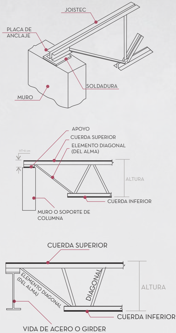
Figura 65, Detalles estructurales Elaboración propia.
