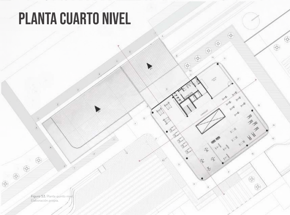
Figura 52, Planta cuarto nivel, Elaboración propia.
