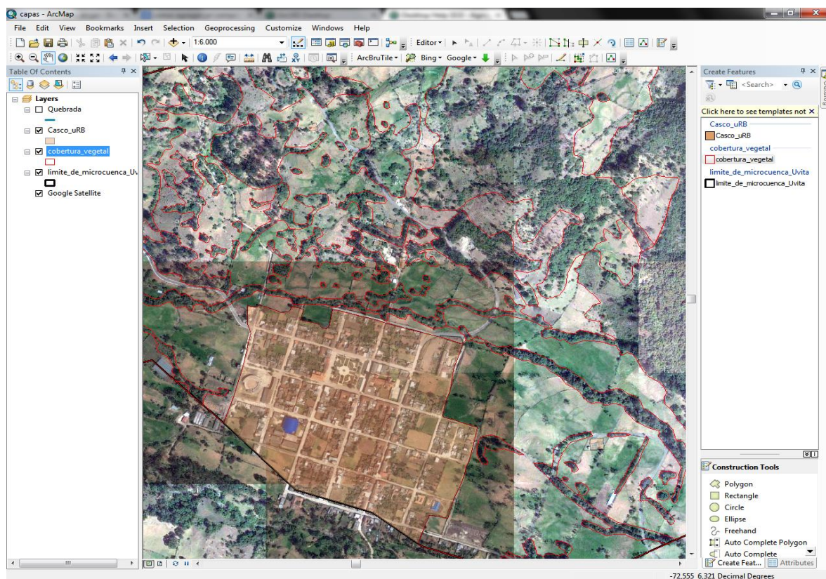
Imagen 18. Digitalización de la estructura ecológica del límite de la microcuenca Quebrada Negra.
