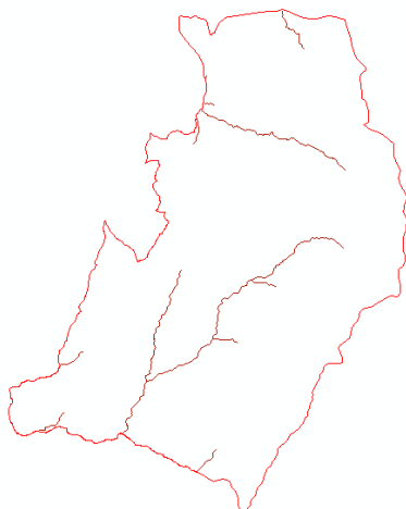
Imagen 13. Drenajes del municipio de La Uvita.
