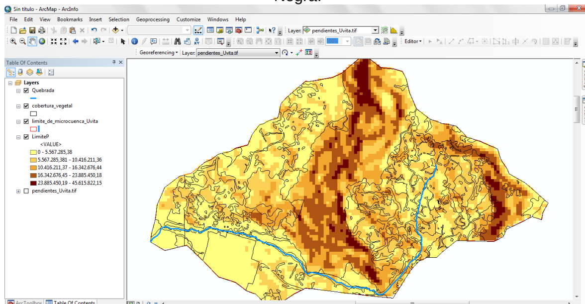
Imagen 19. Generación del mapa de pendientes de la microcuenca Quebrada Negra.
