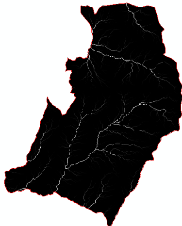
Imagen 15. Zonas de acumulación del municipio de La Uvita
