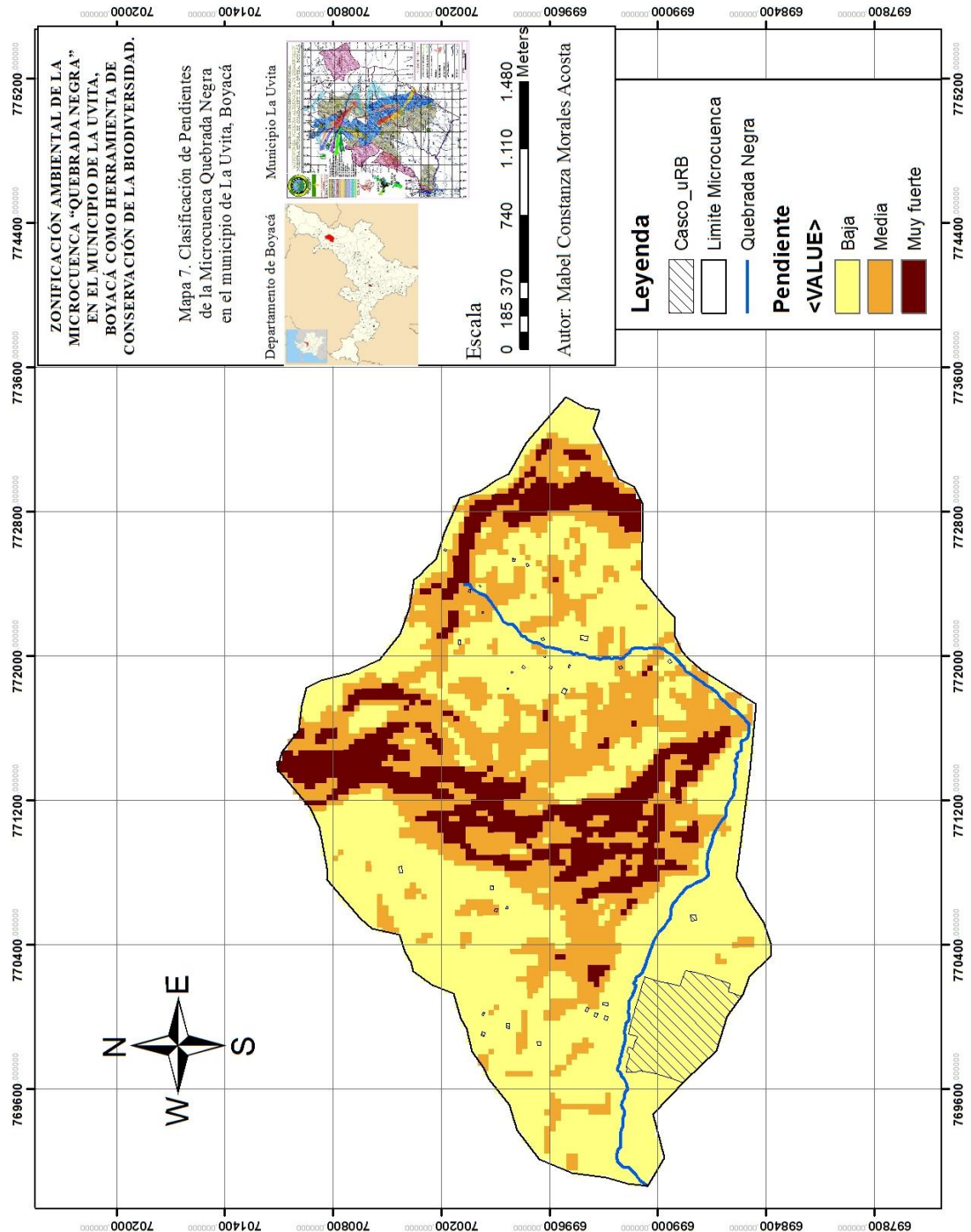
Mapa 8. Mapa de pendientes de la Microcuenca Quebrada Negra.
