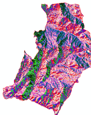
Imagen 16. Dirección del drenaje del municipio de La Uvita
