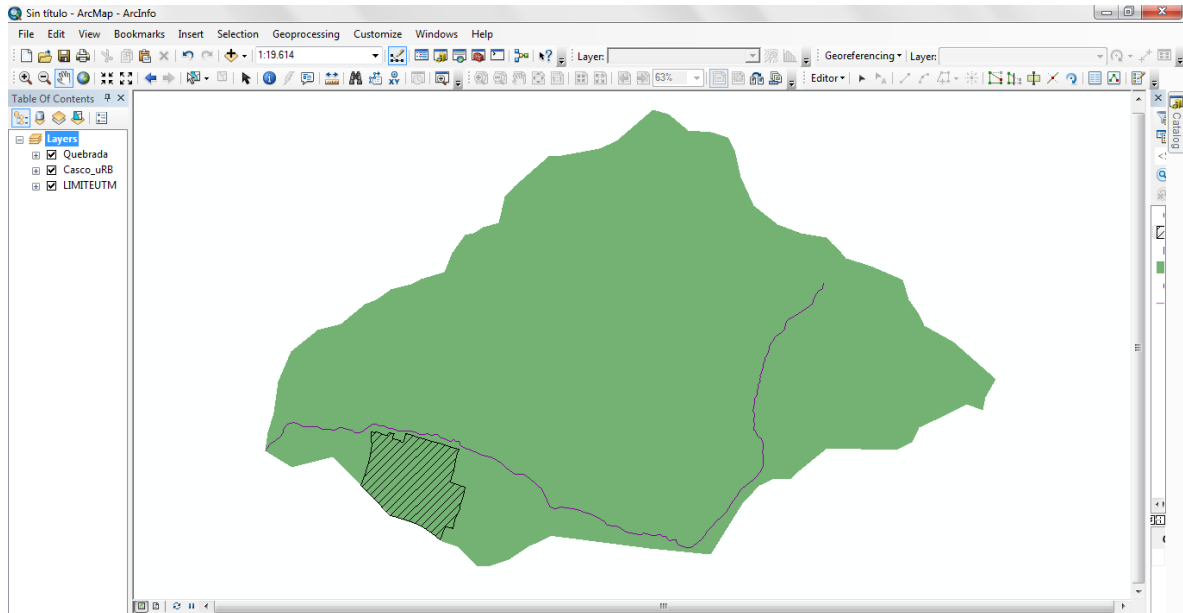
Imagen 17. Definición del límite de la microcuenca Quebrada Negra.
