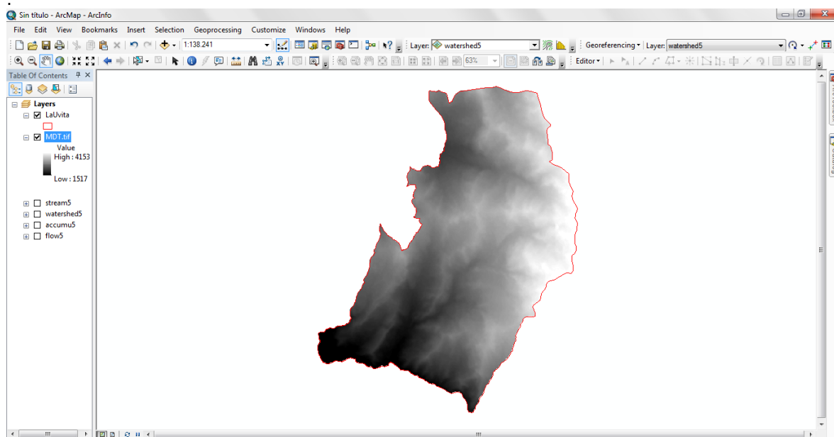
Imagen 12. Modelo Digital del Terreno (MDT) del municipio de La Uvita
