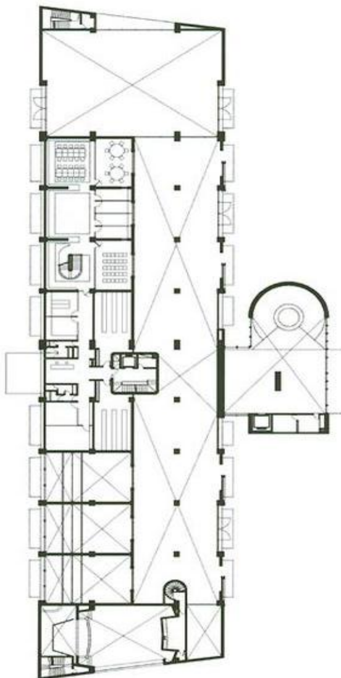
Imagen 12. Planta Mezzanine.
