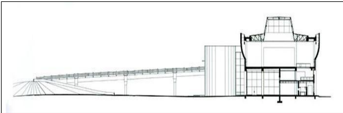
Imagen 15. Corte transversal.
