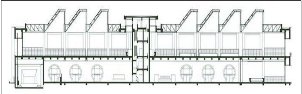
Imagen 14. Corte longitudinal.
