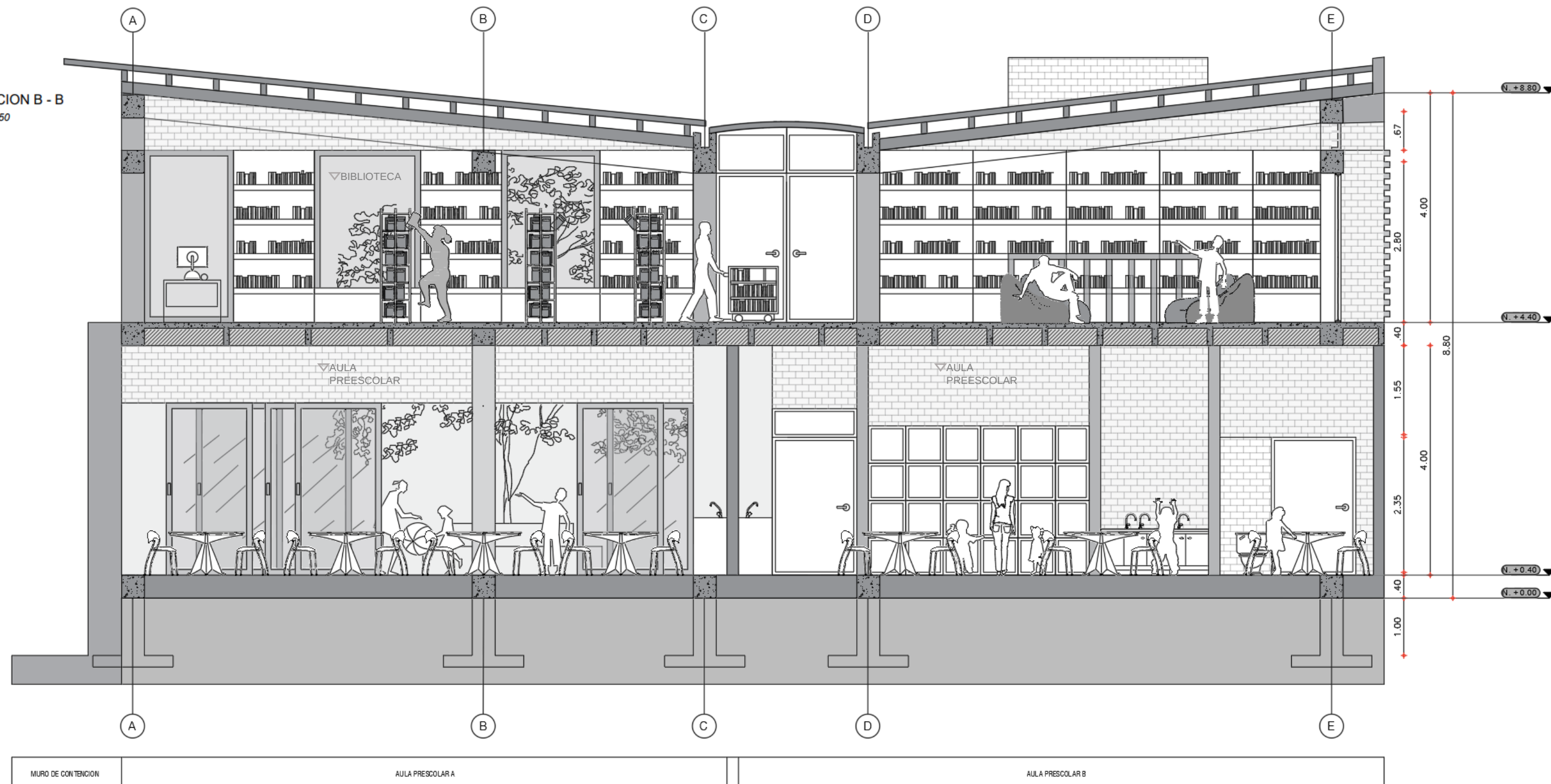
▲ Figura 73 – López, D. A. (2021). Sección B-B colegio nuevo comienzo. [Imagen].
