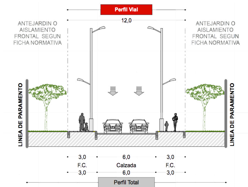
Figura 32. Perfil Vial 12.00 mts, Tipo C – POT
