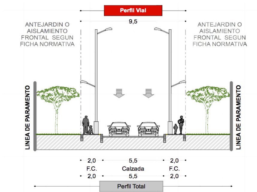
Figura 31. Perfil Vial 9.50 mts, Tipo A – POT
