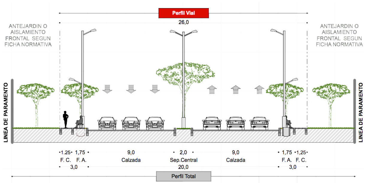
Figura 33. Perfil Vial 26.00 mts, Tipo A – POT
