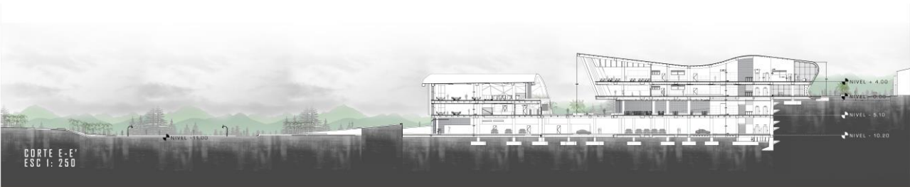
CORTE E-E'
