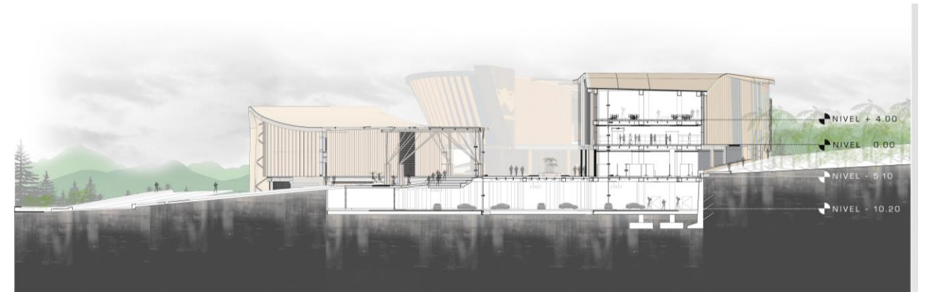
CORTE C-C'
