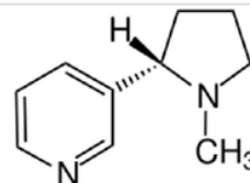
Figura 3. Nicotina
