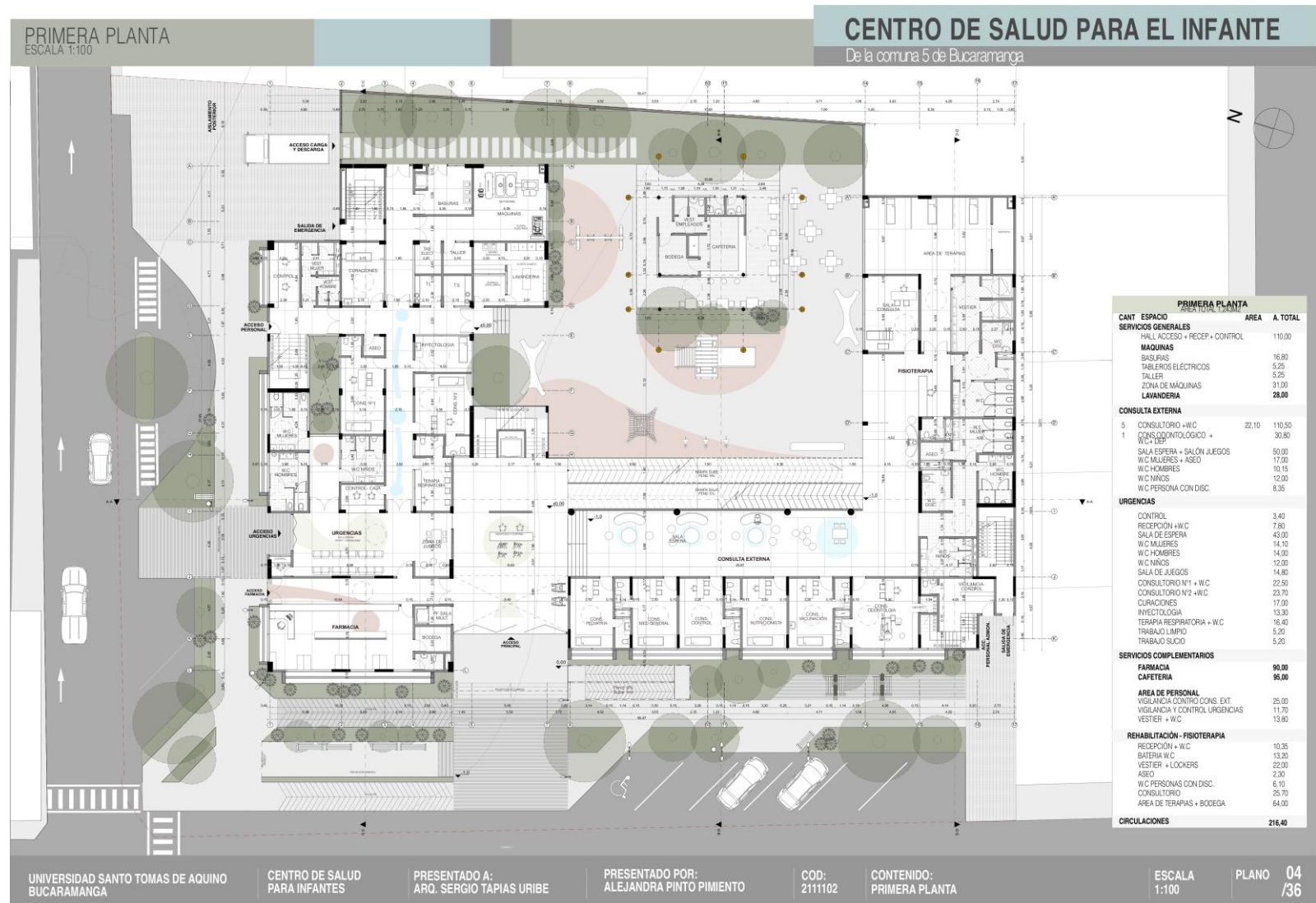
Figura 95. Primera planta.
