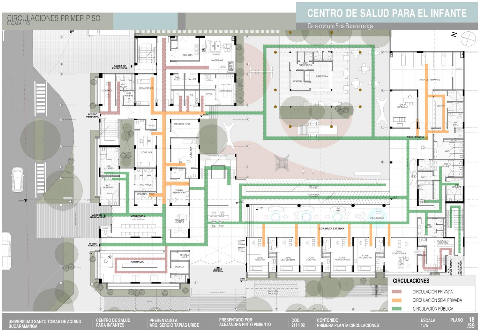
Figura 109. Plano de circulaciones del primero piso.
