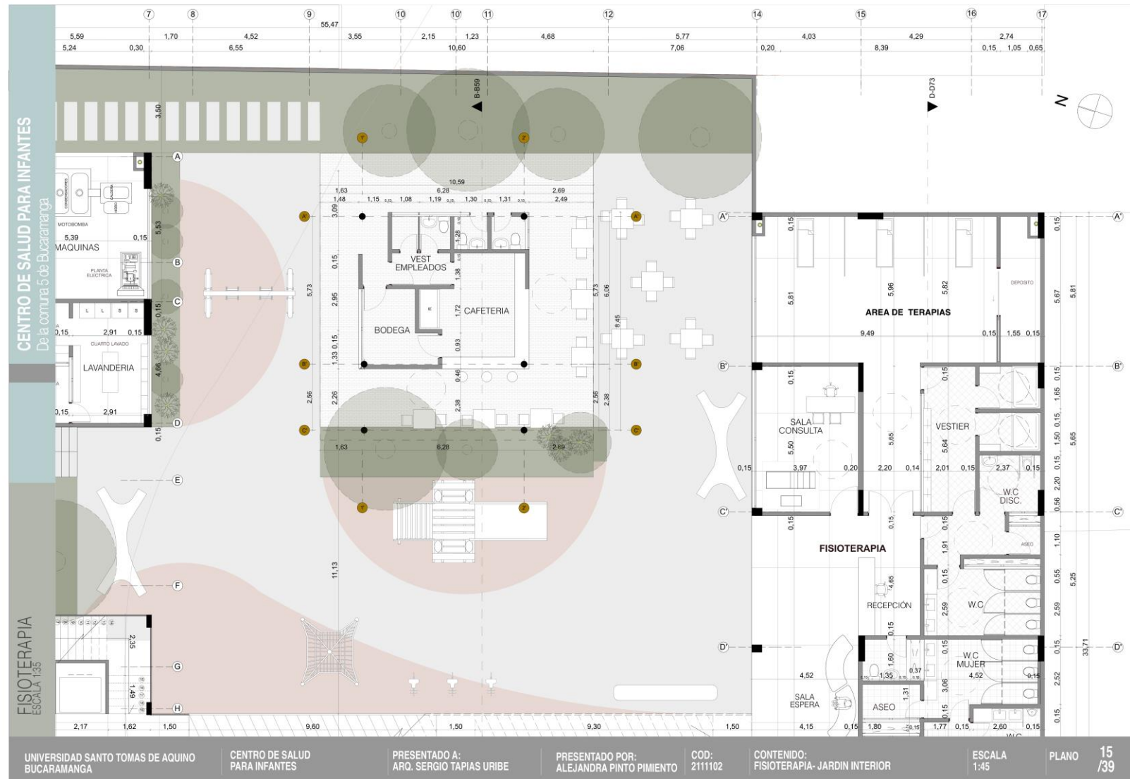
Figura 106. Ampliación fisioterapia.
