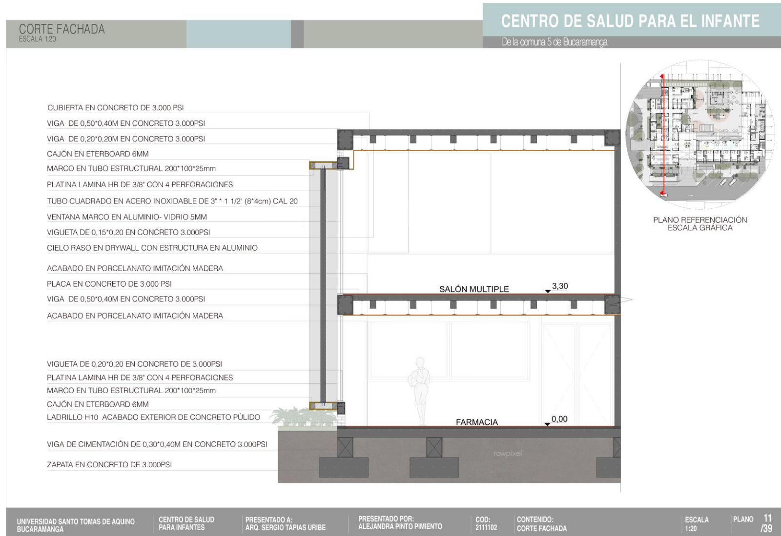
Figura 102. Corte fachada.
