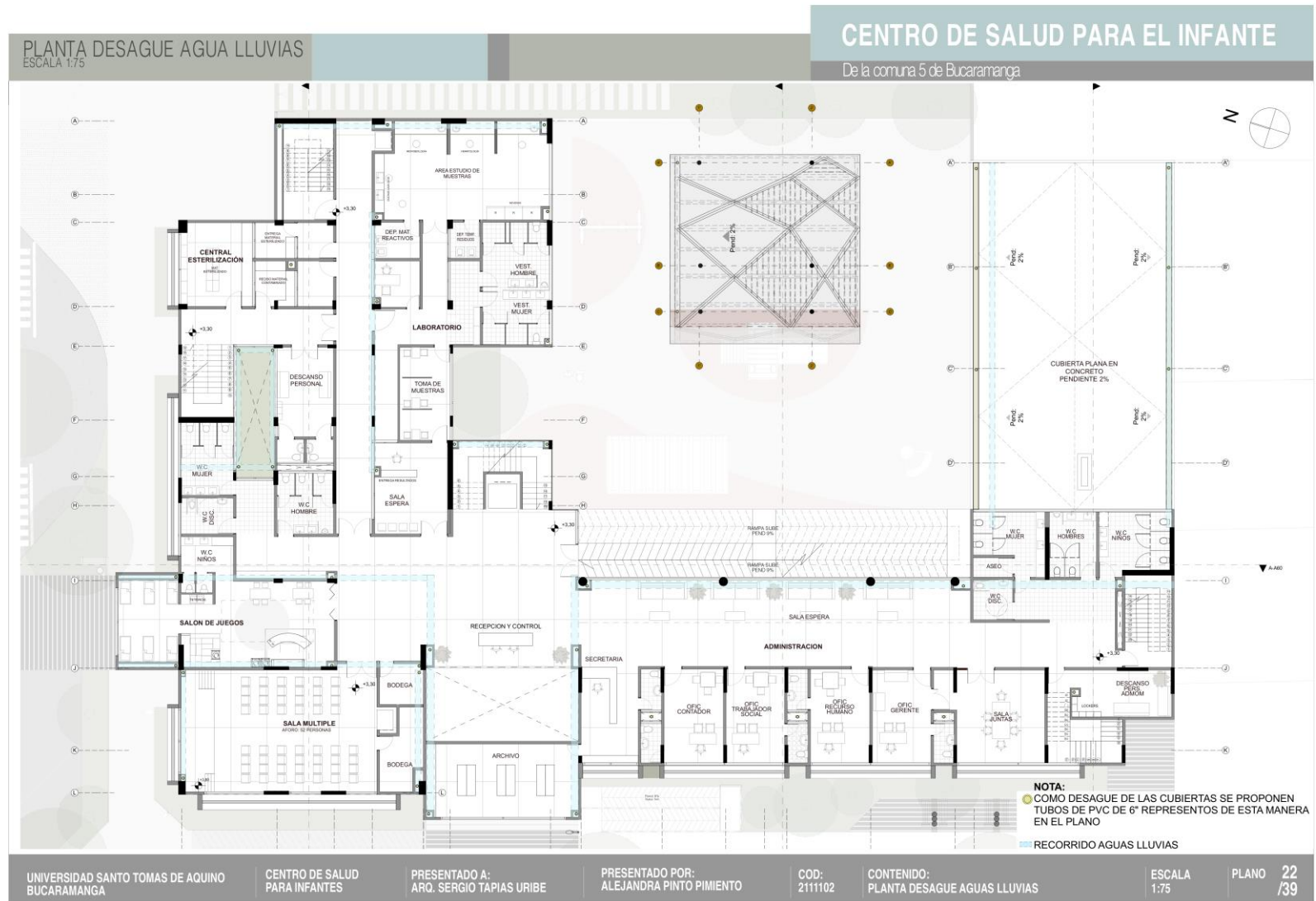
Figura 113. Plano de desagües de agua lluvia.
