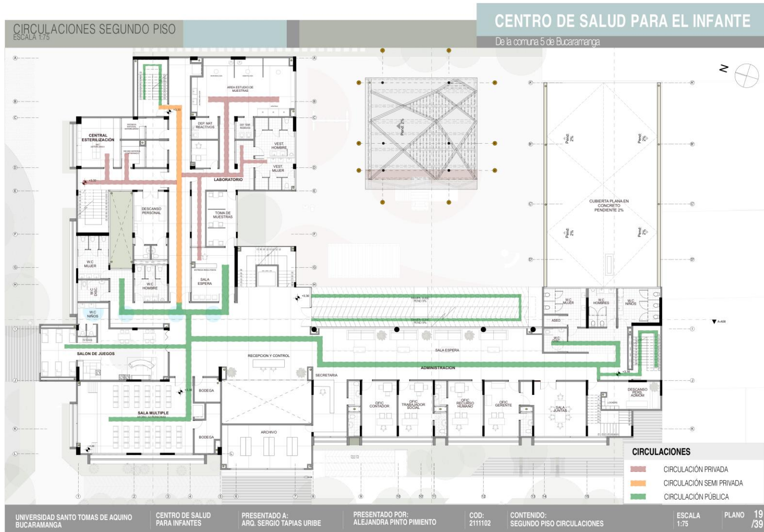
Figura 110. Plano de circulaciones del segundo piso.
