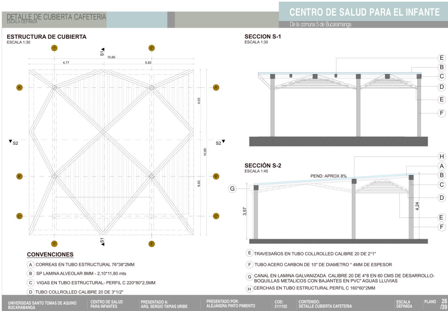
Figura 119. Detalle de cubierta de cafetería.
