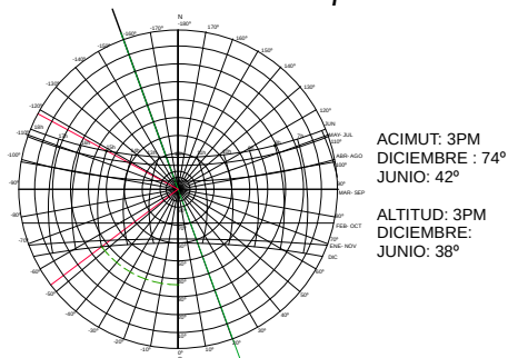
Figura 12. Carta solar latitud 7° fachada 4- Occidente.
