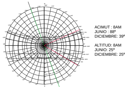
Figura 10. Carta sola latitud 7° 2- Oriente.
