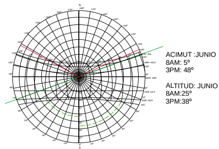
Figura 9. Carta solar, latitud 7° Fachada 1- Norte.
