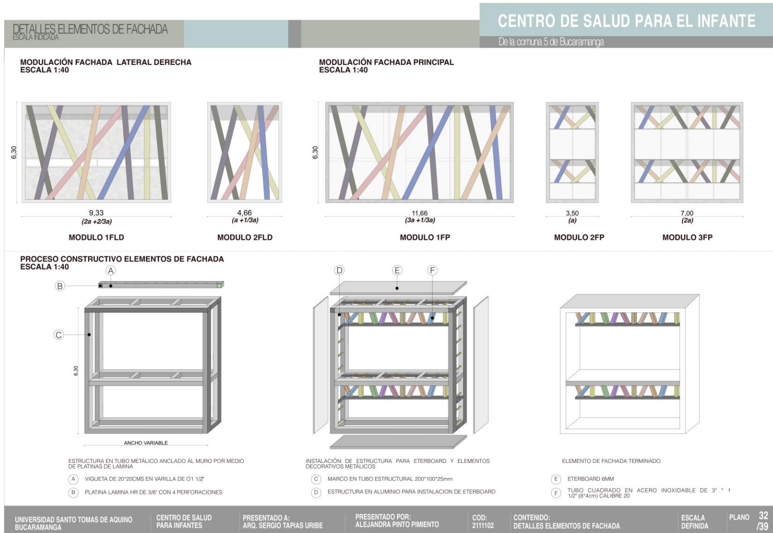
Figura 123. Detalle de fachada.
