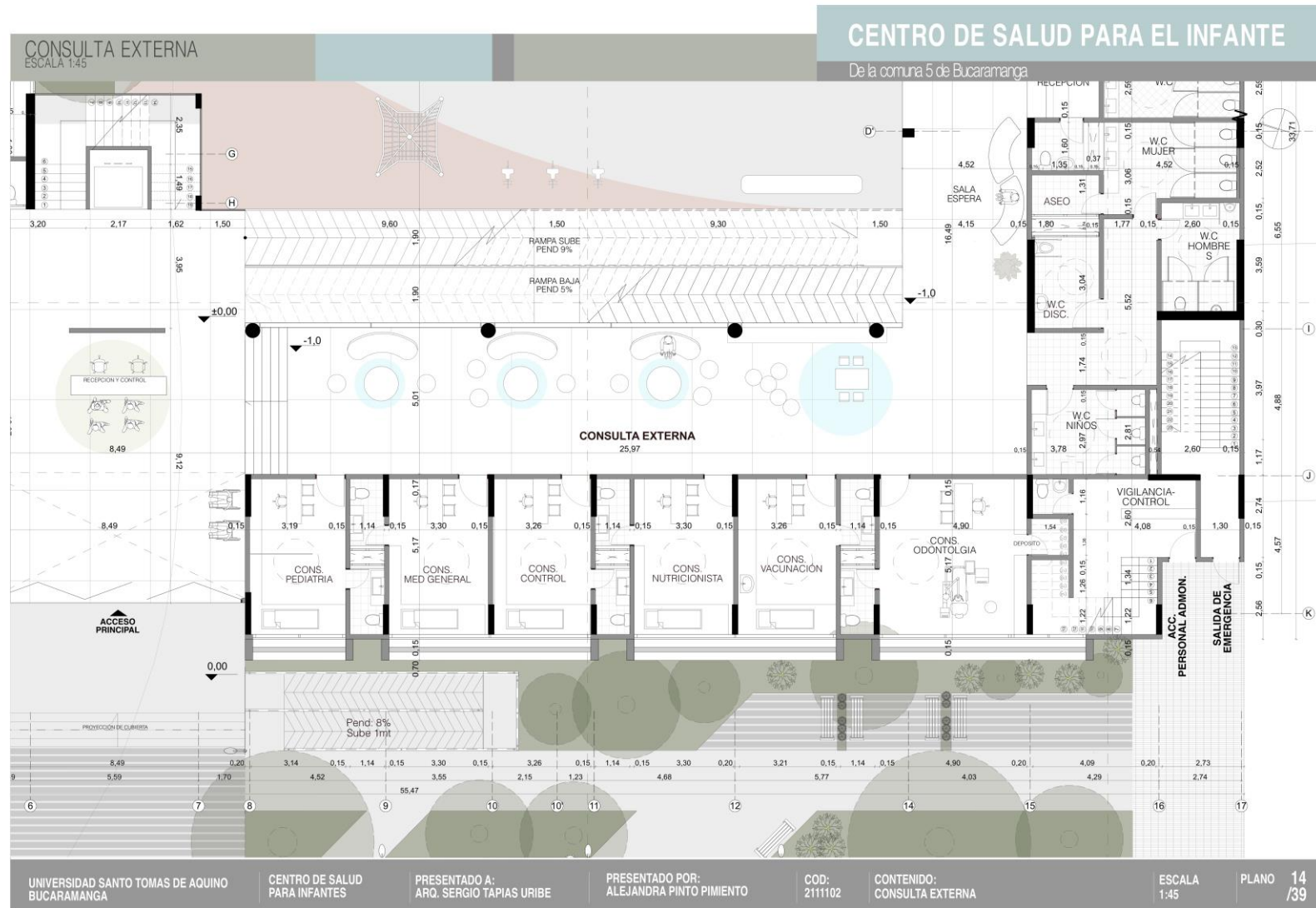
Figura 105. Ampliación consulta externa.
