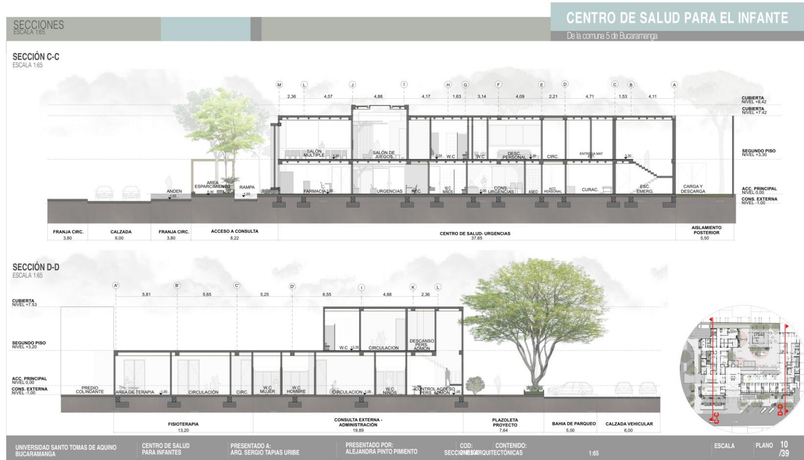
Figura 101. Secciones.
