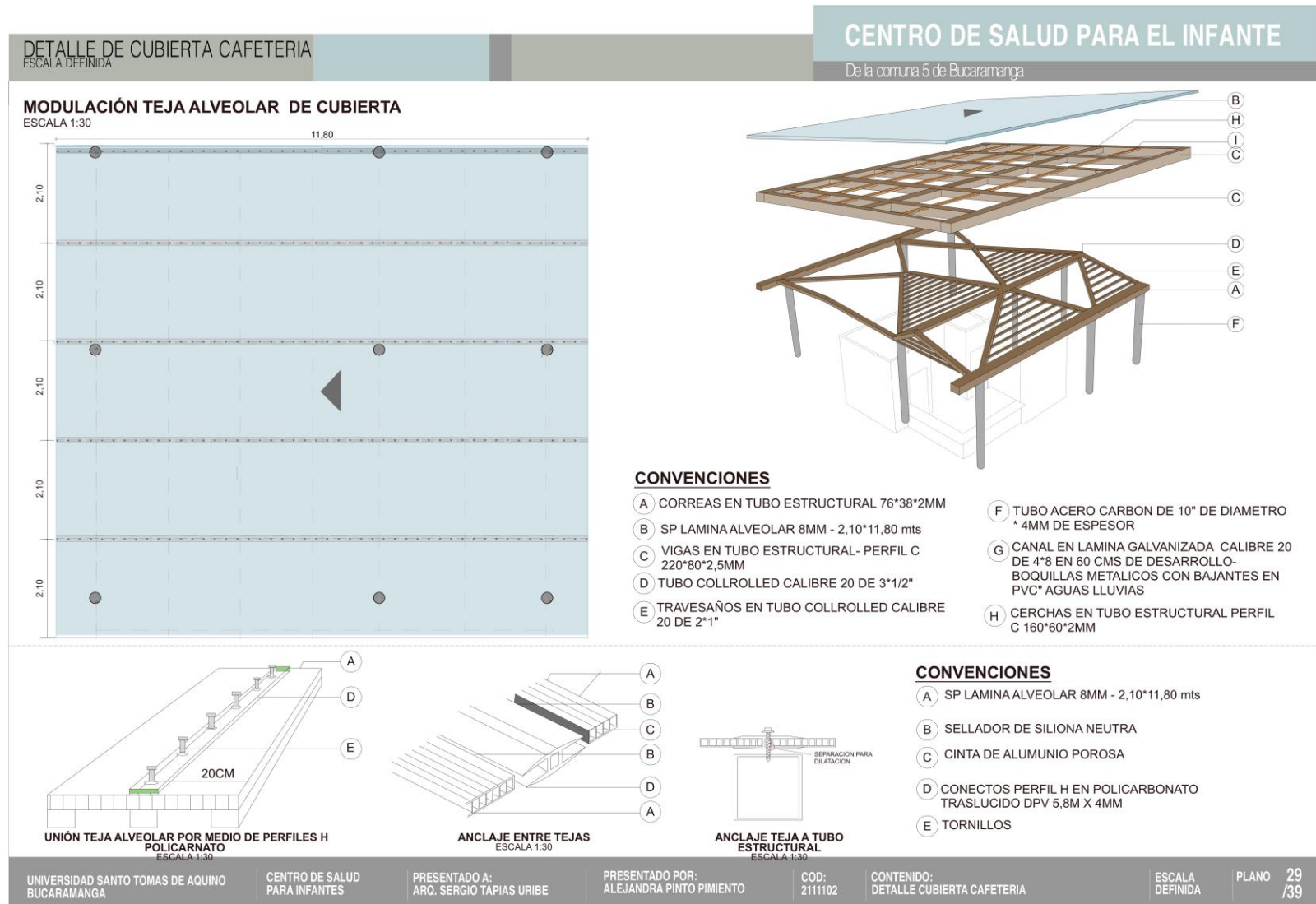
Figura 120. Detalle de cubierta de cafetería.
