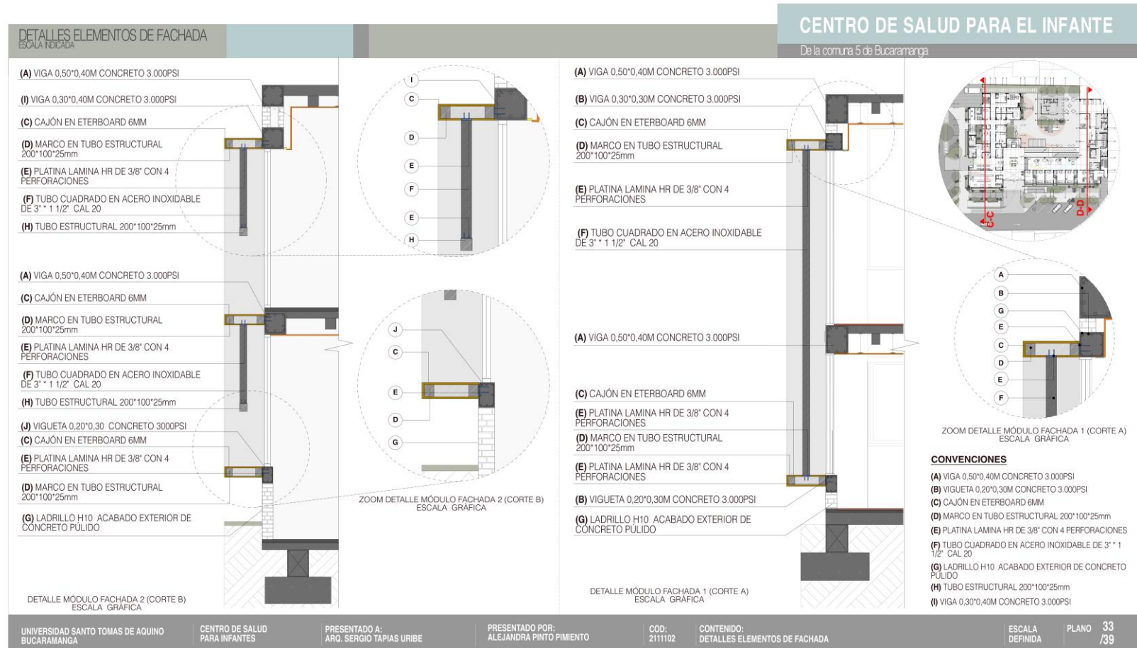
Figura 124. Detalle de fachada.
