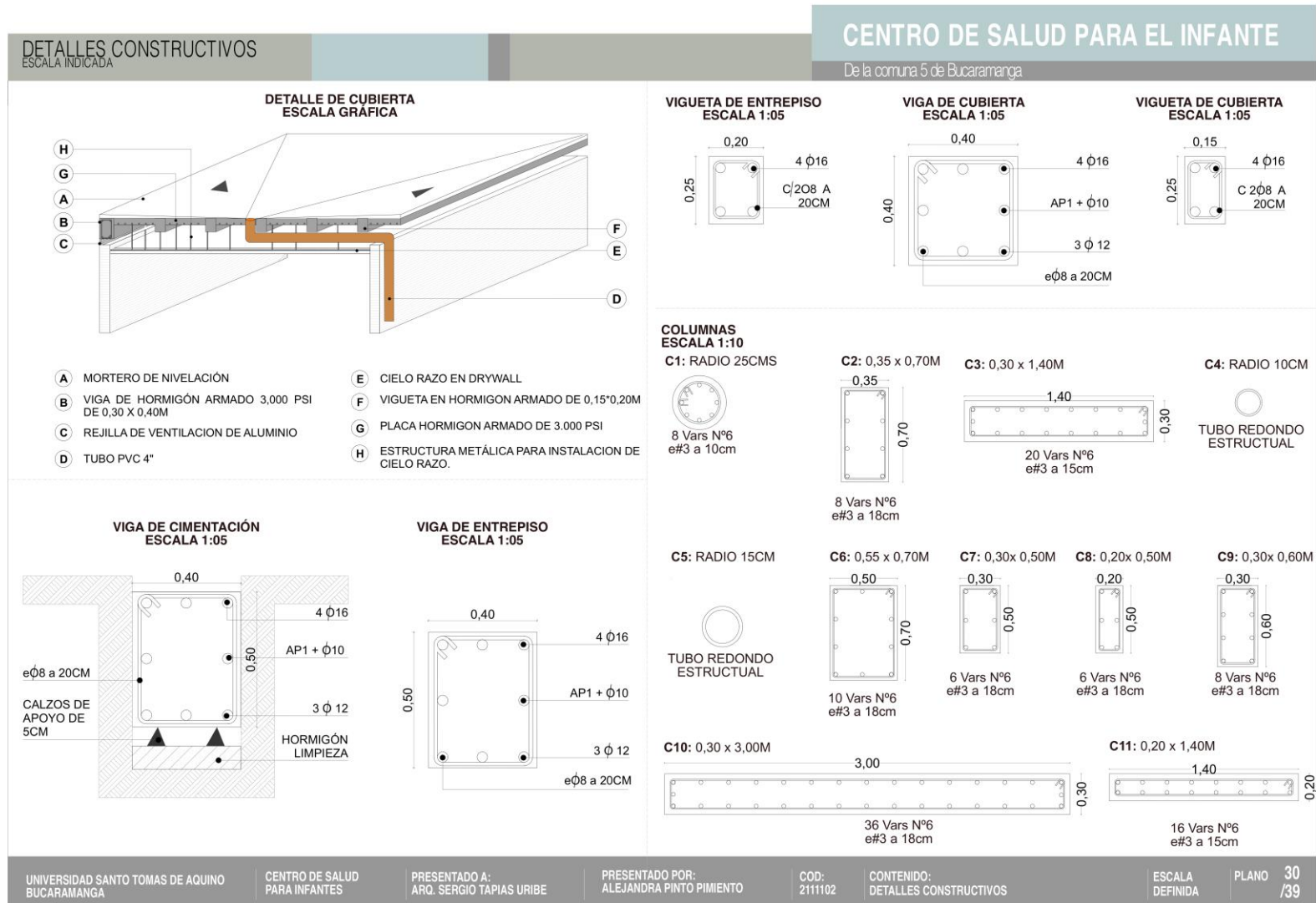
Figura 121. Detalles constructivos.
