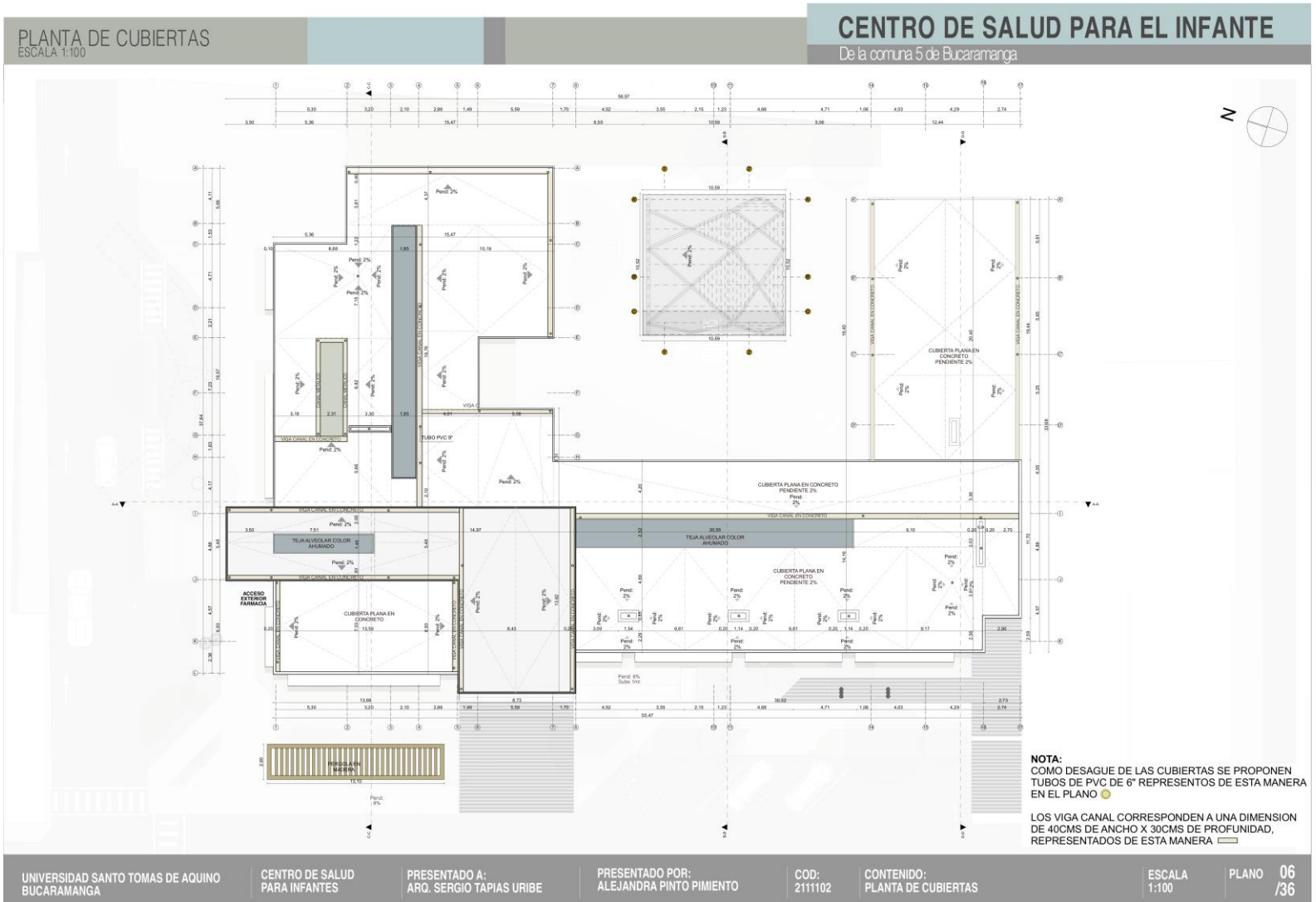
Figura 97. Planta de cubiertas.
