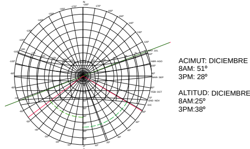
Figura 11. Carta Solar latitud 7° fachada 3- Sur.
