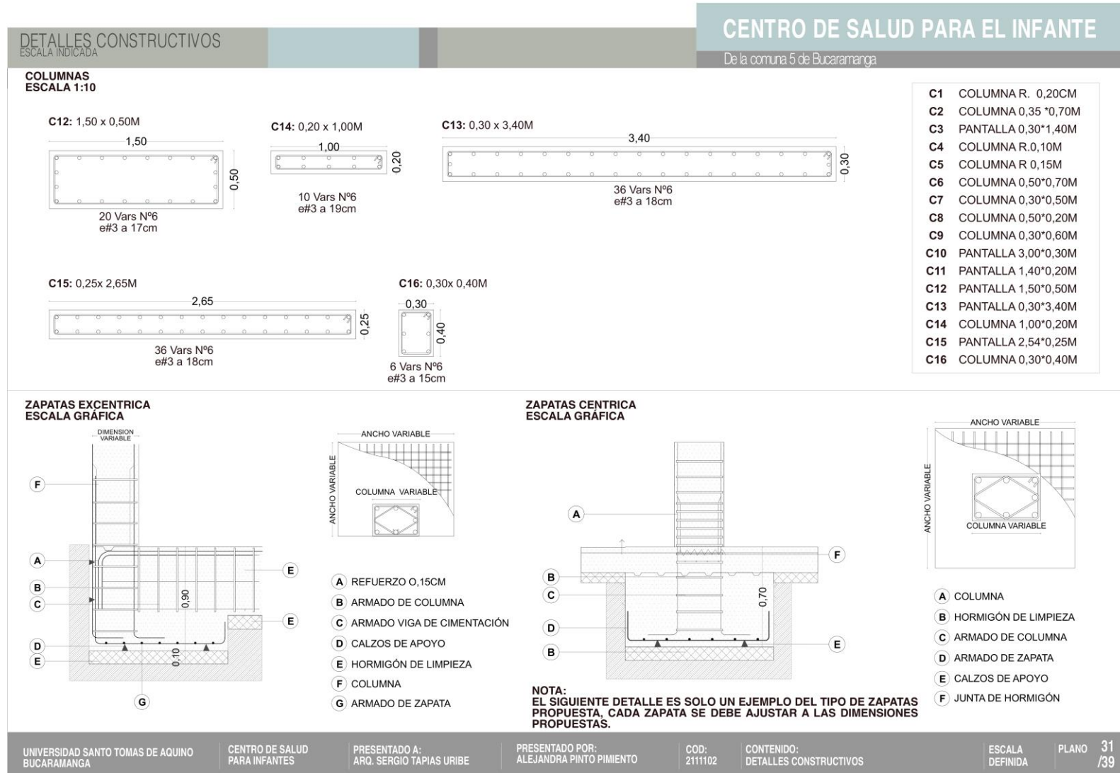
Figura 122. Detalles constructivos.
