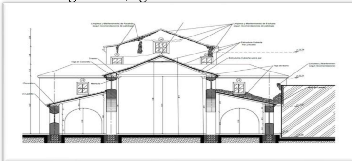
Imagen 2. Corte Longitudinal; Iglesia Santa Rita Casia
