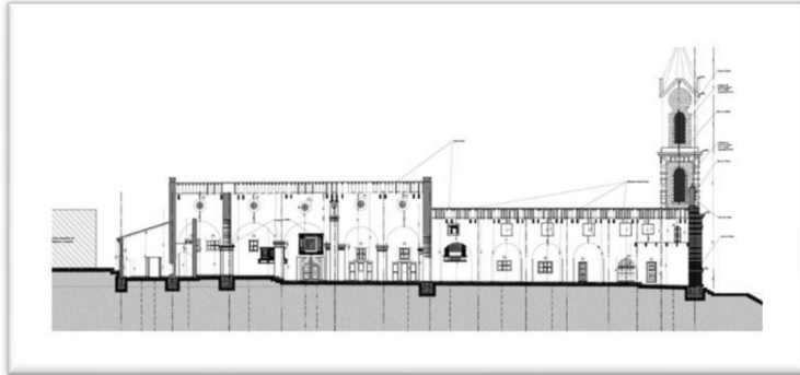
Imagen 1. Corte C; Iglesia Santa Rita Casia
