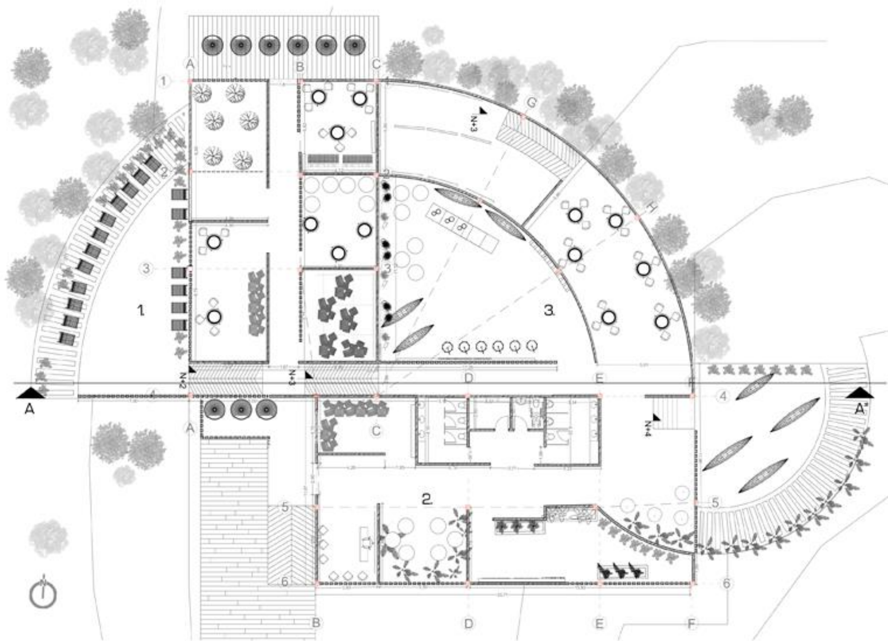
PLANTA
