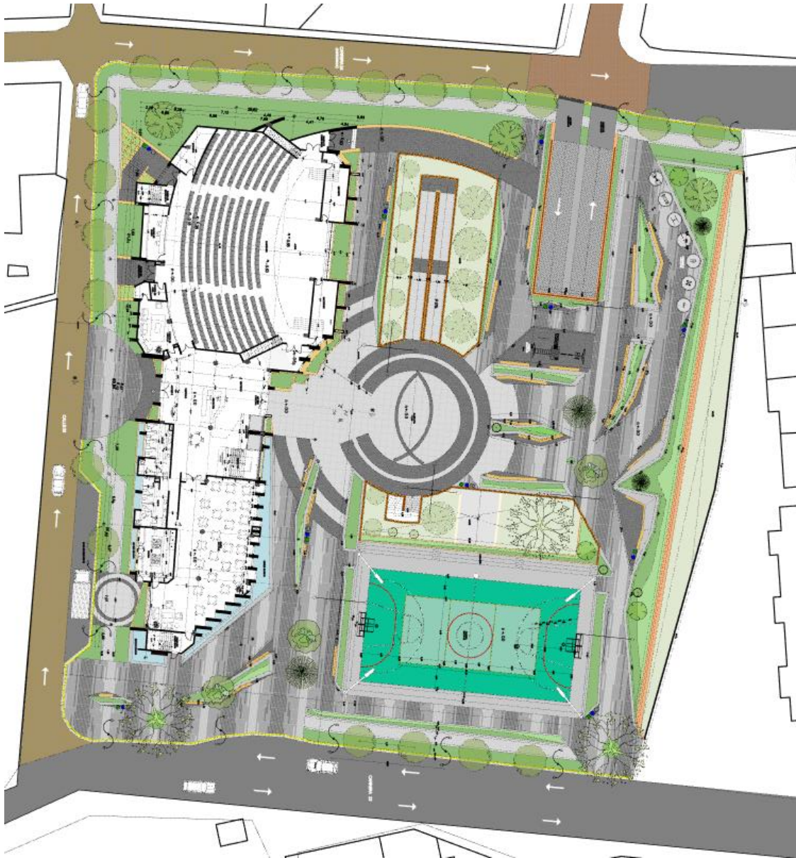
Figura 146. Planta Urbana, templo para mil quinientas personas en Girón, Santander, escala gráfica. Fuente propia.
