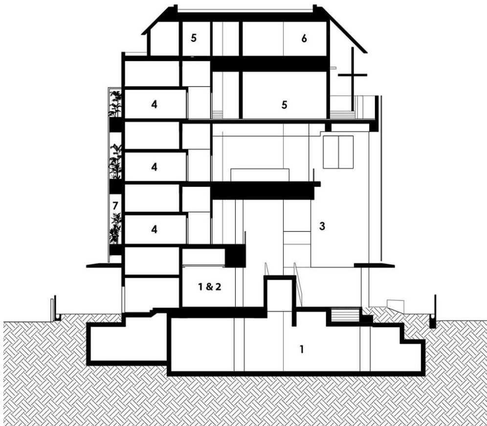
Figura 41. Corte perpendicular iglesia en Singapur Tomada de Plataforma de Arquitectura.
