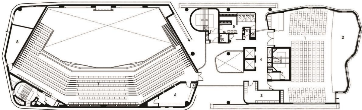
Figura 38. Planta tercer piso iglesia en Singapur Tomada de Plataforma de Arquitectura.
