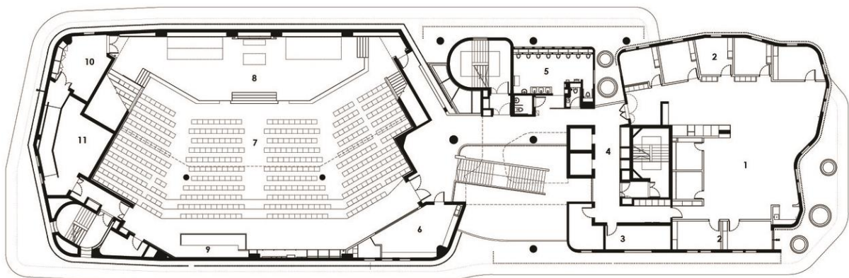
Figura 36. Planta segundo piso iglesia en Singapur Tomada de Plataforma de Arquitectura.
