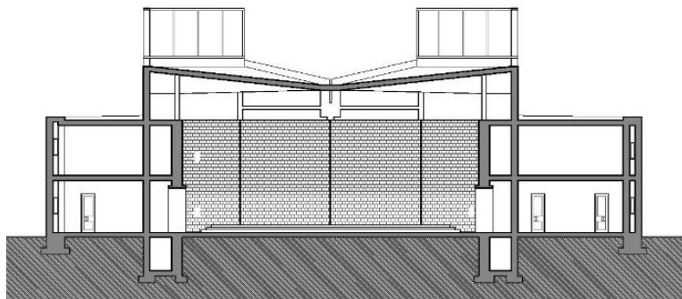
Figura 70. Corte B-B, iglesia en Rochester Tomada de Urbipedia.org, editada por el autor.
