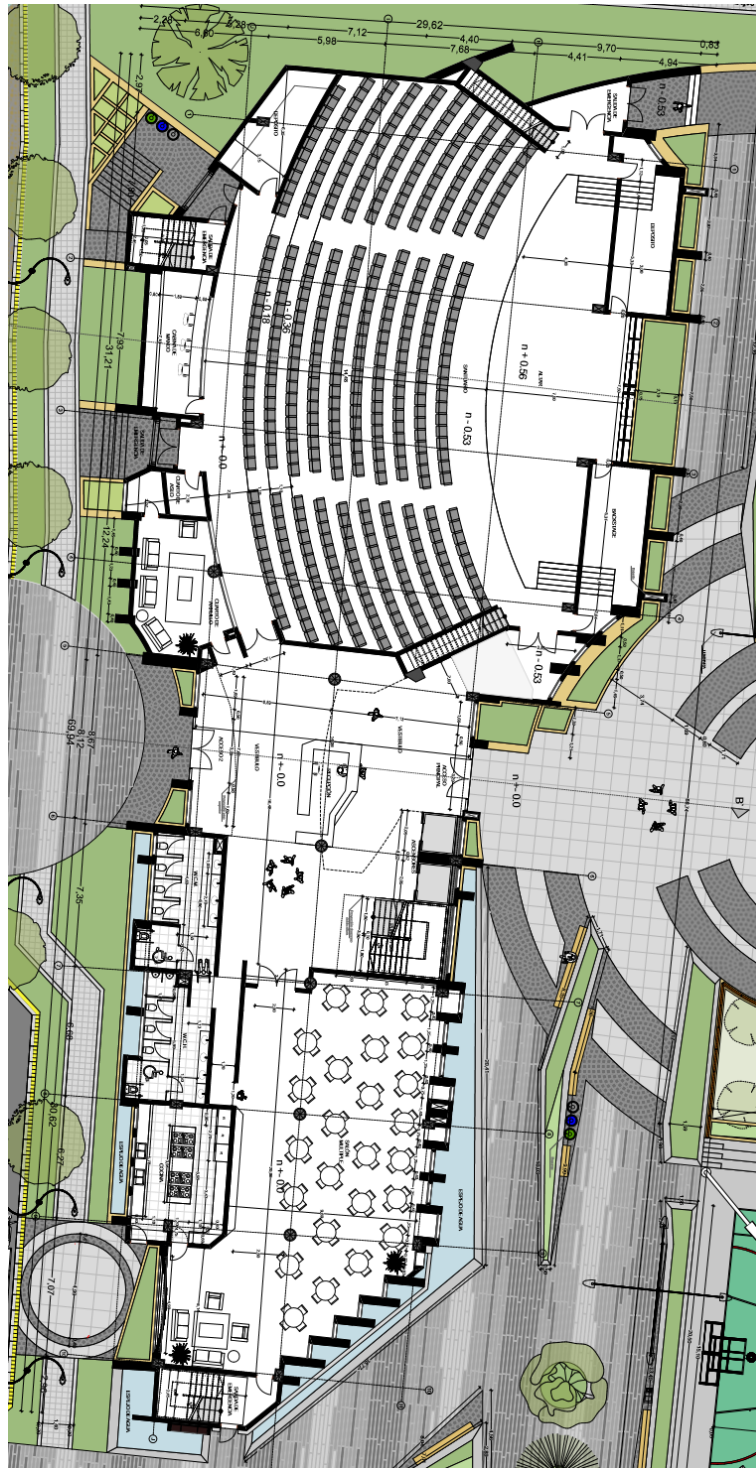
Figura 147. Planta Baja, templo para mil quinientas personas en Girón, Santander, escala gráfica. Fuente propia.
