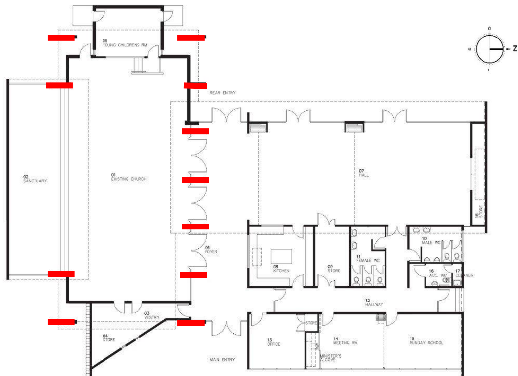
Figura 78. Análisis estructural templo en Wailuku Tomada de Plataforma de Arquitectura, editada por el autor.
