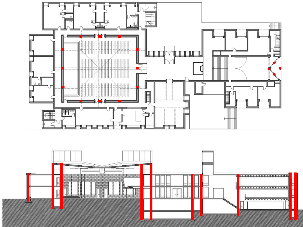
Figura 60. Análisis estructural templo unitario Tomada de Urbipedia. Org, Editada por el autor.
