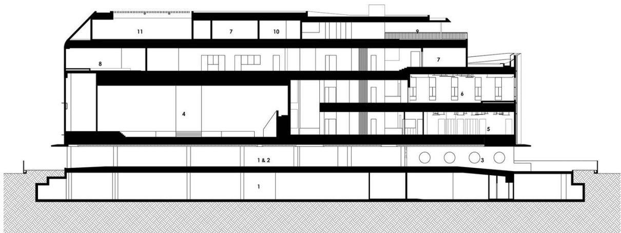
Figura 40. Corte longitudinal iglesia en Singapur Tomada de Plataforma de Arquitectura.
