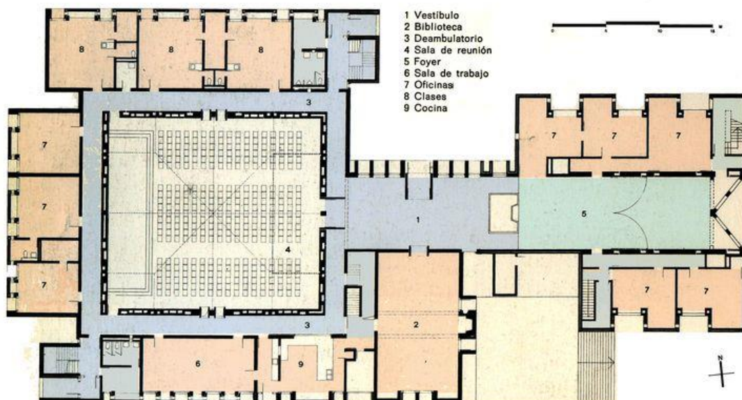
Figura 64. Planta baja iglesia en Rochester. Tomada de CoisasdaArquitectura.wordpress
