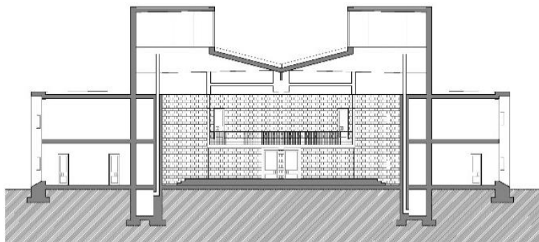
Figura 71. Corte B-B, iglesia en Rochester Tomada de Urbipedia.org, editada por el autor.
