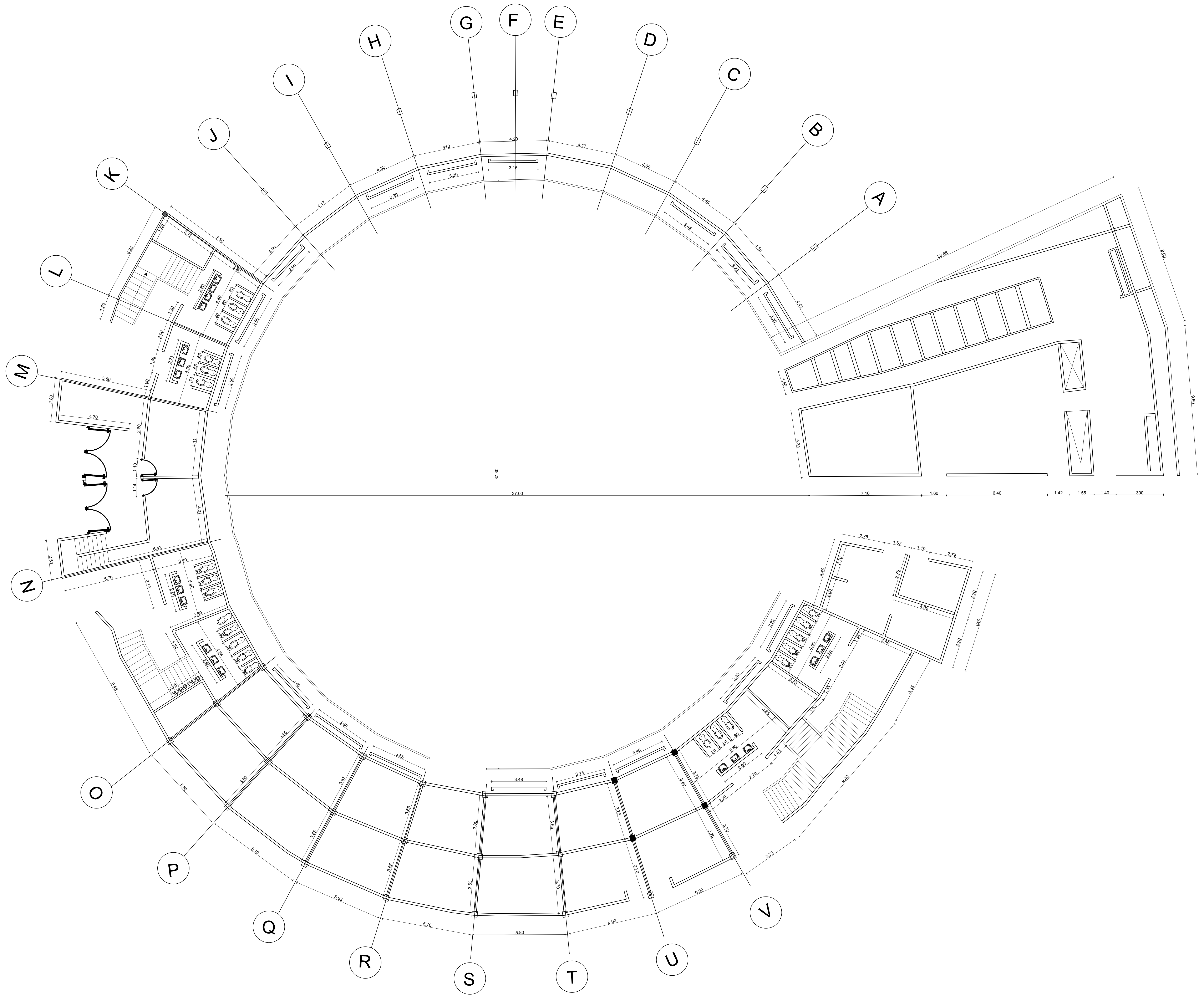
PLANTA ARQUITECTÓNICA
