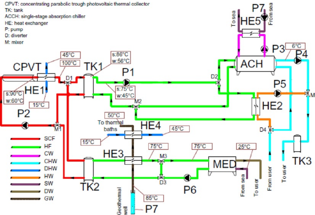
Figura 1. Diagrama de flujo de un sistema de poligeneración geotérmico. Figura tomada de [25]
