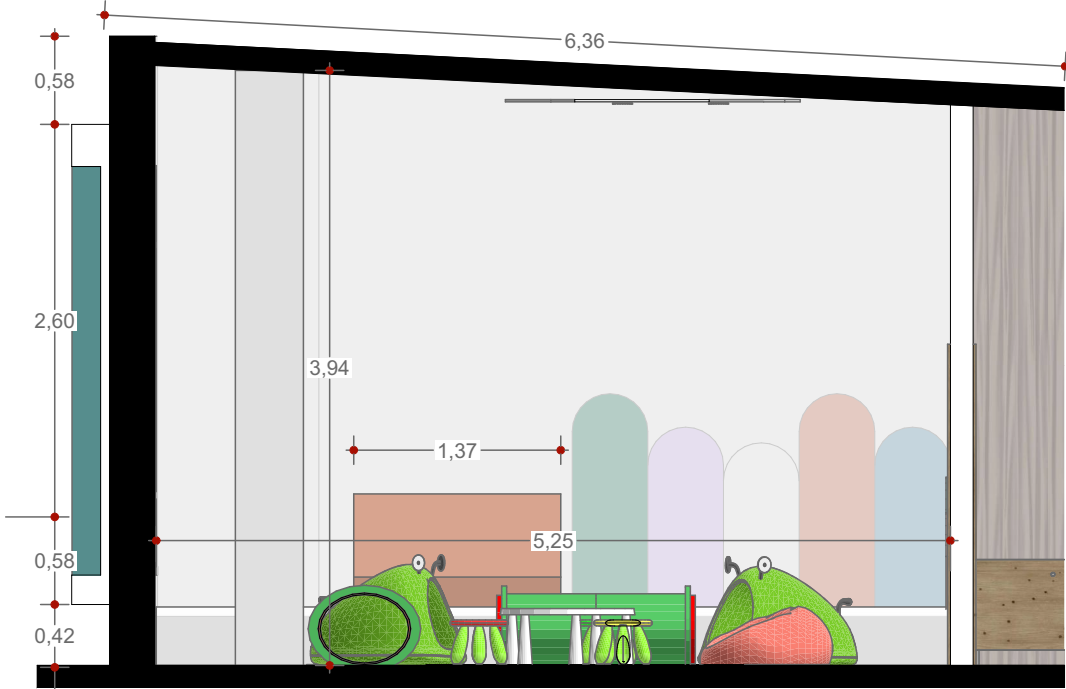
CORTE GIMNASIO Y GATEO
